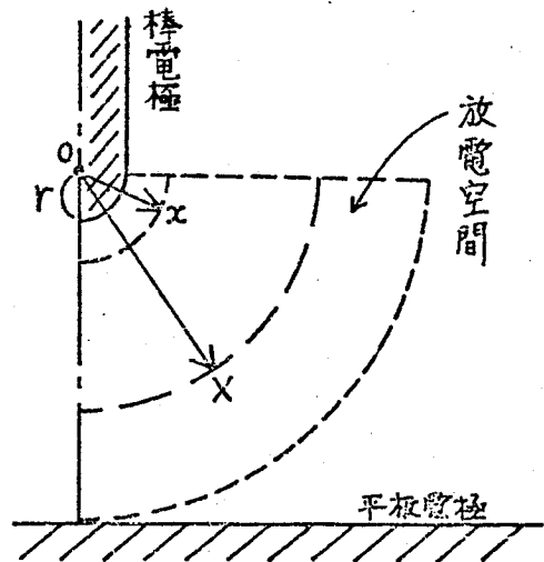
図19 放電空間の説明図
