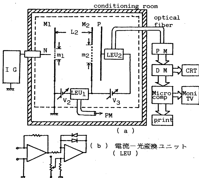
図71 実験装置
