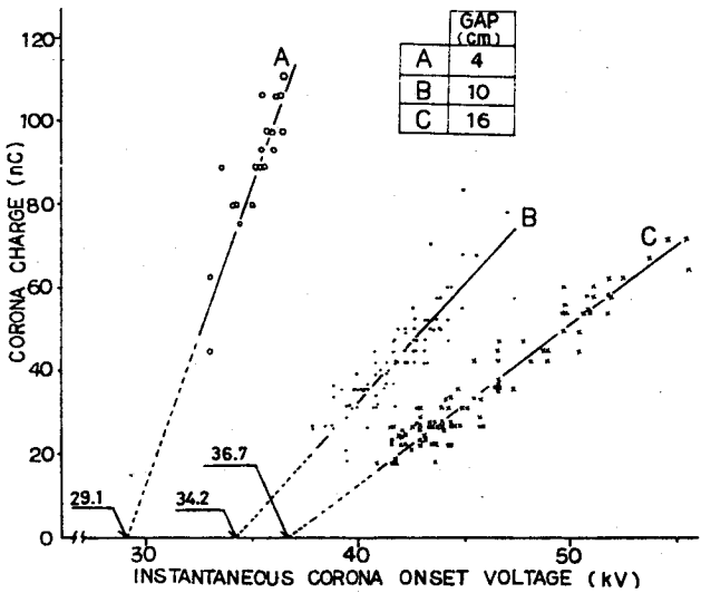
図 3 7 ファーストコロナの放電電荷量－発生瞬時電圧特性 ( V_s = 0 , 室外大気)
