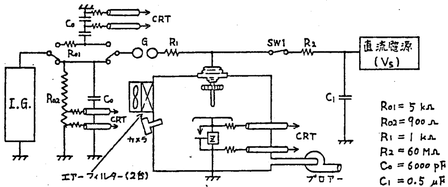
図 20 実験装置
