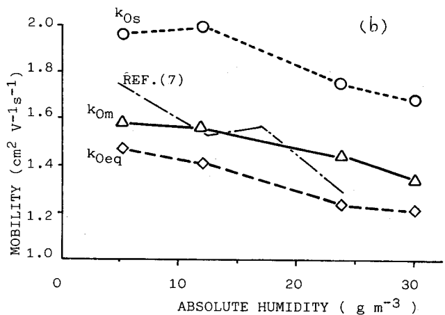
図 81 負イオン移動度に及ぼす湿度の影響 (a) 相対湿度特性, (b) 絶対湿度特性
