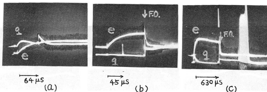
図 31 開閉インパルス印加時のオシログラム ( 4 cmギャップ , フィルタ通過大気 )
