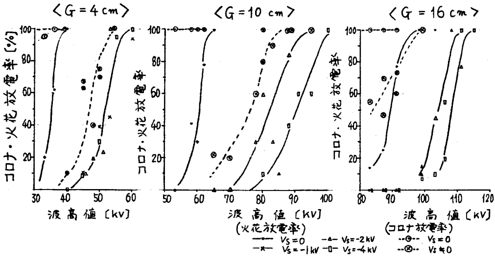
図34 コロナおよびフラッシュオーバー発生率曲線 (開閉インパルス, フィルタ通過大気) (a) 4 cmギャップ (b) 10 cmギャップ (c) 16 cmギャップ
