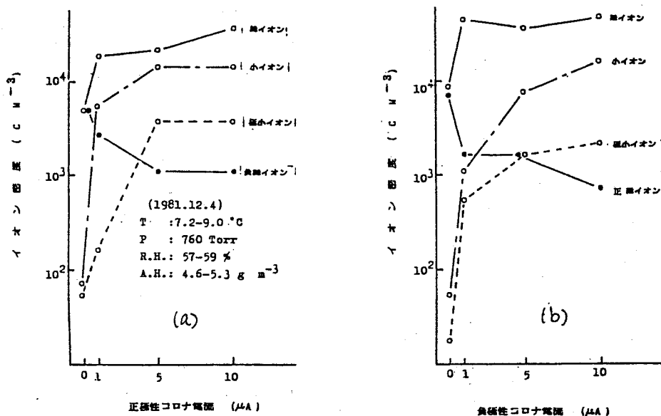
図85 直流コロナによるイオン量変化
