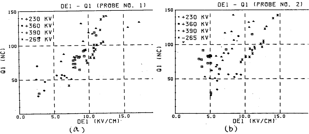
図 6 3 Q_1 - DE_1 特性 (a)プローブ 1, (b)プローブ 2
