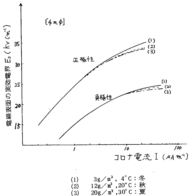
図 87 電線表面実効電界 - コロナ電流特性 (4 m φ)
