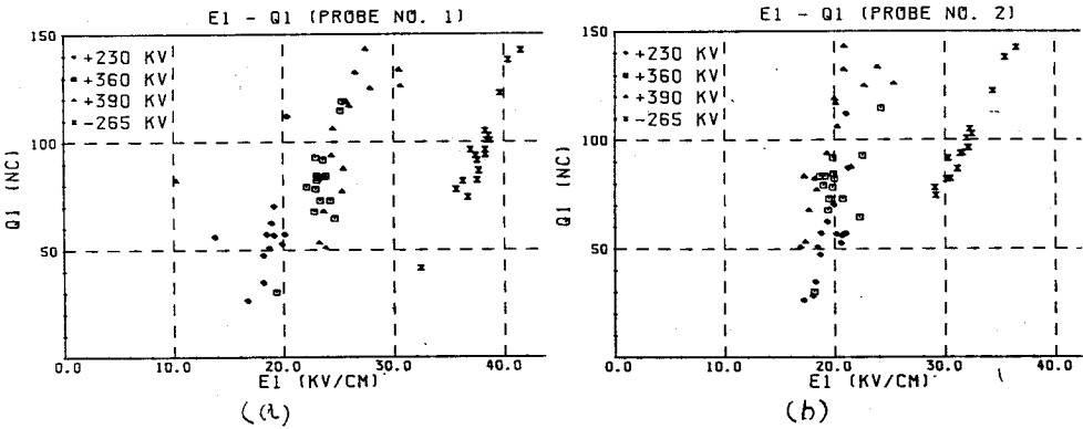
図 6 2 Q_1 - E_1 特性 (a)プローブ 1, (b)プローブ 2
