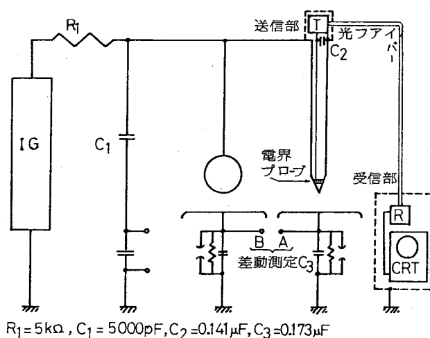
図4-1 実験装置
