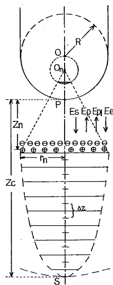
図 35 等価単一電子なだれモデル
