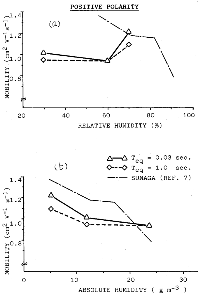
図 80 正イオン移動度に及ぼす湿度の影響 (a) 相対湿度特性, (b) 絶対湿度特性
