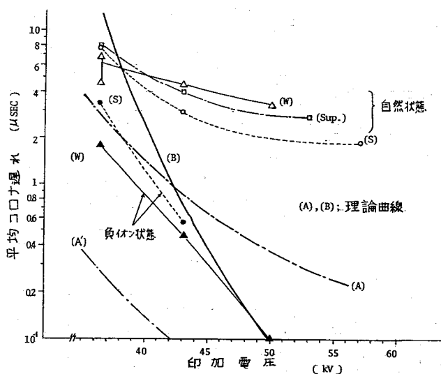
図 4 平均コロナ遅れ－印加電圧特性
