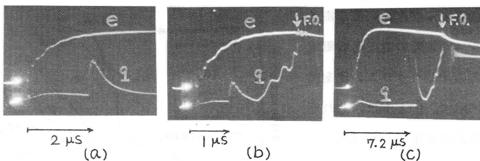
図 30 雷インパルス印加時のオシログラム ( 16 cmギャップ , フィルタ通過大気 )
