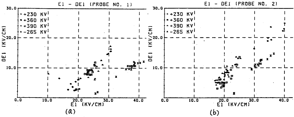
図 6 4 DE1-E1 特性
