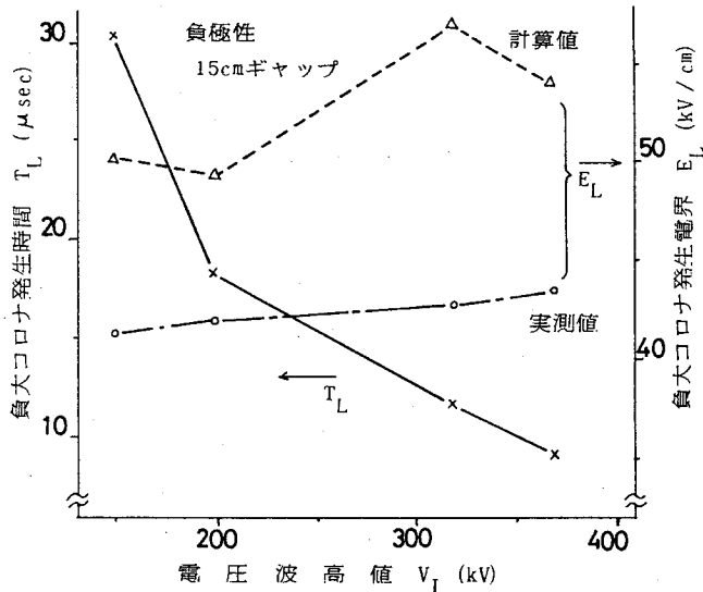
図 50 負極性大コロナの発生時間と発生電界
