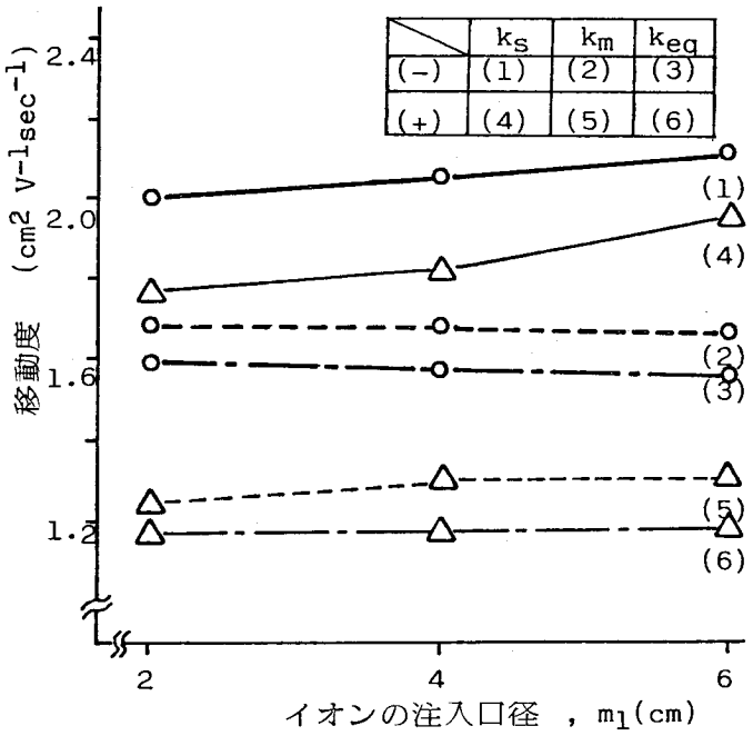
図74 イオン移動度に及ぼす口径 m_1 の影響
