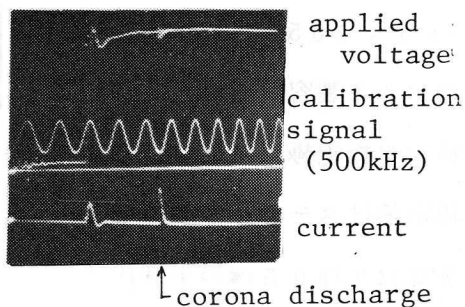
図2 電圧と電流のオシログラム
