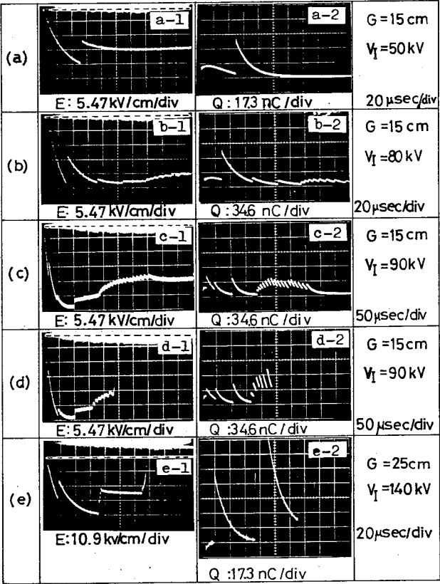
図 4 3 プローブ電界と放電電荷の オシログラム (正極性)
