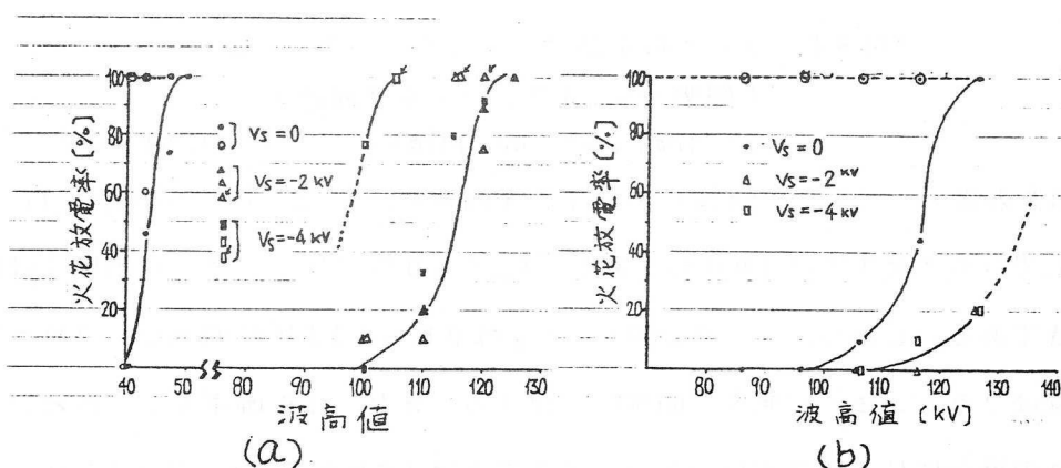
図 3 3 コロナおよびフラッシュオーバー発生率曲線 ( 雷インパルス, フィルタ通過大気 ) (a) 4 cm ギャップ (b) 16 cm ギャップ
