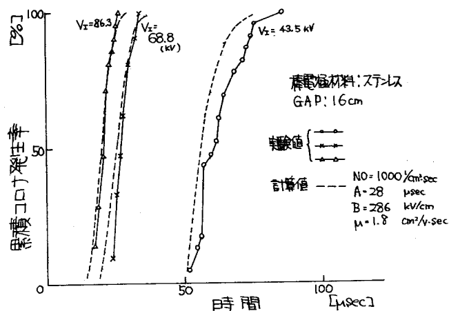
図 27 開閉インパルス印加時のファーストコロナ発生時間分布 ( V_s = 0 , 室外大気)
