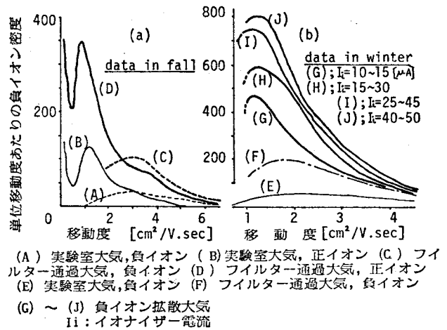
図10 各種大気の小イオン移動度分布 (a) 自然大気とフィルタ通過大気 (b) 負イオン拡散大気
