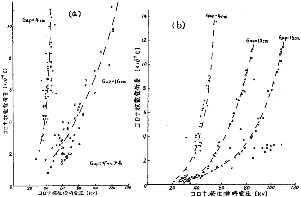
図 23 ファーストコロナの放電電荷量－発生瞬時電圧特性（フィルタ通過大気） (a)雷インパルス (b)開閉インパルス
