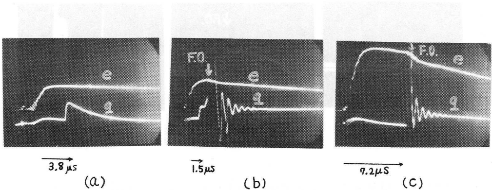
図29 雷インパルス印加時のオシログラム (4 cmギャップ, フィルタ通過大気) (a) V_I = 40 kV, V_S = 0 (b) V_I = 50 kV, V_S = 0 (c) V_I = 120 kV, V_S = -2 kV
