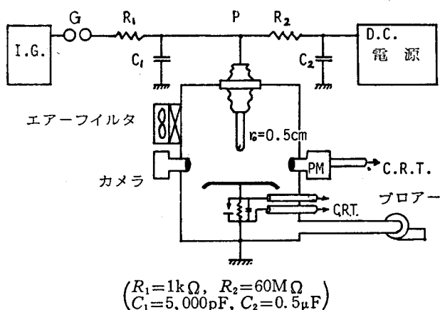
図9 実験装置
