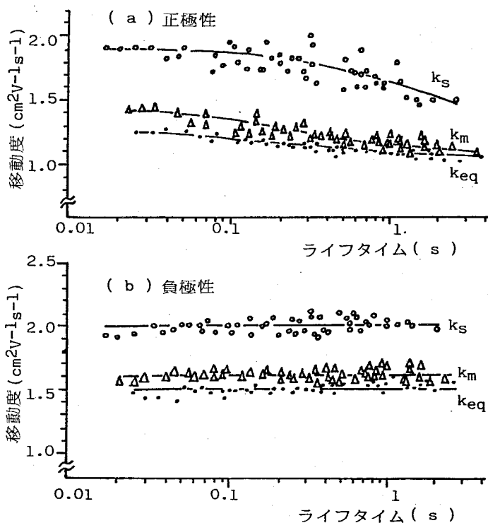
図78 イオン移動度の経時変化 ( 6^\circ\text{C} , 70\%\text{RH} , 5.1\text{ g/m}^3 )
