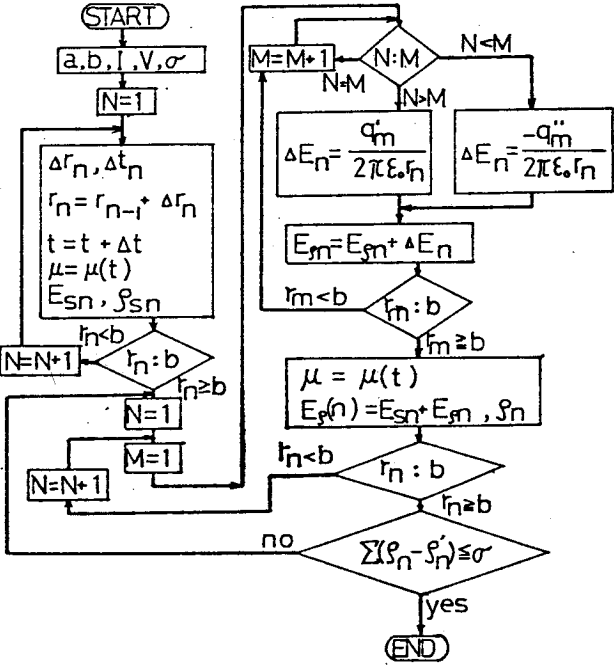
図 83 空間電荷に関する計算フローチャート
