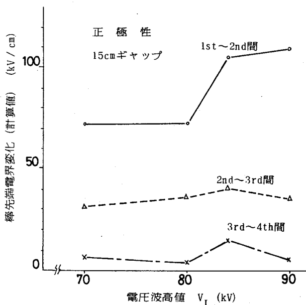
図 5.6 コロナ休止期間の棒先端電界変化（正極性，計算値）
