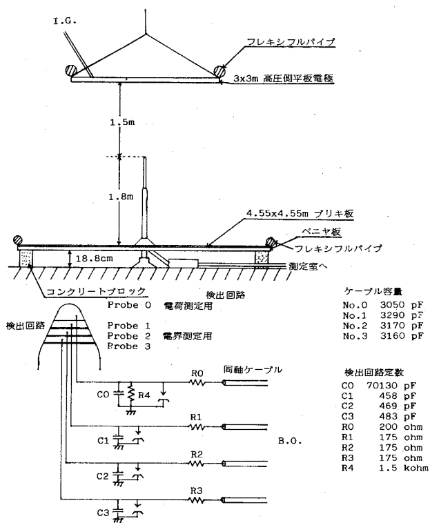
図57 実験装置
