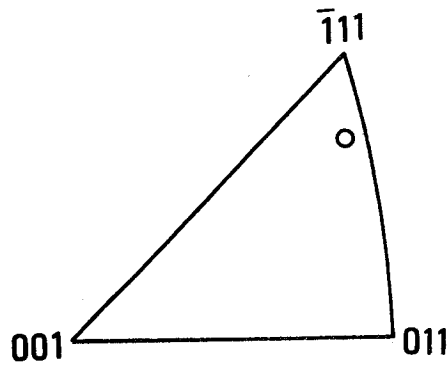
第6-1図：単結晶試料I, IIの圧縮軸方位。
