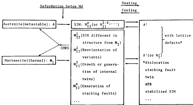
第 9-7 図：R S M 効果の機構の概念図。
