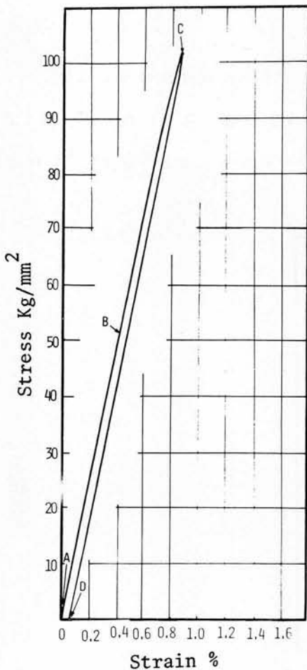
第6-6図：試料Iの応力-歪曲線図（ 40^{\circ}\text{C} ）
