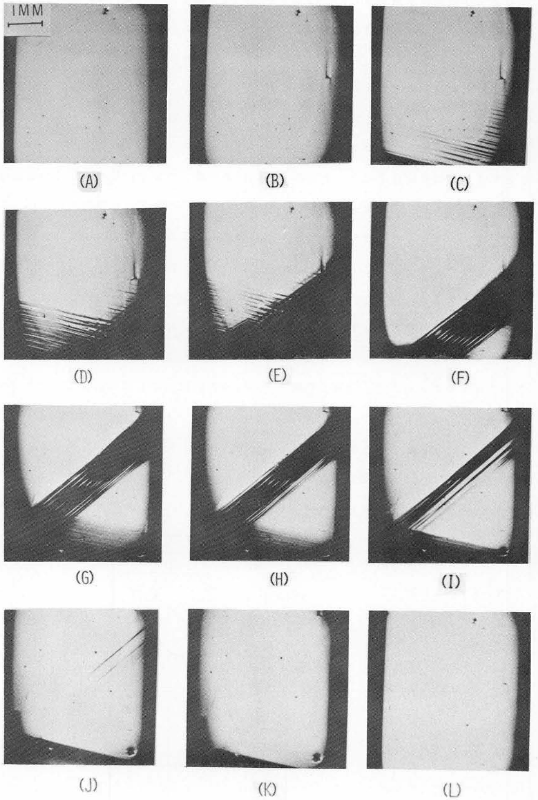
第 6-5 図： 6-4 図に対応する表面組織の変化。A-L は 6-4 図の各点に対応。
