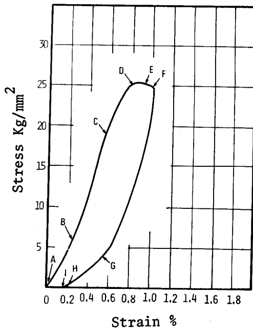
第 6-13 図：試料Ⅱの応力-歪曲線図（160℃）
