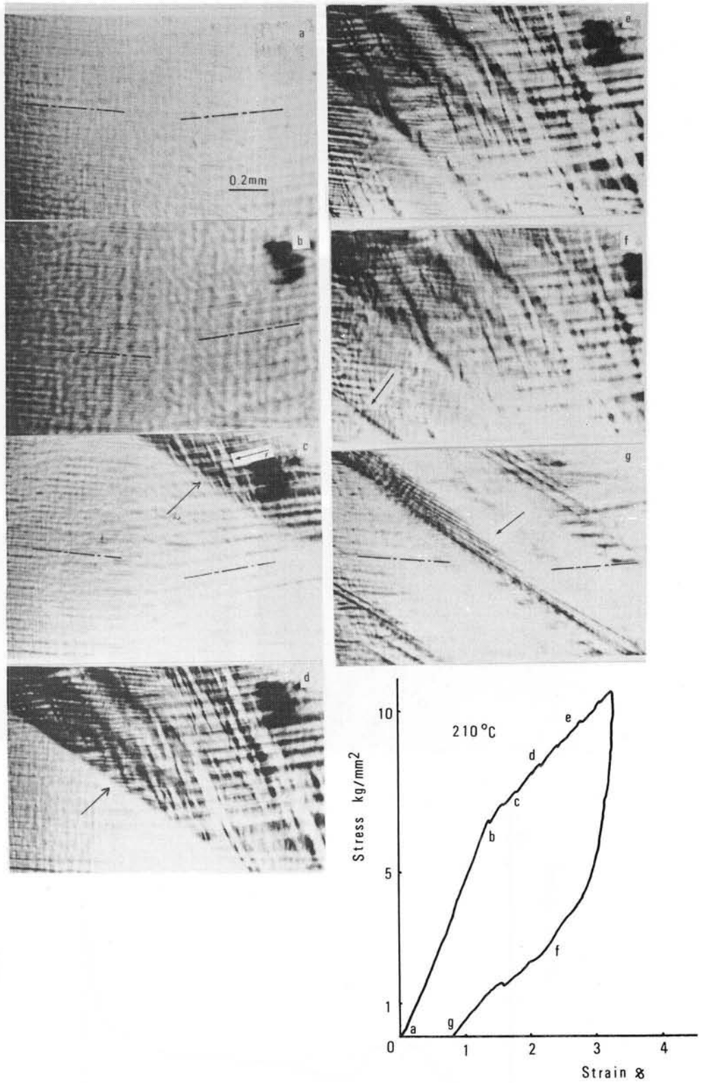
第 5 - 8 図 : 同じく 210°C における変形による表面組織の変化。
