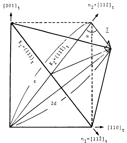
第 2-24 図: \{111\}_t \langle 112 \rangle_t 双晶の各要素。ここでは c/a \approx 0.86 として図示。紙図は (1\bar{1}0)_t 面。
