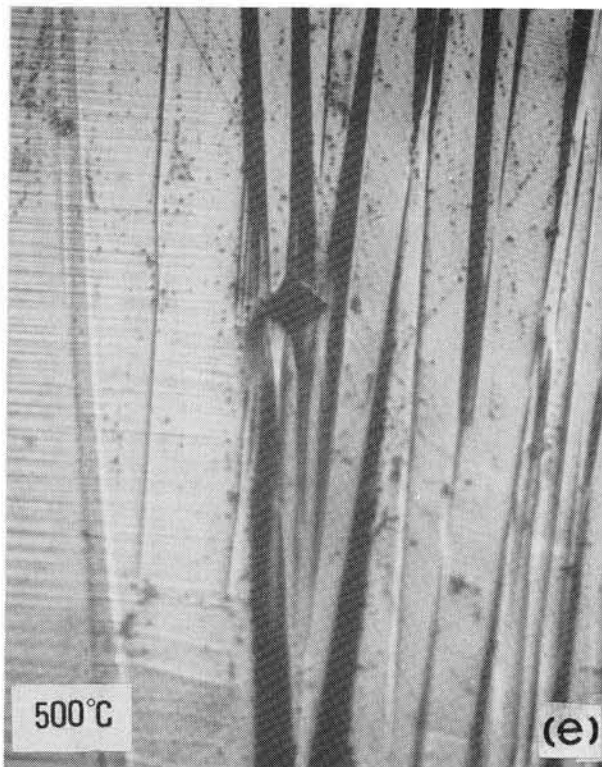
第5-2図(a)~(d): 63.8Ni-1Co-Al マルテンサイトの形状記憶効果に伴う試料表面組織の変化(説明は本文)。
