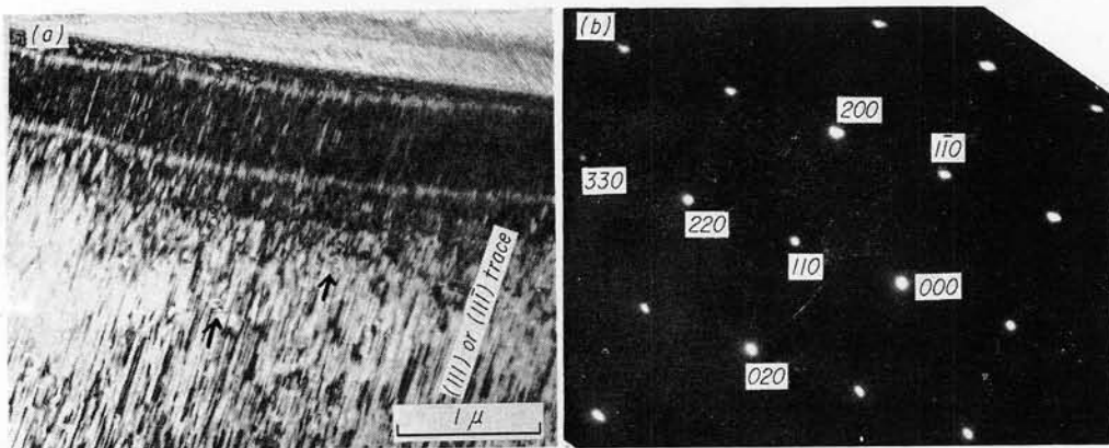
第2-14図：63.8Ni-1Co-Al (合金A) マルテンサイトの透過電顕写真、(a)多数の面欠陥は積層欠陥と考えられる。
