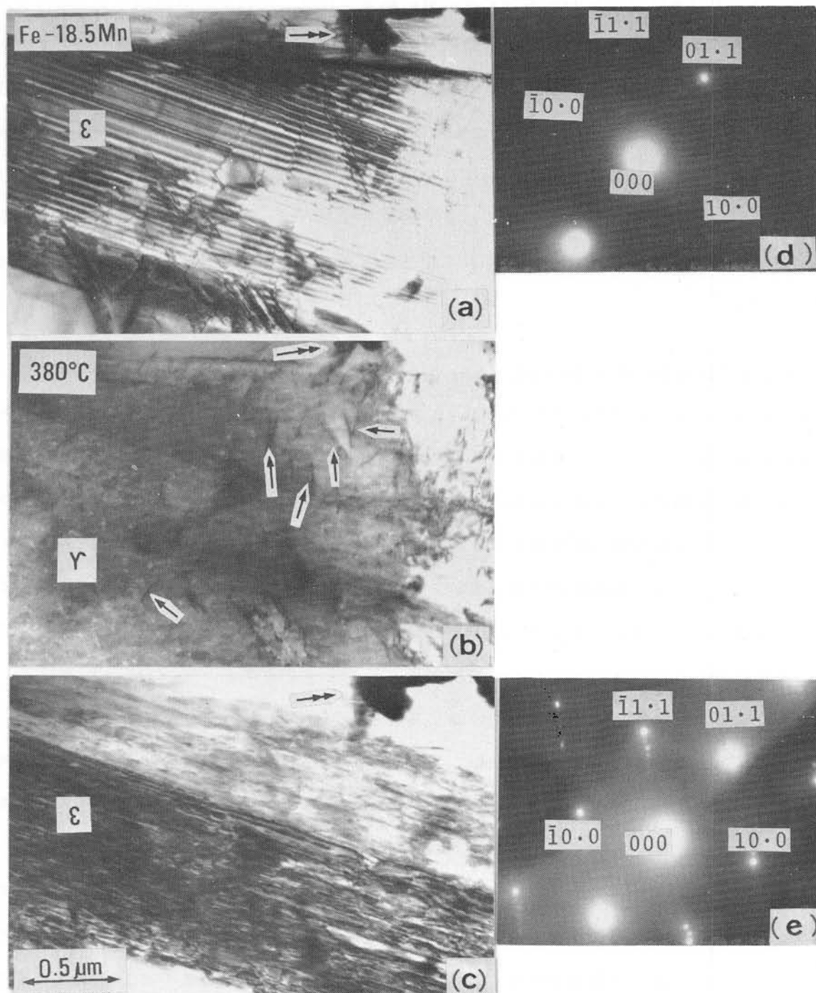
第9-6図：Fe-18.5Mn合金のRSM効果に伴う組織変化の電子顕微鏡観察。
