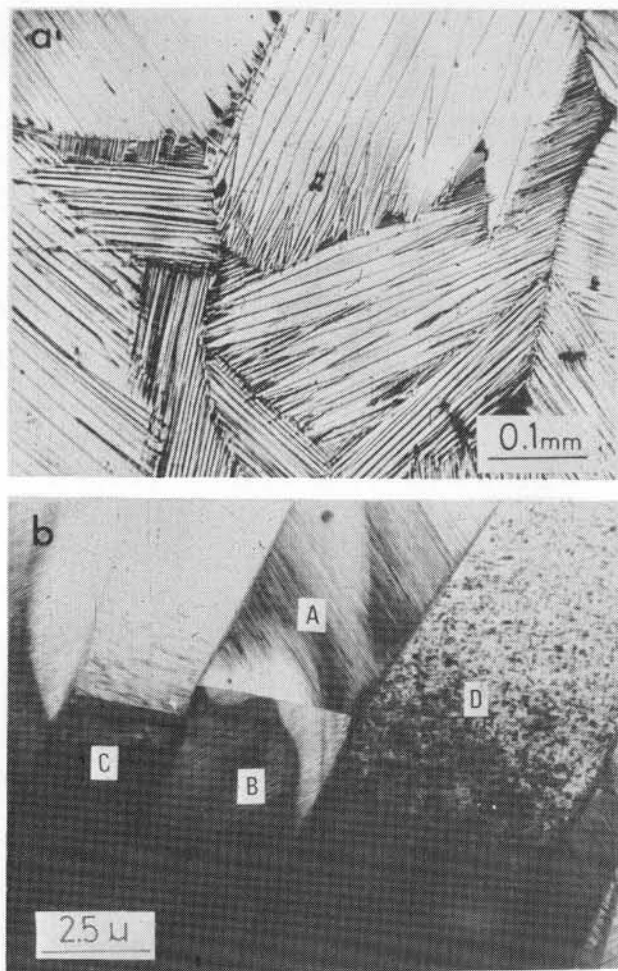
第2-18図：水焼入れした合金Aのマルテンサイトの光学顕微鏡写真(a)及び電子顕微鏡写真(b)。
