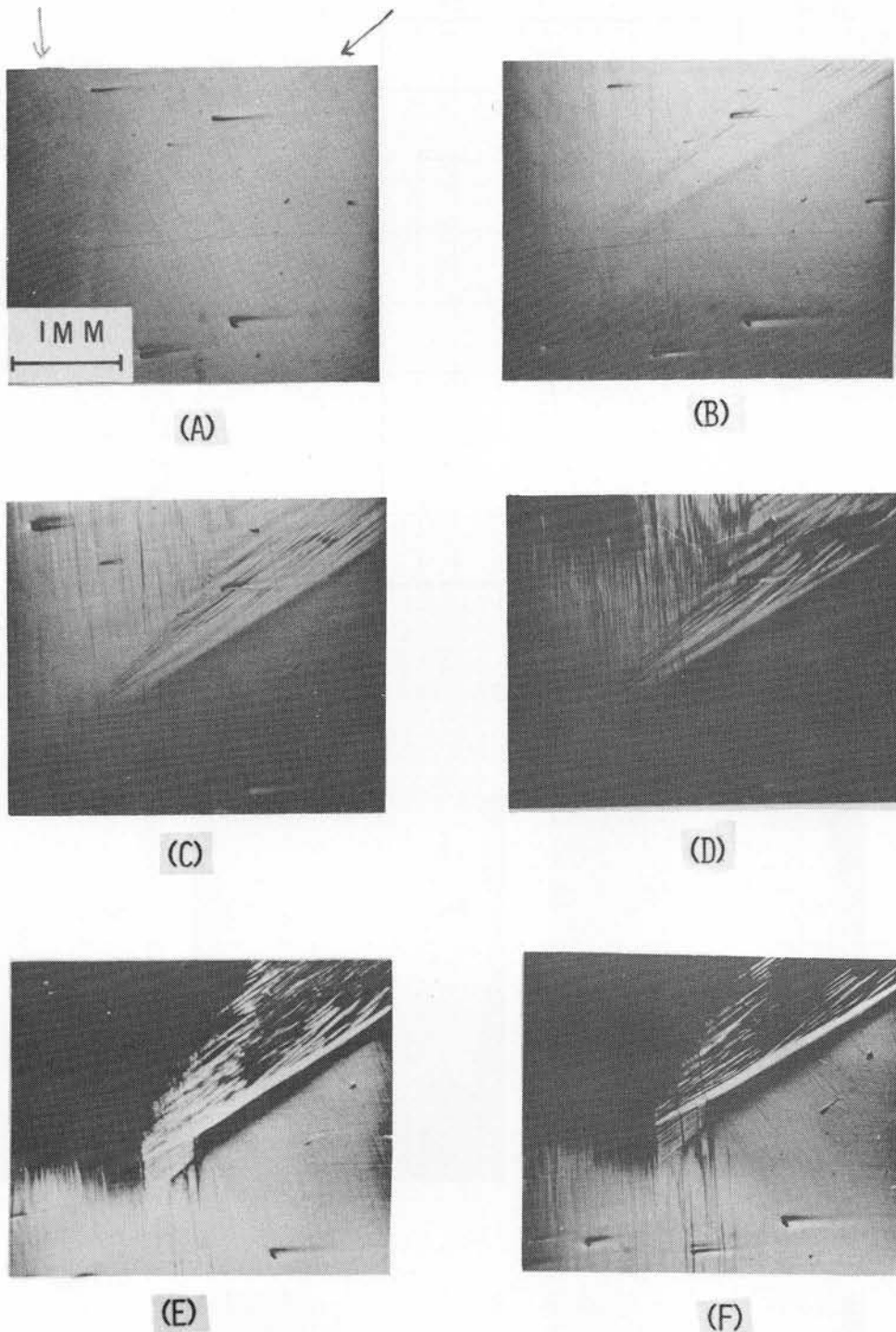
第6-9図：6-8図に対応する表面組織変化。A-Fは6-8図各点に対応。
