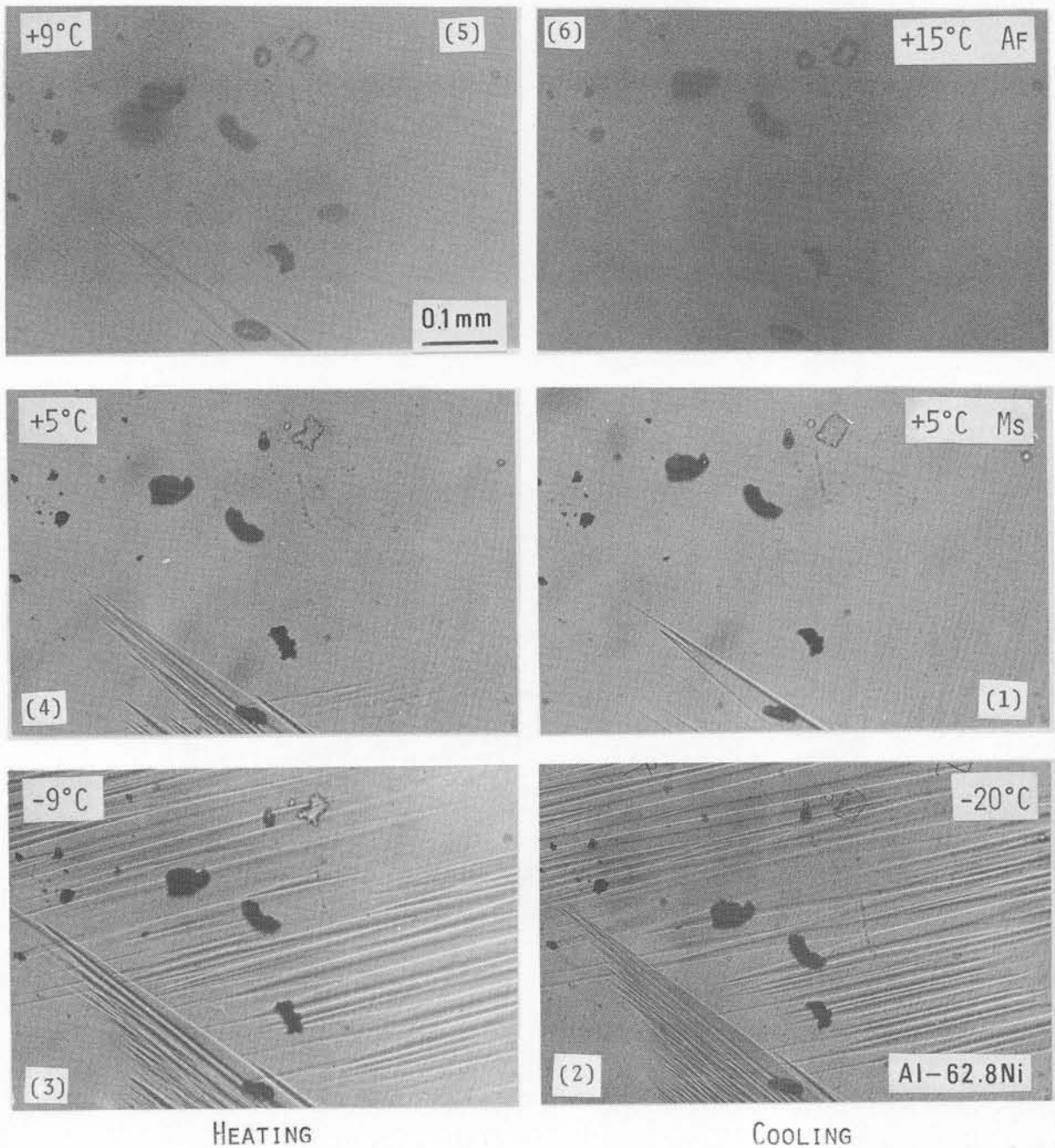
第 2-12 図： 62.8 Ni-Al 合金（合金 B）のマルテンサイト変態、逆変態に伴う表面起伏の変化、（1～6 は同一視野）。
