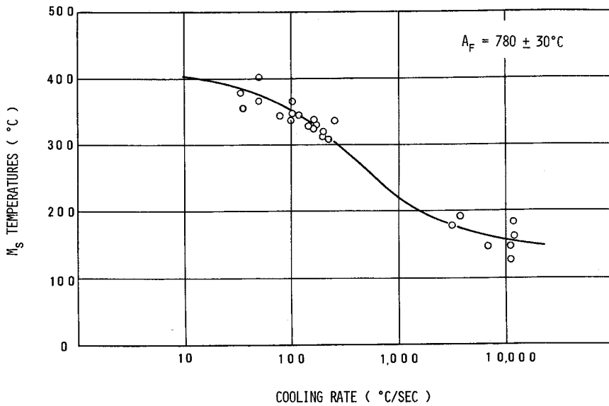
第2-9図：63.8 Ni-1 Co-Al 合金の Ms 点の冷却速度依存性
