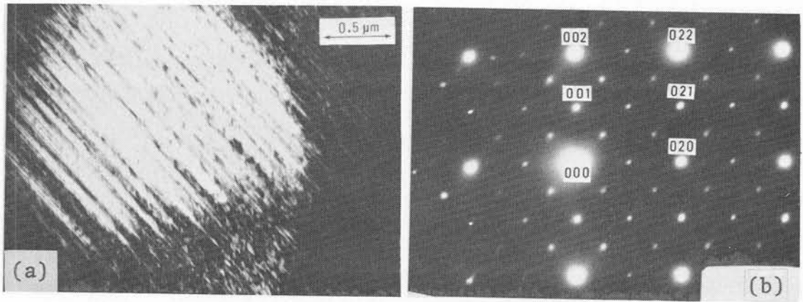
第3-5図：300℃×30分時効後の焼戻しマルテンサイトの電顕写真、(a)透過電顕写真。(b)制限視野回折写真。 この指数は、もとのマルテンサイトの結晶構造(L1 0 )のものを付してある。
