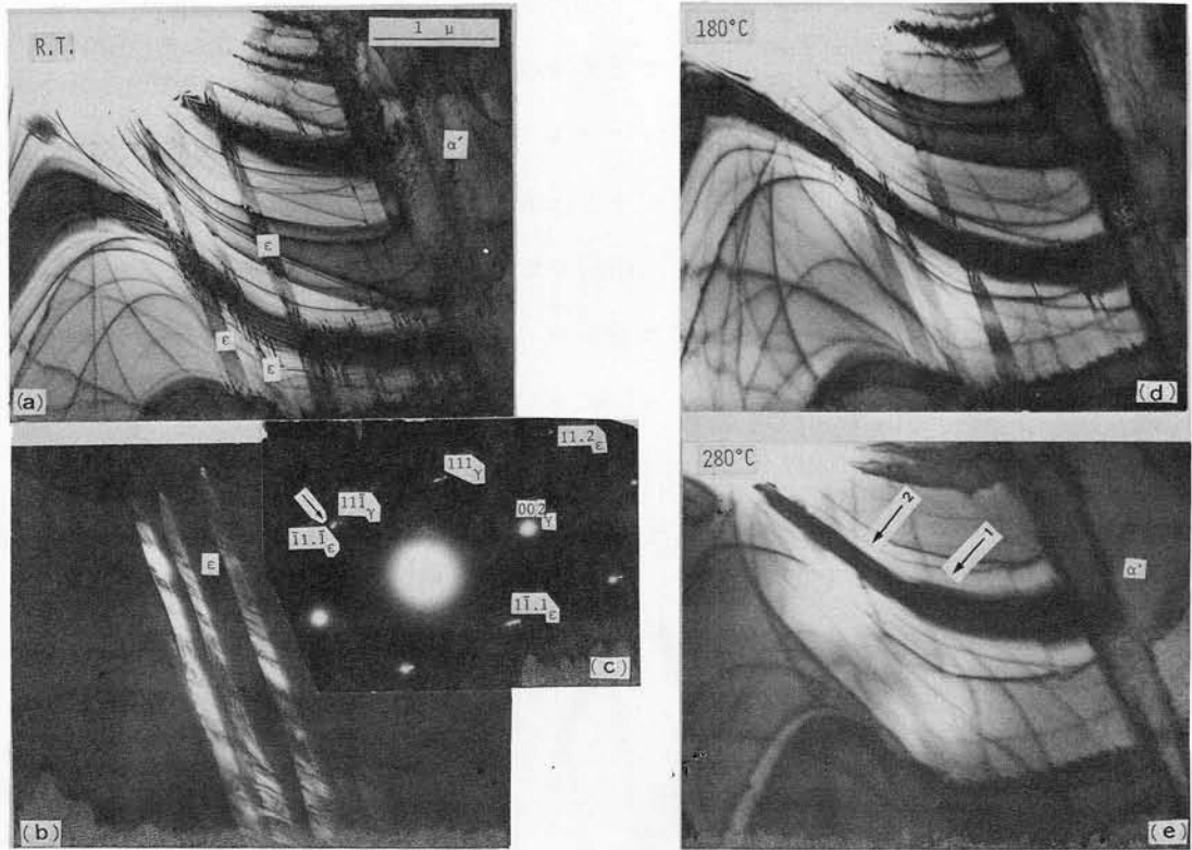
第7-6図：加熱による \epsilon 相の変化。(a)透過電顕写真(室温)。 \epsilon 相に注意。(b) 111_{\gamma} \cdot \bar{1}\bar{1}\bar{1}_{\epsilon} 斑点による暗視野像、 \epsilon 相が反転していることにより、(a)の \epsilon と記したすじが \epsilon 相であることがわかる。(c)制限視野回折写真。 \gamma 相に加え \epsilon 相の回折斑点が存在する。(d)180°C、 \epsilon 相は徐々に消滅しはじめる。(e)280°C、 \epsilon 相は殆んど消滅したのがわかる(矢印1)。いずれの写真も \alpha' 相は変化がない
