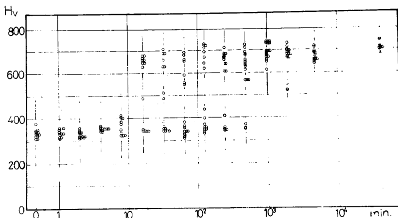
第3-1図(a): 63.8 Ni-1 Co-Al合金マルテンサイトの時効に伴う硬度(VHN)の変化。
