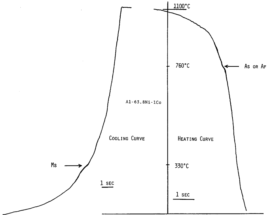
第2-8図：63.8 Ni-1 Co-Al 合金の冷却・加熱に伴う Thermal arrest.
