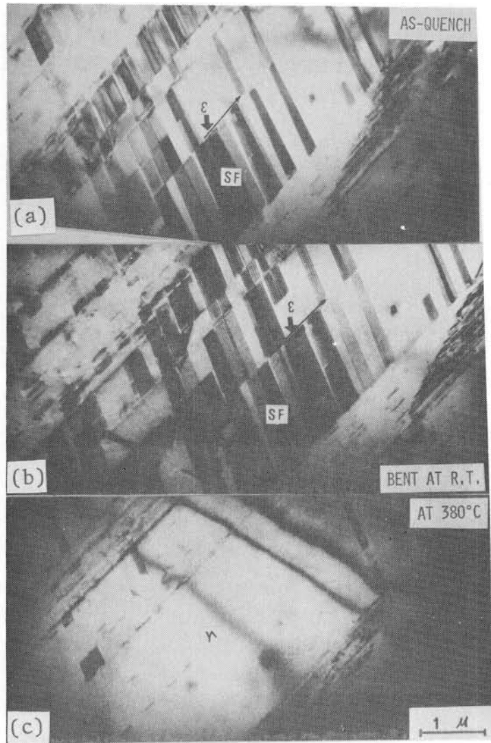
第 8 - 5 図: Fe-18.5 Mn 合金の透過電子顕微鏡写真。
