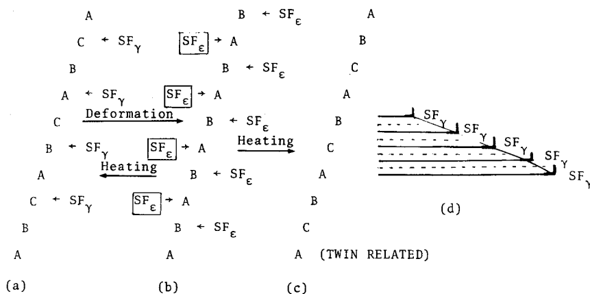
第8-9図: \gamma \leftrightarrow \epsilon 変態の機構
