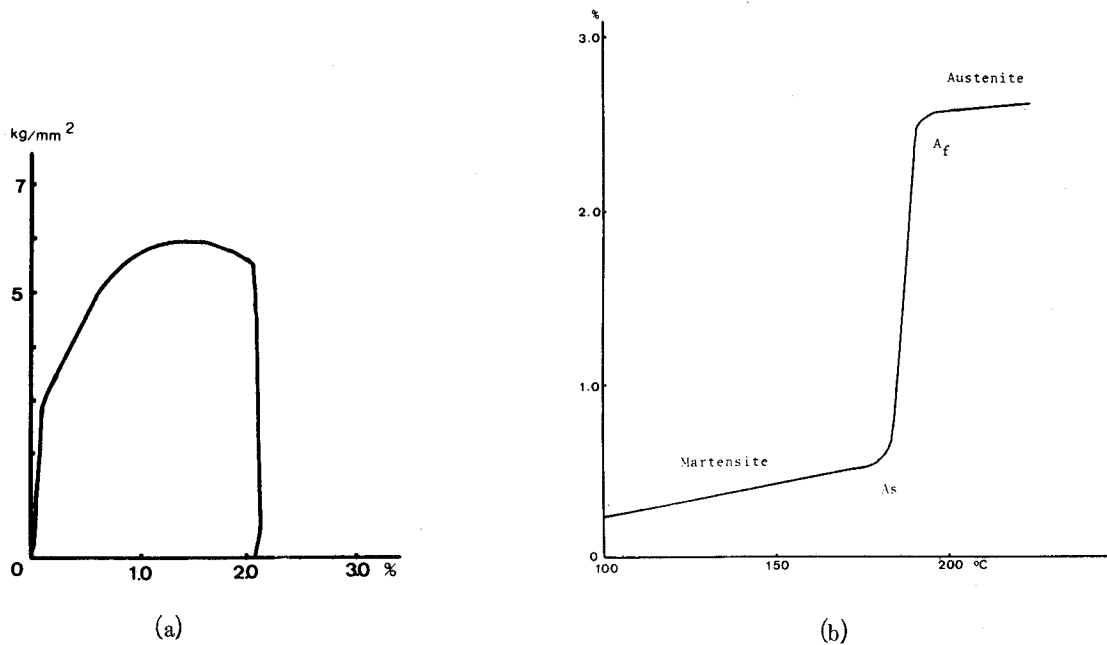
第6-17図 (a): 64.0 Ni-Al マルテンサイトの応力-歪線図(室温)。
