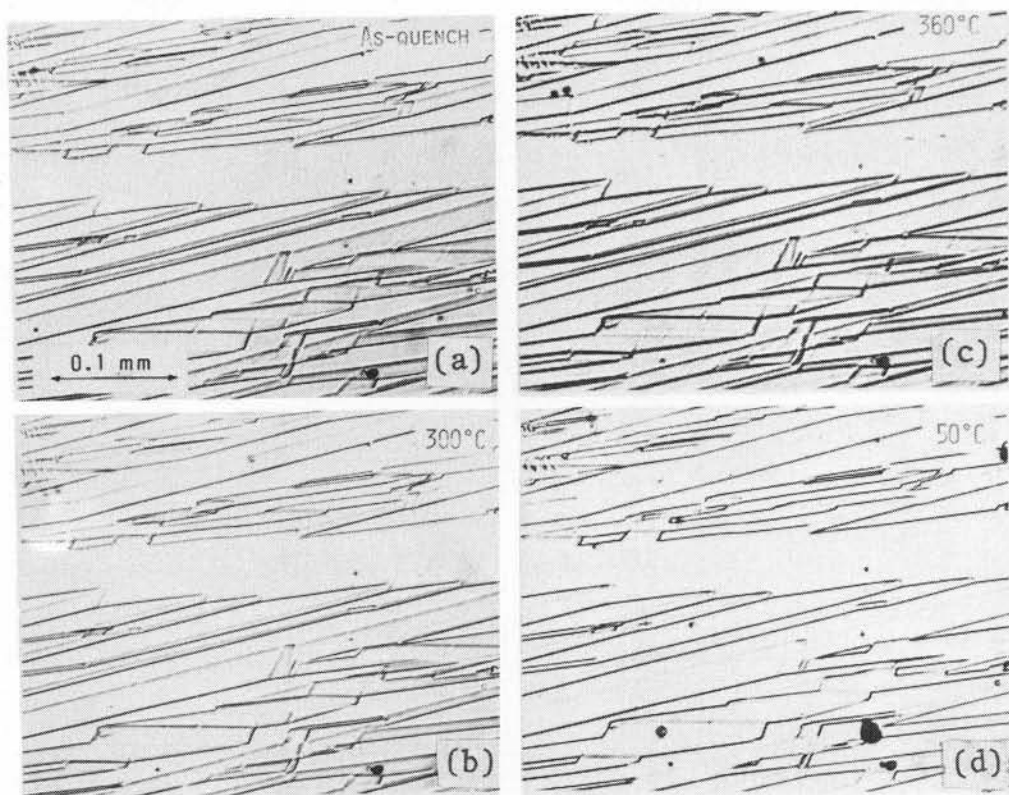
第2-10 図：63.8 Ni-1Co-Al 合金マルテンサイトの加熱に伴う表面組織の観察。写真はすべて同一視野である。
