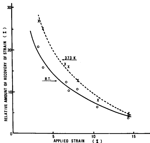
第7-2図：18-8ステンレス鋼における形状記憶効果。
