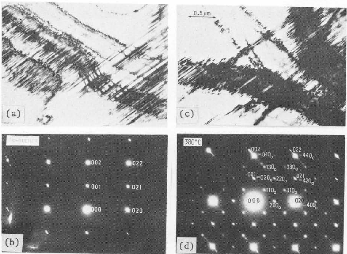
第3-8図: 電顕内加熱による結晶構造変化を示す電顕写真。
