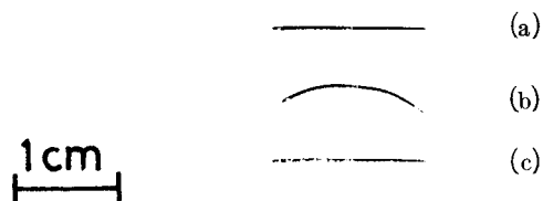
第5-1図：63.8Ni-1Co-1Al マルテンサイトの形状記憶効果。
