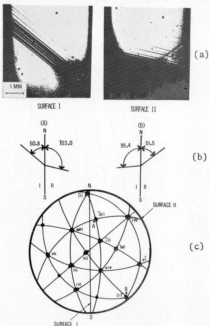
第 6-16 図：試料 I の応力誘起マルテンサイトの晶癖面の決定。
