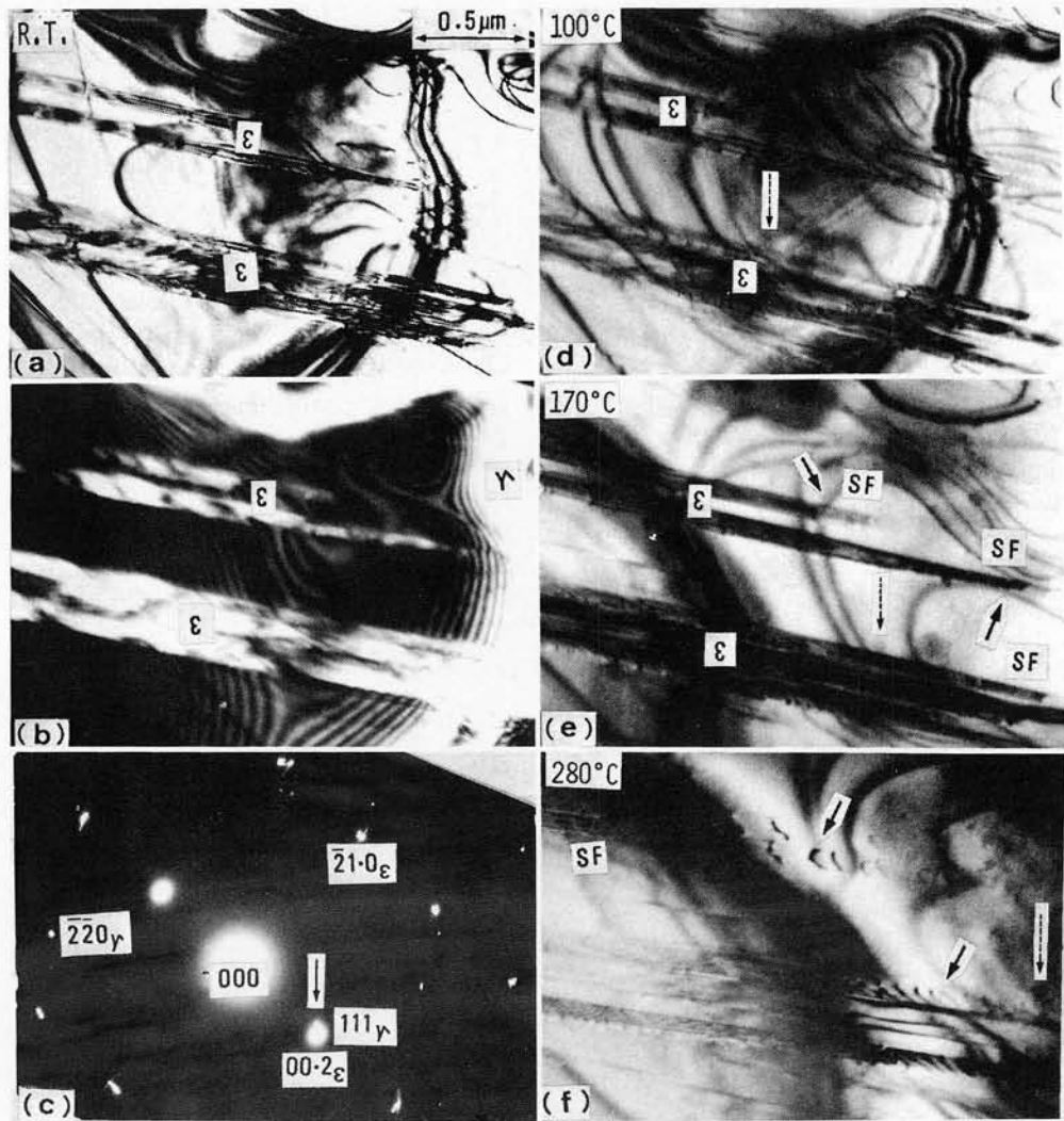
第7-8図：加熱に伴う \epsilon 相の変化。
