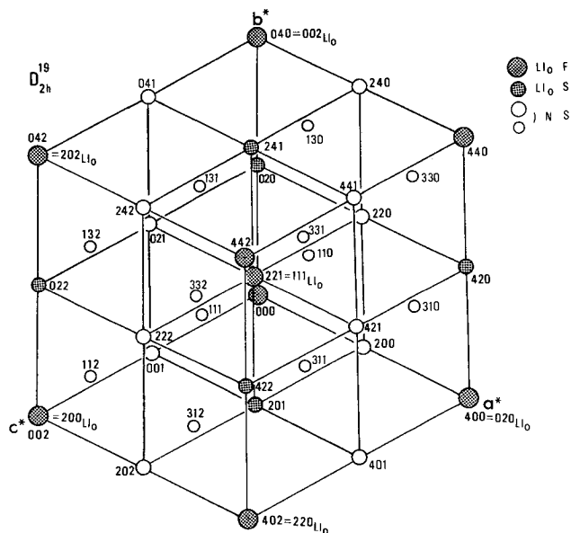
第 3-16 図： 3-15 図を考慮して入れて構成した逆格子。 D_{2h}^{19} に相当する。
