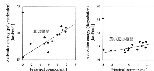
図 3 第 1 主成分と重合 (左)、熱分解 (右) 反応性との相関
