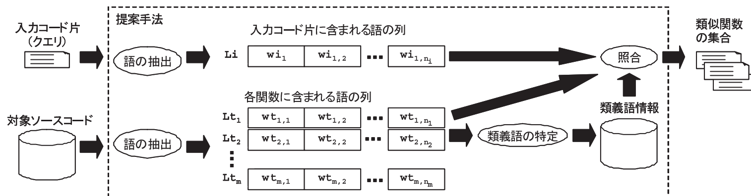
図 5 提案手法の概要
