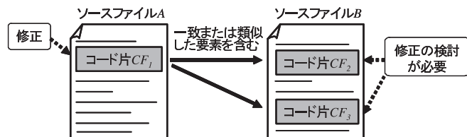
図 1 類似コード片
