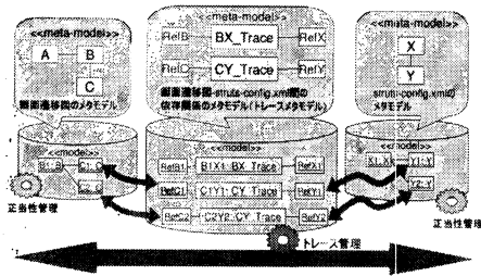
図 12: 成果物間のトレース管理
