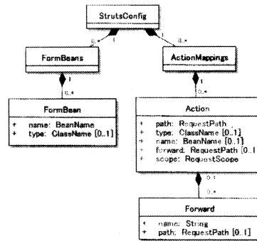
図 5: struts-config.xml の MOF メタモデル
