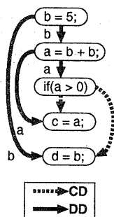
図 3: 図 2 の PDG
