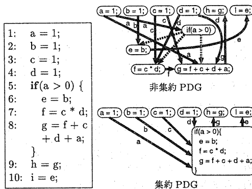
図5: 節点集約例
