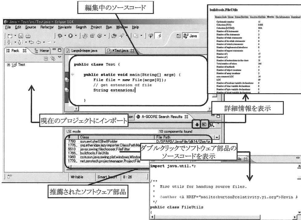
図 4 A-SCORE の画面
