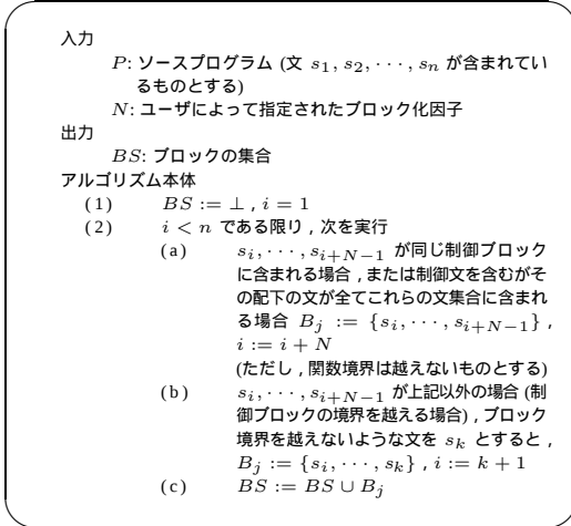
図 5 ブロック化アルゴリズム
