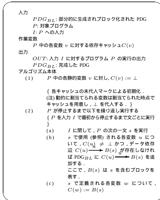
図 7 データ依存関係収集アルゴリズム
