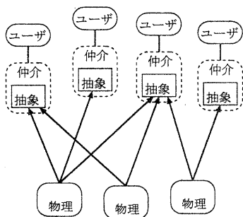
図 2: 概念的関係
