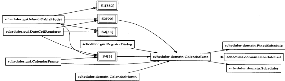
図 2: DateCell をグループ化したクラス間の呼び出し関係グラフ。 G_c(\text{DateCell}) = \{s_1, s_2, s_3, s_4\}
