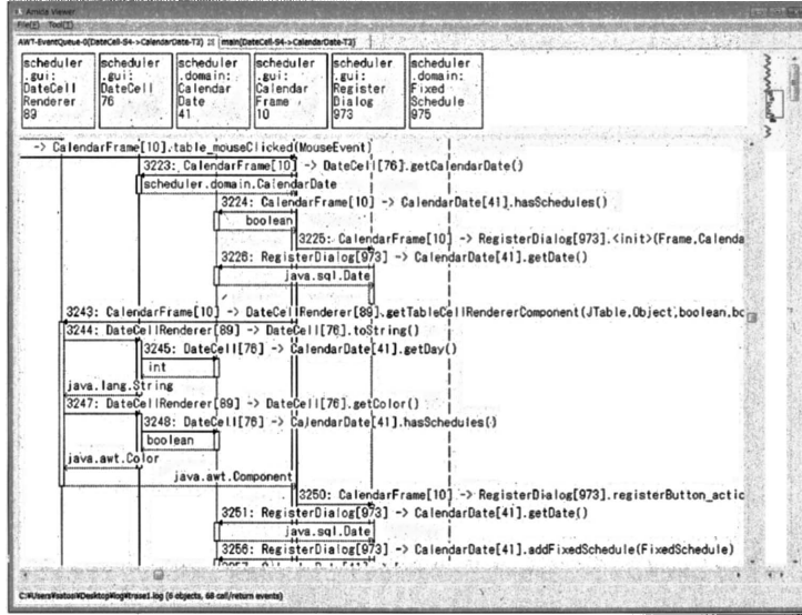
図 7: DateCell クラスのグループ s_4 と CalendarDate クラスのグループ t_3 の相互作用例を可視化したシーケンス図. ユーザのマウス操作に関するメソッド呼び出し後, DateCell から CalendarFrame を経て RegisterDialog に CalendarDate が渡されたのち, RegisterDialog により予定データが追加されている.
