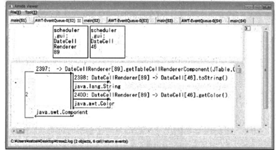
図 3: DateCell クラスのグループ s_2 に属するオブジェクトの振舞いを可視化したシーケンス図。DateCellRenderer からの描画情報の要求に応じている。
