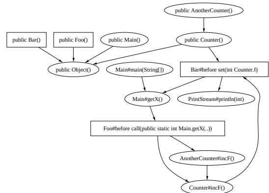
図 2 コールグラフの例 Fig. 2 A call graph.
