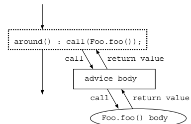
図4 メソッド呼び出し頂点における around アドバイスの呼び出し Fig.4 Around advice call at method call node.
