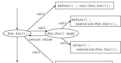
図3 メソッド呼び出し頂点におけるアドバイス呼び出し Fig.3 Before advice call and after advice call at method call node.
