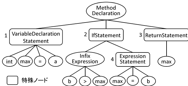
図 3 AST 中の特殊ノードへの番号付の例
