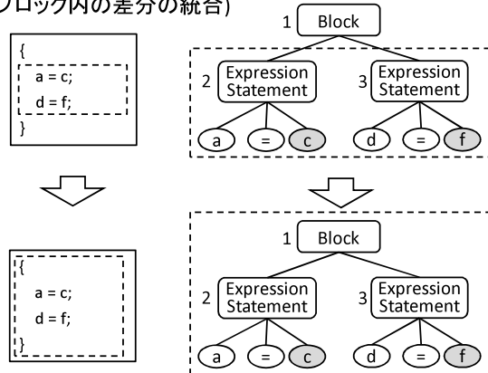
図 6 差分の統合操作
