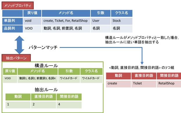
図 3 メソッドプロパティ, 抽出パターン, パターンマッチ Fig. 3 Method property, extraction pattern and pattern match.
