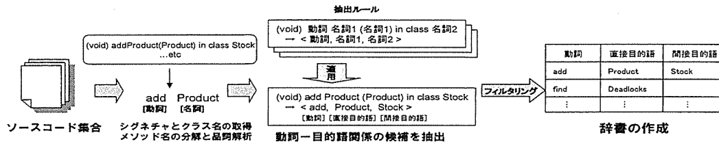
図 1 手法の概要
