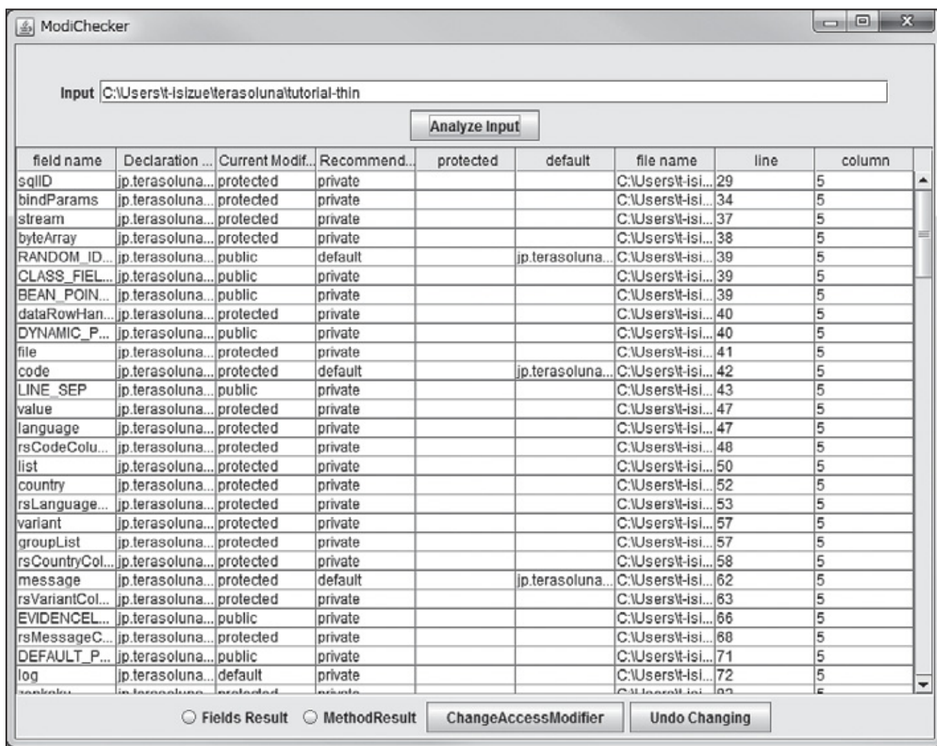
図 1 ModiChecker の AE 表示画面
