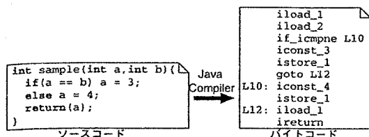
図1 バイトコードへの変換例
