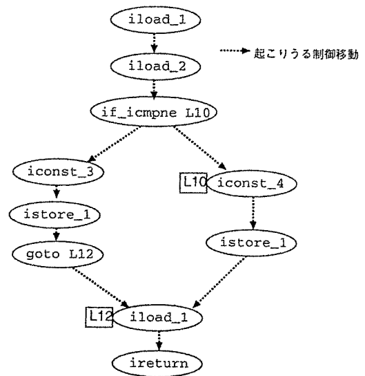
図 6 図 1 の CFG
