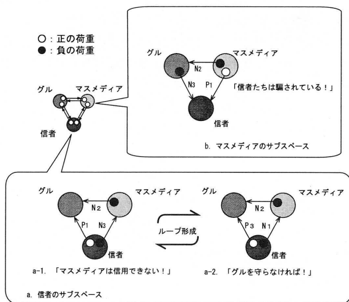
図 4.2 マスメディアのネットワーク反対効果
