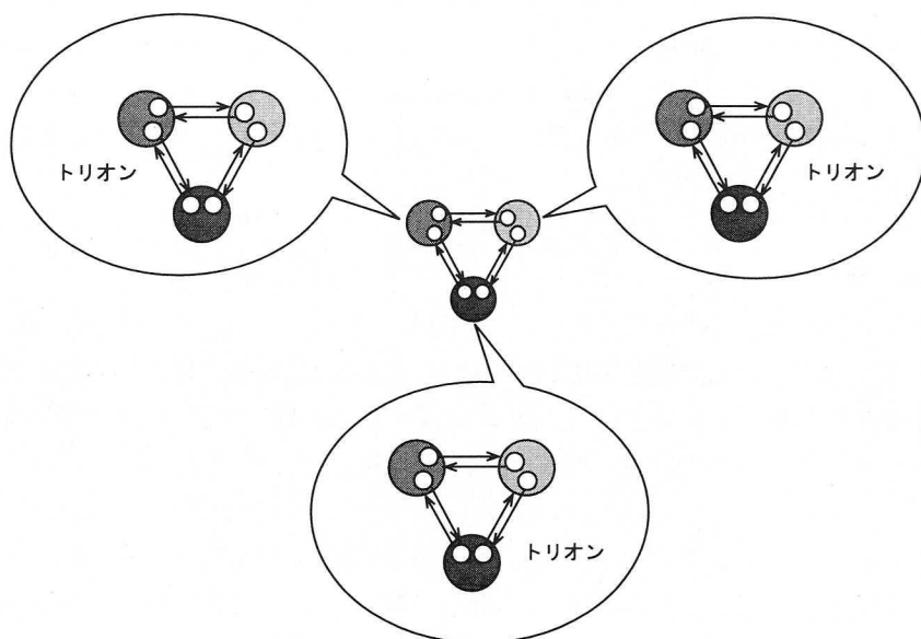
図3.1 トリオンの吹き出しモデル
