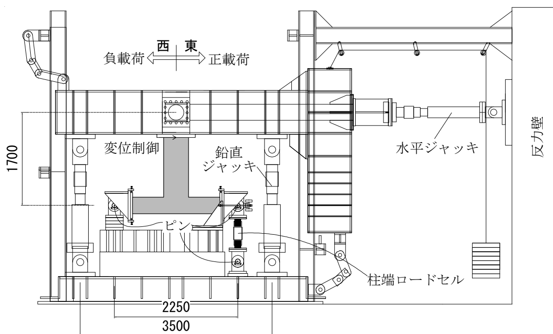
図 3.2.2 実験設置
