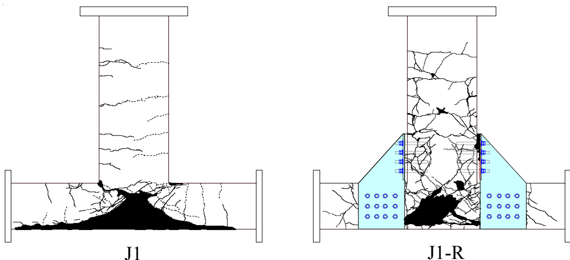
図 4.6.5 最終破壊状況の比較
