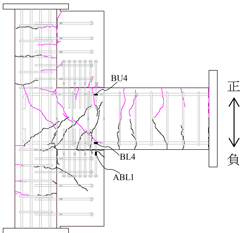
図 5.4.5 鉄筋の降伏位置および破壊状況 (1/133 サイクル載荷終了時)
