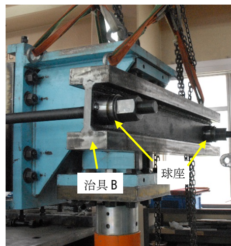
(c) 詳細写真：治具 B
