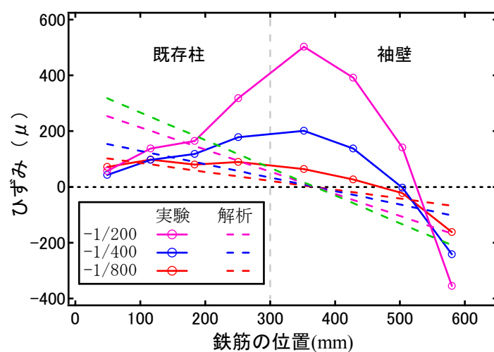
図 6.4.3 J2-W1 の袖壁付き柱の危険断面で鉄筋ひずみ度の実験値と解析値の比較
