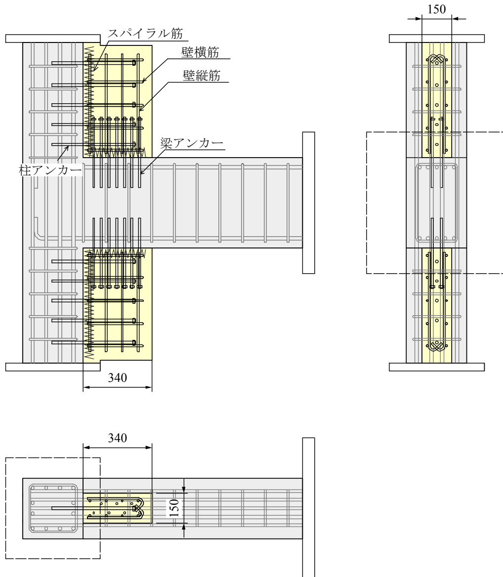
図 5.3.2 補強試験体の形状
