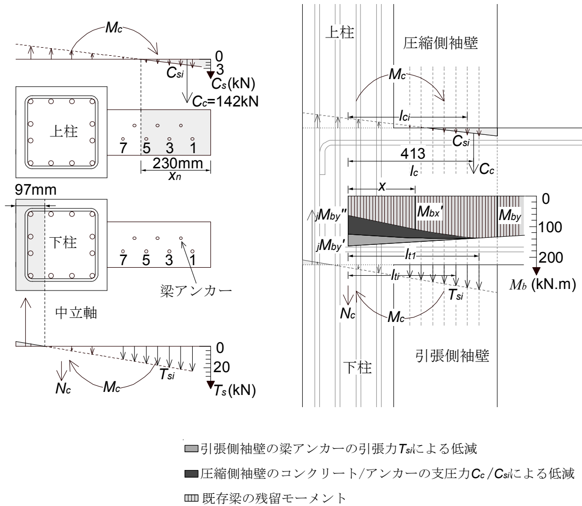
(a) 袖壁付きの上/下柱の曲げ解析結果 (b) 既存梁のモーメント分布
