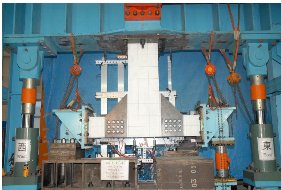
写真 4.5.1 試験体設置の様子
