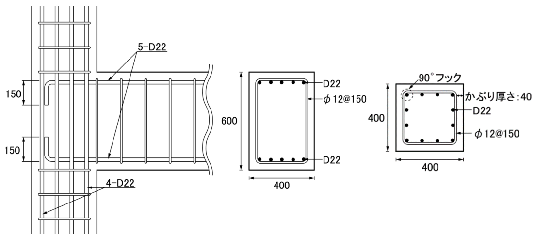
図 1.2.2 研究対象建物の外柱梁接合部の構造詳細 15)
