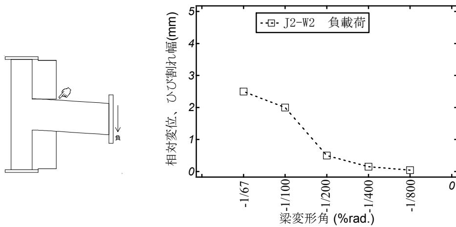
(b) 連層補強試験体の負荷荷時
