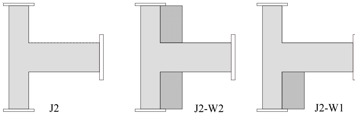
図 5.3.1 袖壁補強の検証実験用の試験体
