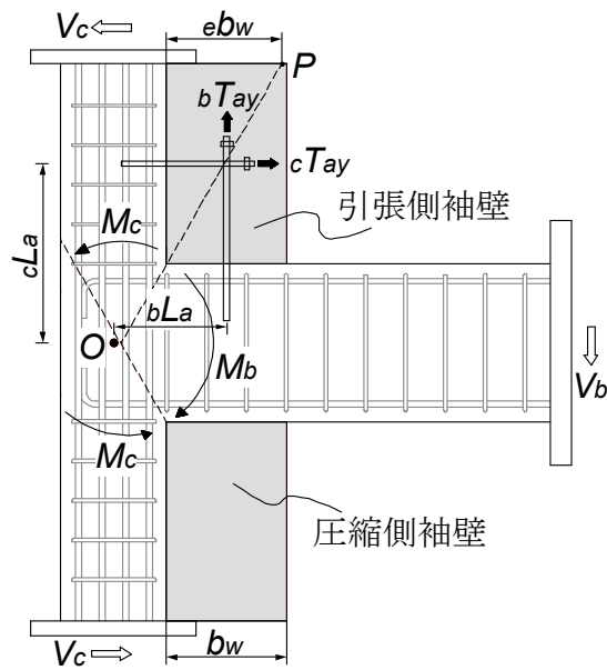
図 5.2.1 袖壁補強の概念
