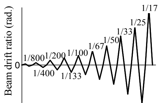
図 5.3.7 载荷プログラム
