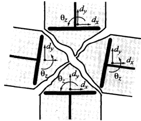
図 1.5.2 9 自由度モデル 25)
