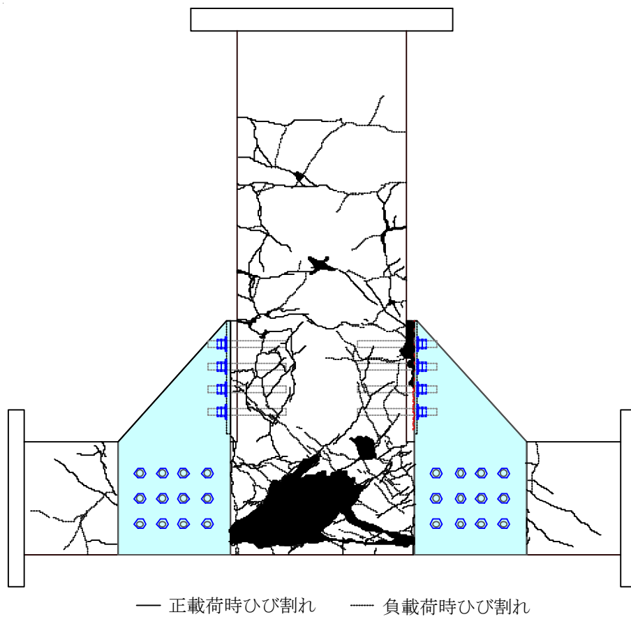
(a) 全体損傷状況
