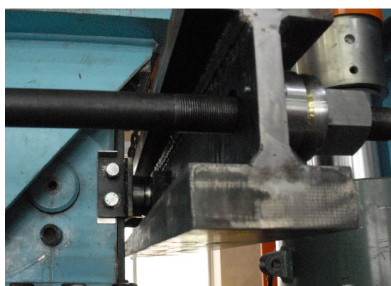
(d) 詳細写真：治具 B と柱端の接続
