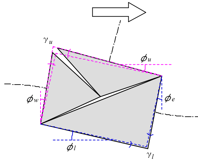
(a) 正載荷
