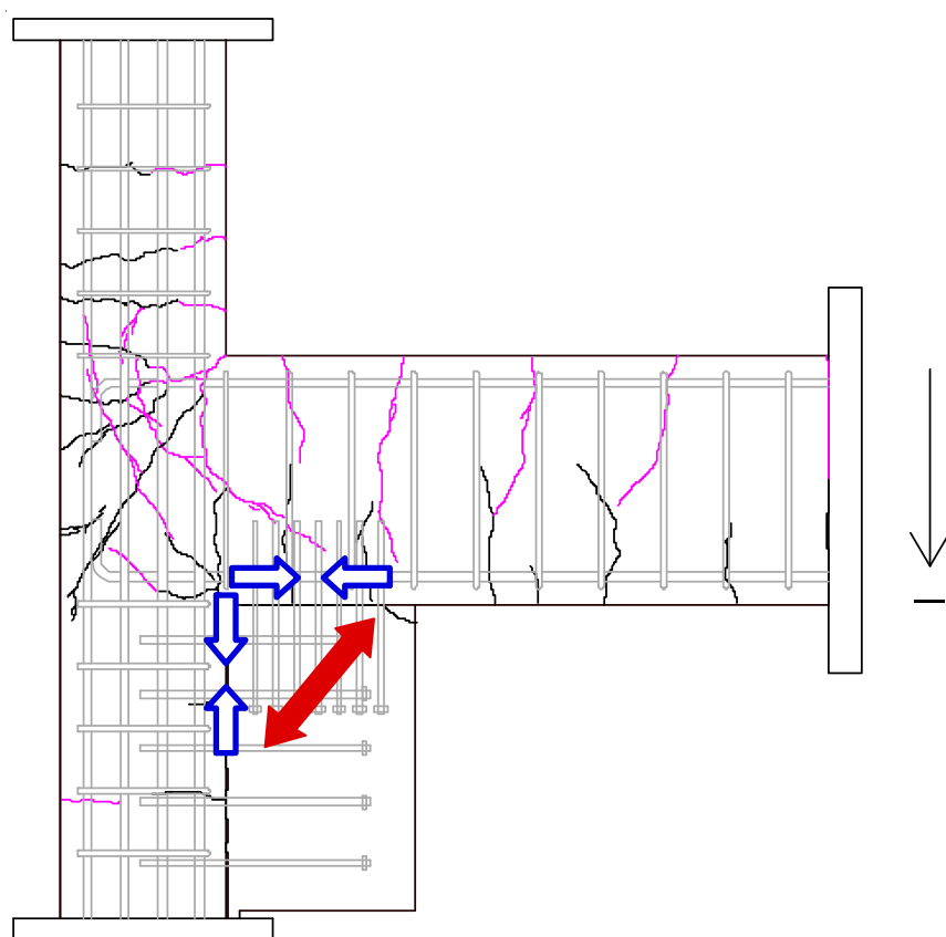
図 6.4.4 下層補強試験体の負荷荷時に形成されるトラス機構 ( R=1/300\text{rad} .サイクル)
