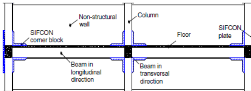
(a) 補強のイメージ
