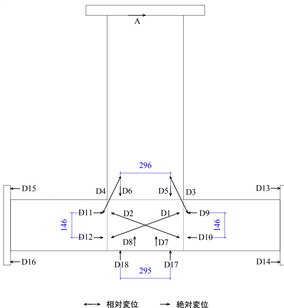
図 3.2.3 変位計計画
