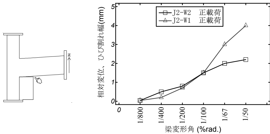
(c) 両補強試験体の正載荷時の比較
