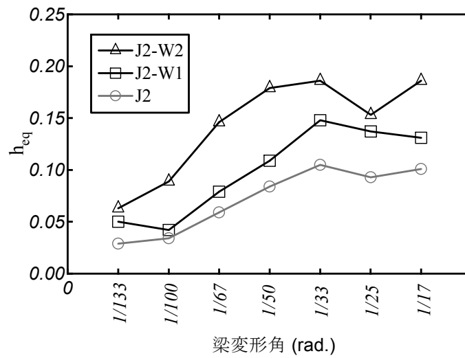
(a) 正載荷
