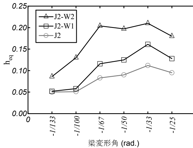
(b) 負載荷
