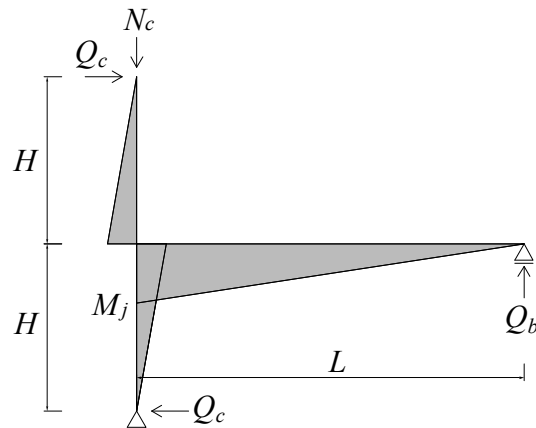
(a) 地震時荷重状態
