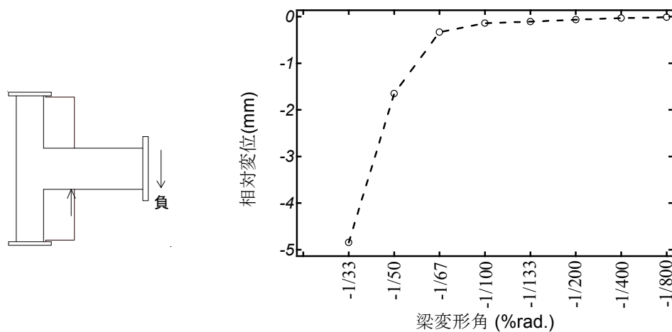
(b) J2-W2 負载荷方向 (図 5.3.8 の D21 より)
