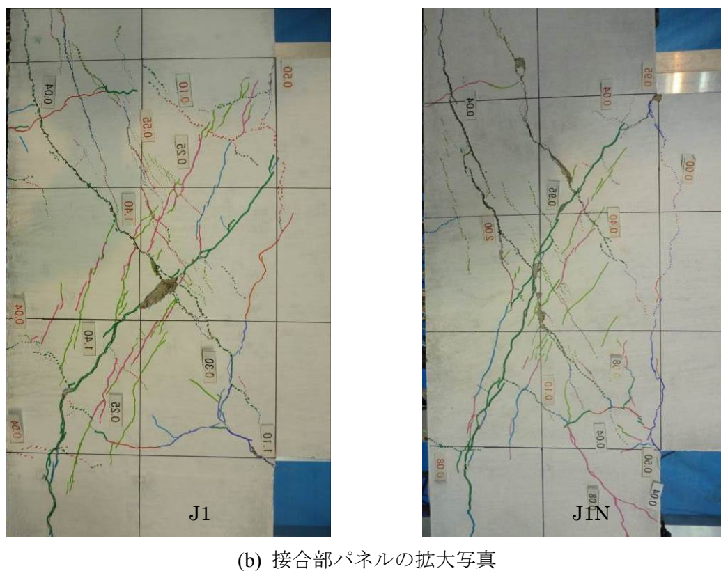
図 3.3.4 R=1/67 サイクル終了時損傷状況
