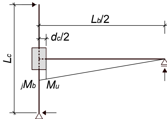
図 3.3.2 梁降伏時節点モーメント
