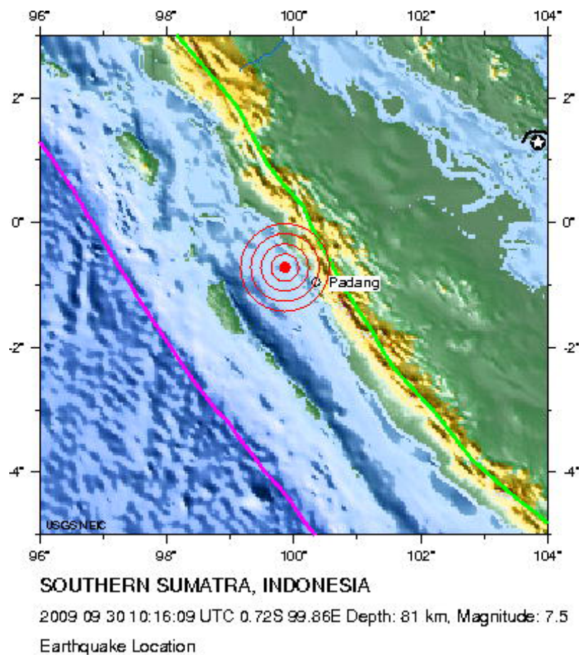
図 1.2.1 震源 14)
