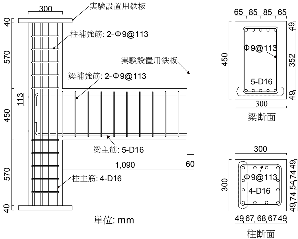
図 3.2.1 試験体形状および配筋
