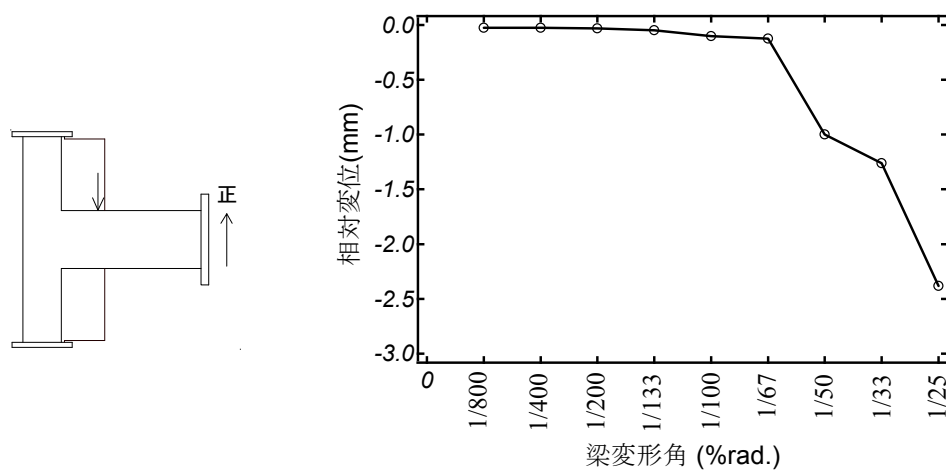
(a) J2-W2 正载荷方向 (図 5.3.8 の D25 より)
