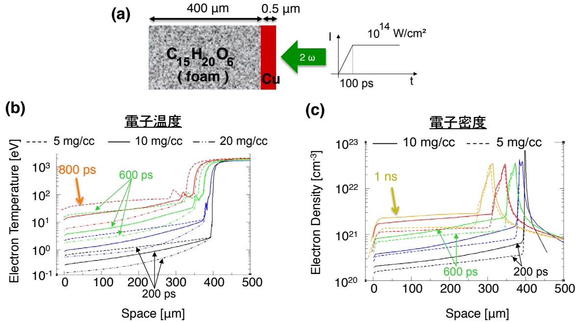
図 4.2.2: (a) シミュレーションセットアップ. 0.5 \mu\text{m} 厚の銅薄膜に強度 10^{14} \text{ W/cm}^2 のレーザーを照射することによって高輝度な X 線を発生させる. その X 線は長さ 400 \mu\text{m} のプラスチックフォームを加熱する. (b) 電子温度の時間発展. レーザーの照射から 800 \text{ ps} 経過するとフォームの電子温度は 10 \text{ eV} から数 10 \text{ eV} まで加熱される. (c) 電子密度の時間発展. レーザーの照射から 1 \text{ ns} 経過すると空間的に一様な密度制御されたプラズマが形成される.
