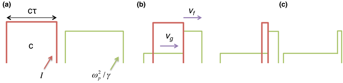
図 2.4.3: レーザーパルス伝搬距離に関する概念図. 赤及び緑線はレーザー強度, 相対論的なプラズマ周波数を示している. (a) 一様なプラズマ領域に侵入する一様強度をもつ長さ c\tau のレーザーパルスがプラズマ中を伝搬すると, (b) レーザー光先端は伝搬速度 v_f で伝搬するのに対してパルス内部はレーザー光の群速度 v_g で伝搬する. そのためにレーザー光がプラズマ中を伝搬するに従ってレーザーパルスの長さは短くなる. (c) 群速度 v_g で伝搬するレーザー光の後尾がその先端位置に追いつけばレーザー光の伝搬が停止する.
