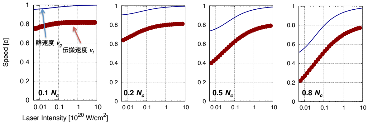
図 2.4.2: レーザー強度とプラズマ電子密度に依存するレーザー光の伝搬速度を赤丸で、群速度を青線で示した。上段は超臨界密度プラズマ、下段は未臨界密度プラズマとした。ここからレーザーの伝搬速度はレーザーの群速度に比べて 0.2c から 0.4c 程度遅いことがわかる。加えて、対象プラズマの電子密度と相対論的臨界密度が近くなればレーザー光の群速度と伝搬速度の差が小さくなることがわかる。
