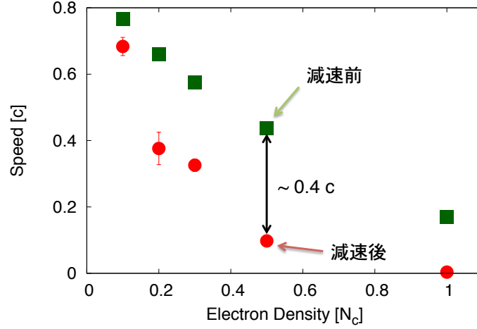
図 5.5.1: 強度 10^{18} W/cm 2 のレーザーを一樣なプラズマに対して照射した際に得られる伝搬速度. 緑四角, 赤丸はそれぞれ伝搬速度が異常低下する前後の結果を示している. 対象プラズマの電子密度が 0.5 N_c である場合, その前後の速度差は \sim 0.4 c である.
