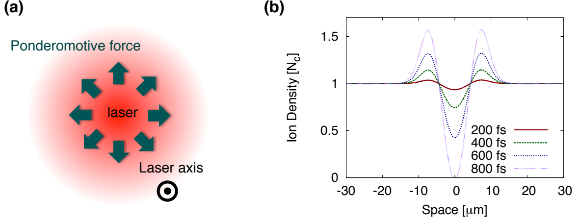
図 2.2.1: (a) レーザー半径方向に働くポンデラモーティブ力. 一般的にレーザー光はビーム中心でその強度を最大とするため, ポンデラモーティブ力はビームの中心から外側へ向かって働く. (b) (2.2.28) 式に基づいて計算されたプラズマチャンネルの時間発展. 赤, 緑, 青, 紫線はそれぞれレーザー光が入射されてから 200, 400, 600, 800 fs 経過した際のイオン密度分布を表している.
