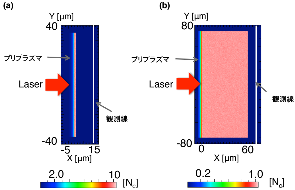
図 4.3.1: (a) 平板ターゲットを模擬したシミュレーションに用いたプラズマの初期電子密度分布. 80\ \mu\text{m} \times 25\ \mu\text{m} のシミュレーションボックス中に 70\ \mu\text{m} \times 1\ \mu\text{m} , 10\ N_c のプラズマを設置した. そのプラズマにはスケール長 1\ \mu\text{m} のプレプラズマが加えられている. (b) 臨界密度プラズマを模擬したシミュレーションに用いたプラズマの初期電子密度分布. 160\ \mu\text{m} \times 80\ \mu\text{m} のシミュレーションボックス中に 140\ \mu\text{m} \times 60\ \mu\text{m} , 1\ N_c のプラズマを設置した. そのプラズマにはスケール長 2\ \mu\text{m} のプレプラズマが加えられている.
