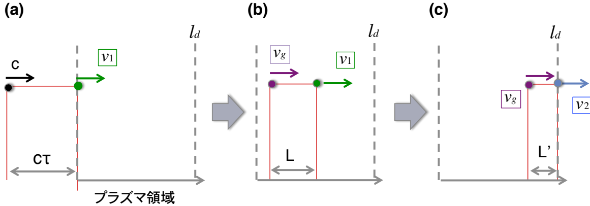
図 5.4.2: 伝搬速度が減速した後も伝搬し続けるレーザーパルス伝搬距離. (a) パルス長 c\tau のレーザーがプラズマ領域に侵入すると、その先端は伝搬速度 v_1 でプラズマ中へ侵入する. (b) パルス先端は伝搬速度 v_1 で伝搬するのに対して、パルス内部は群速度 v_g で伝搬する. そのため、プラズマ中を伝搬するに従って、そのパルス長 L が縮む. (c) パルス先端が伝搬速度の異常低下を引き起こす位置 l_d に到達する場合、それ以降の先端の伝搬速度を v_2 とする. 尚、パルス内部は (b) と同様に群速度 v_g で伝搬する. このような伝搬が続きパルス長 L' が L' = 0 となった位置を伝搬距離とする.
