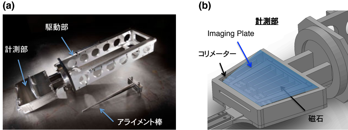
図 3.2.1: (a) OMEGA 施設において使用するために開発した多方向電子エネルギー spektrometer. これは駆動部, 計測部, アライメント棒によって構成されている. 駆動部は真空チャンバポートに予め取り付けられた駆動装置 (TIM) と連結し, 計測部を所定の位置まで運ぶ. 計測部に取り付けたアライメント棒の先端が tcc に合うように計測部のアライメントを行う. (b) 計測部の概要. 計測部は5つのコリメーターと5対の磁石, 1枚の Imaging Plate によって構成される. ノイズを抑えるために計測部は SUS 製の箱によって囲われている. ターゲットから放出された高速電子はその箱に開けられたスリットを通り抜ける. スリットを通り抜けた高速電子はコリメーターを通過した後, 磁石によってエネルギー分解され, 検出器である IP に入射する.
