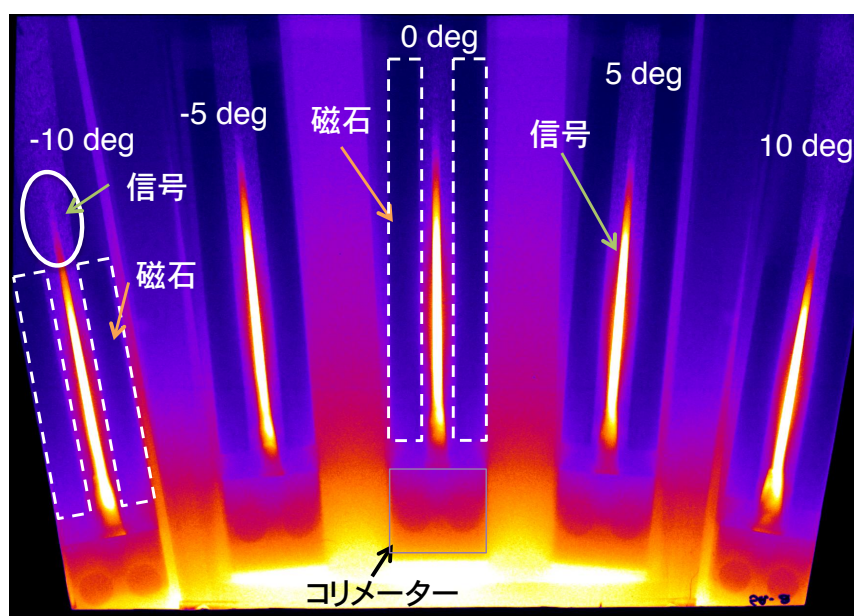
図 3.2.3: MCESM によって観測された信号の例. 2 枚の磁石と 1 つのコリメーターによって構成された 1 つの ESM が, それぞれ異なった角度方向から高速電子のエネルギースペクトルを観測する. 点線内で囲まれた領域に磁石が配置され, その間に電子による信号が確認できる. -10^\circ , 及び 10^\circ の位置における磁石の長さはその他の磁石よりも短く設計されている.
