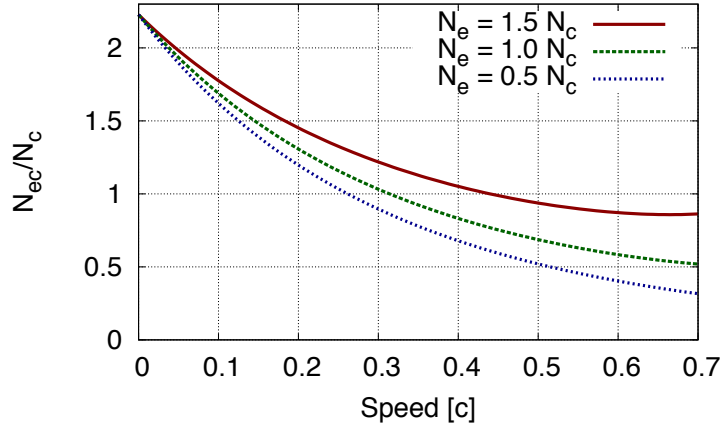
図 5.2.1: プラズマの流速に依存する実効的な相対論的臨界密度. ただし, レーザー強度は I = 10^{19} W/cm 2 とした. 赤実線, 緑破線, 青点線はそれぞれ電子密度が 1.5 , 1.0 , 0.5 N_c の場合を示している. 例えば電子密度が 1.0 N_c の場合, プラズマの流速が 0.3 c を超えると N_{ec} が 1.0 N_c を下回る. そのため, その対象プラズマは入射レーザーに対して超臨界密度プラズマとして作用する.
