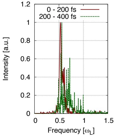
図 5.3.4: (a) 反射光スペクトル. 赤実線は時刻 0 fs から 200 fs までの, 緑点線は時刻 200 fs から 400 fs までの観測結果である. 0.72 \omega に対応する反射体の速度は 0.19 c となり, 先端領域が超臨界密度プラズマとなる閾速度 0.17 c と近い値を示している. また, 0.53 \omega に対応する反射体の速度は 0.42 c であり, 速い時間帯 (0~300 fs) における伝搬速度 0.42 c と一致する. (b) 時刻 400 fs における実効的な相対論的臨界密度で規格化された電子密度 (青実線) とレーザー強度 (赤点線) の空間分布. 実効的に超臨界密度プラズマとなった微小な領域 (島) がレーザー光先端領域において多数形成されている.
