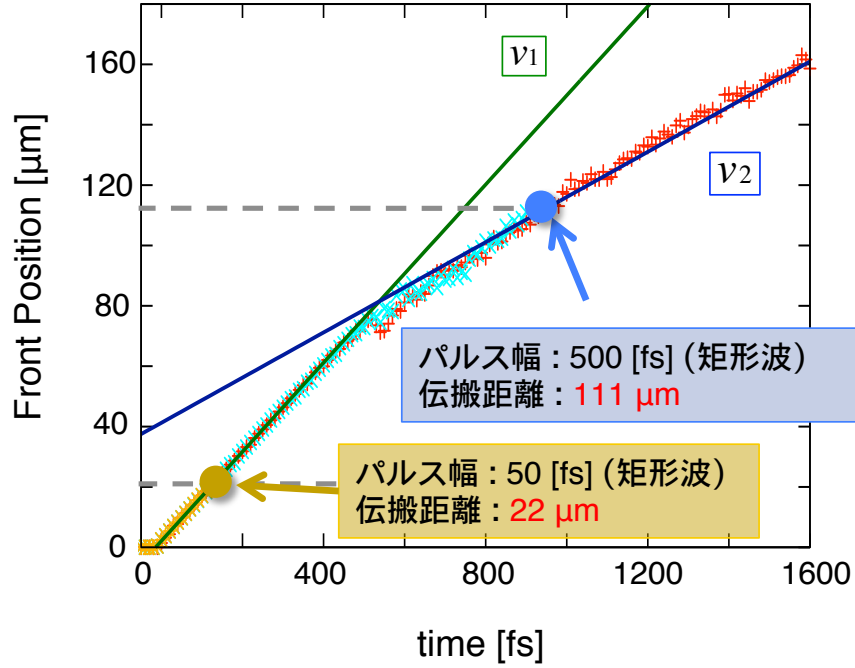
図 5.4.1: 一様な臨界密度プラズマに対して強度 2 \times 10^{19} \text{ W/cm}^2 のレーザーを照射した際に得られたレーザー光先端位置の時間発展. 赤, 青, 黄色はそれぞれパルス幅を半無限, 500 fs, 50 fs とした場合の結果である. v_1, v_2 の傾きが減速前後の伝搬速度を表している.
