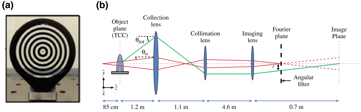
図 3.3.1: (a) 角度フィルター。プラズマを通過することによって曲げられた光をこのフィルターによって部分的に遮る。(b) 光学系の配置図。tcc において生成されたプラズマを通過した光はその密度に応じた角度を持って集光レンズに入射する。その後、その光は2枚のレンズを用いて観測位置まで転送される。角度フィルターはイメージングレンズの焦点に設置されている。この角度フィルターはプローブからの直接光を遮断し、加えてプラズマによって曲げられた光を部分的に遮る。フィルターを通過した光を観測することによってプラズマによって曲げられたプローブ光の角度を見積もることができる。
