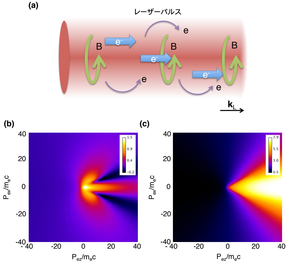
図 2.3.2: (a) 磁場巡回加速の原理. 超高強度なレーザー光がプラズマ中を伝搬するとプラズマチャンネルが形成される. そのプラズマチャンネル中の電子はレーザーによって前方方向へ加速させる. 加速された電子によって生み出される電流はアンペールの法則によって軸対称な磁場を発生させる. その磁場はプラズマチャンネルを抜けようとする電子を引き戻す. 引き戻された電子は再度レーザー光によって加速される. (b) 初期運動量を持った電子が新たにレーザー光からの作用を受けることによって得るエネルギーの分布. ただし, そのエネルギーは m_e c^2 \sqrt{1 + \frac{1}{2} \frac{I}{I_{th}}} によって規格化されている. (c) 1 周期のレーザーが初期運動量を持った電子に作用する時間. ただし, その時間はレーザーの周期によって規格化されている.
