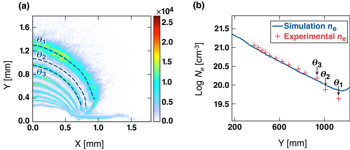
図 3.4.2: (a) AFR によって観測された初期プラズマ密度分布. それぞれの縞模様がプラズマによって曲げられたプローブ光の屈折角 \theta に対応し, その角度から電子密度を算出する. (b) ターゲット表面からの距離 Y に対する電子密度. 青実線は流体シミュレーションから得られた結果, 赤点は屈折角 \theta から見積もられる電子密度である.
