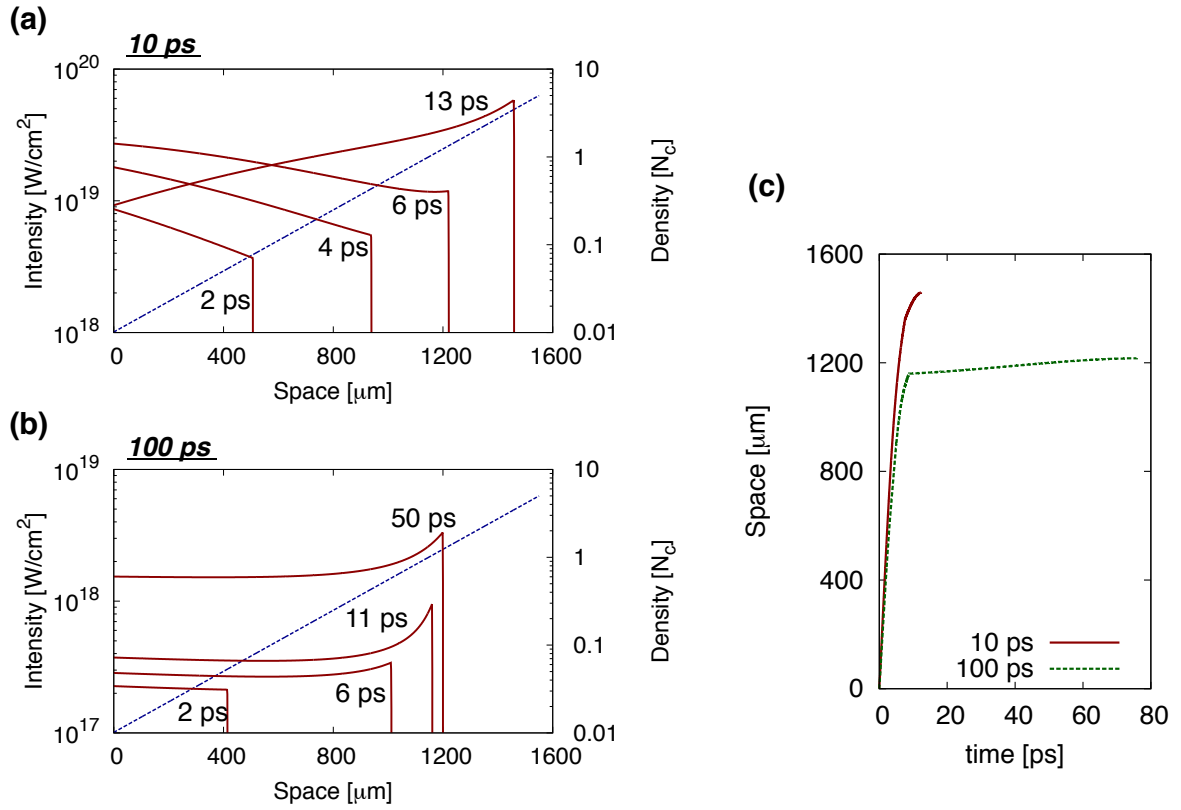
図 3.5.1: (a) パルス幅 10 ps の超高強度レーザーをスケール長 250 \mu\text{m} のプラズマに照射した際のレーザー強度の時間発展. (b) パルス幅 100 ps の超高強度レーザーをスケール長 250 \mu\text{m} のプラズマに照射した際のレーザー強度の時間発展. (c) レーザー光先端位置の時間発展. 赤実線, 緑点線はそれぞれパルス幅 10 ps, 100 ps の結果を示している.
