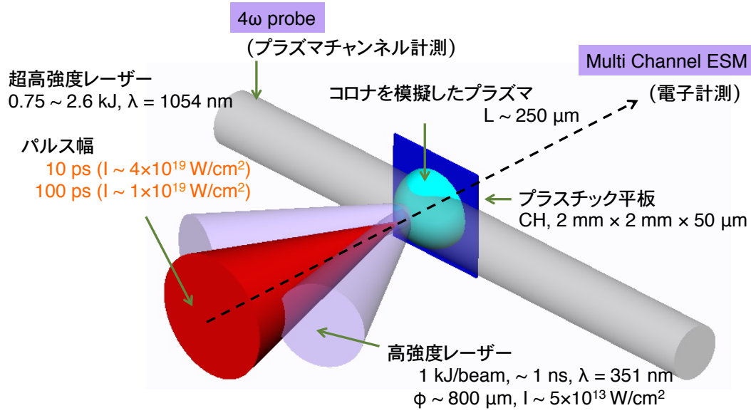
図 3.4.1: 実験セットアップ. 高強度レーザーをプラスチック平板に照射することにより生成されるアブレーションプラズマに対して超高強度レーザーを照射した. レーザー光の伝搬の様子は 4\omega プロブによって, 生成される高速電子の特性は MCESM によって観測される.
