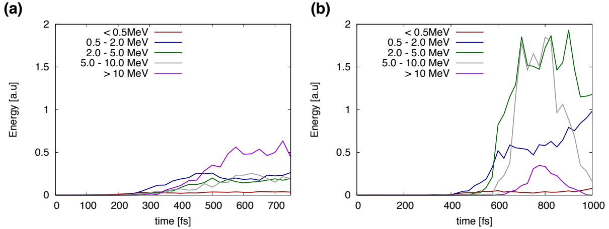
図 4.5.1: 単位時間当たりに観測線を通過する電子のエネルギー. 赤, 青, 緑, 灰, 紫の線はそれぞれの電子のエネルギー帯が < 0.5 , 0.5 \sim 2.0 , 2.0 \sim 5.0 , 5.0 \sim 10.0 , > 10.0 MeV である. 平板ターゲットの結果は (a), 臨界密度プラズマの結果は (b) に示されている. 平板ターゲットの場合, 高エネルギーな電子がターゲットを抜けて観測された. 一方, 臨界密度プラズマの場合, 磁場によるコリメーションを受けた数 MeV 以上のエネルギーを持つ電子が数多く観測された.
