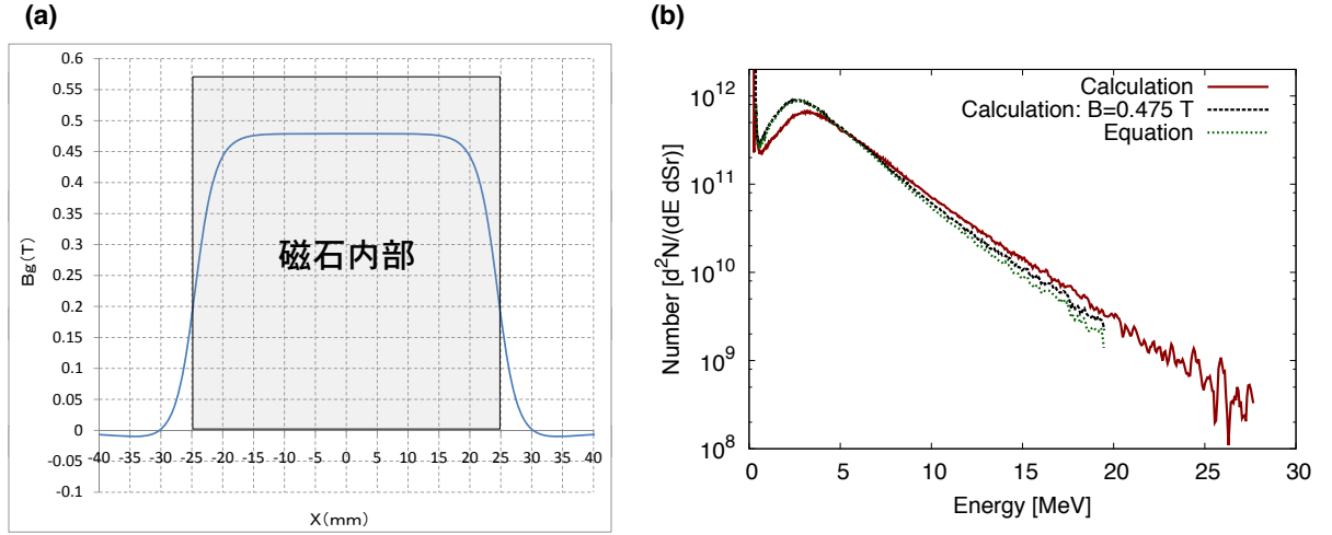
図 3.2.4: (a) 長さ 49 mm の磁石の長さ方向の磁場分布. 中心 x = 0 mm 近辺では一定の磁場が得られているが, x = \pm 20 mm 近辺からその強さは低下する. 加えて磁石の外側においても微弱的な磁場が存在する. (b) 各手法によって得られたエネルギースペクトル. 緑点線は (3.2.9), 及び (3.2.6) 式から得られた結果である. 黒実線は磁石に挟まれた領域における磁場の強さを一定とした場合を数値計算によって求めた結果である. 赤実線は不均一磁場を数値計算に適応して求めた結果である.
