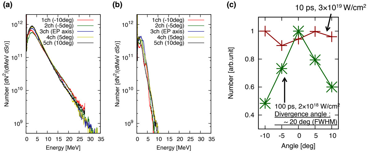
図 3.4.4: (a) パルス幅 10 ps の超高強度レーザーを照射した際に得られた電子のエネルギースペクトル. 傾き電子温度は 3 ~ 4 MeV であった. (b) パルス幅 100 ps の超高強度レーザーを照射した際に得られた電子のエネルギースペクトル. 傾き電子温度は 1 ~ 2 MeV であった. (c) 電子の放出角度分布. パルス幅が 10 ps の場合を赤線で, 100 ps の場合を緑線で示している. パルス幅が 100 ps であった場合, 発生した高速電子ビームに 20° (FWHM) 程度の指向性を確認できる. 尚, 縦軸は各ショットでの最大値で規格化した.
