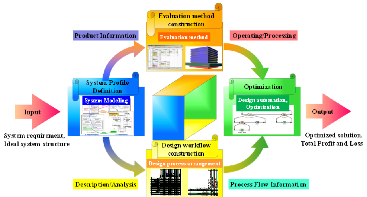
Fig. 2.3 SDSI-Cubic method.
