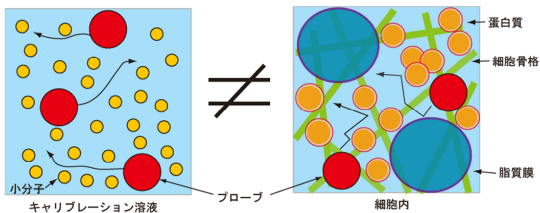
図 4 キャリブレーションに用いる小分子の溶液と細胞内の模式図
