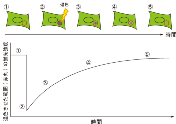
図2 FRAPの概略図
