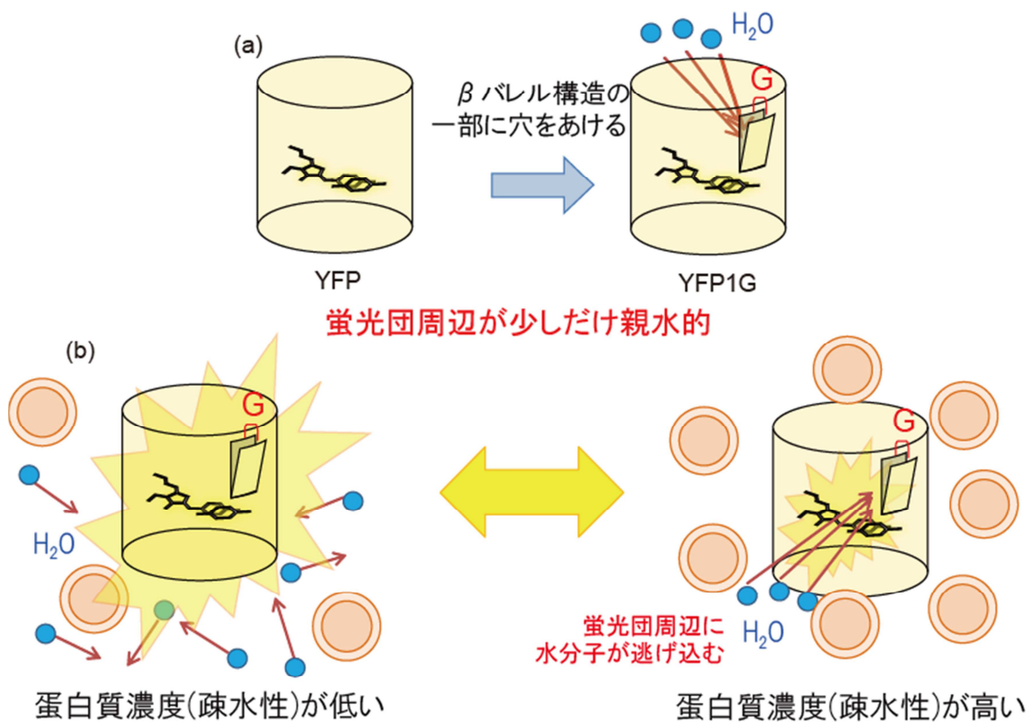
図 20 YFP1G が蛋白質濃度(疎水性)を感受するメカニズム
