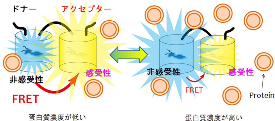
図8 蛋白質濃度感受性 FRET プローブの概略図
