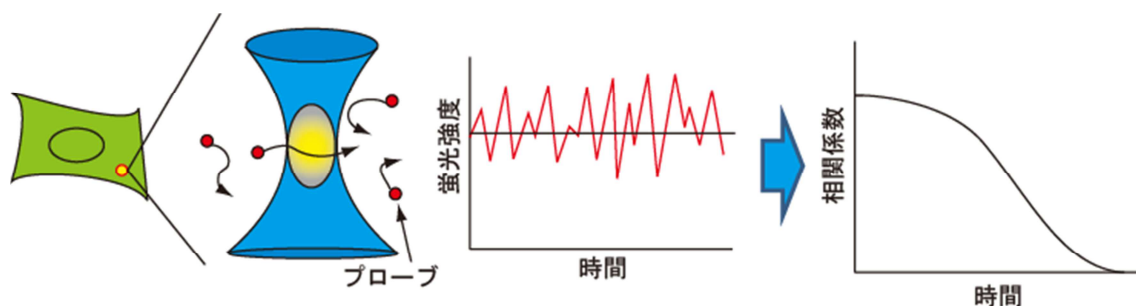
図 3 FCS の概略図
