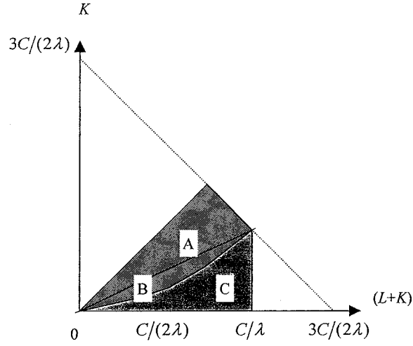
図 5-2. 2-ユニットシステムの最適政策 手元に無限個のユニットがある場合
