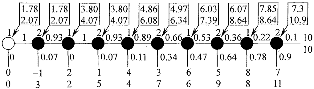
図 7-3. Rosenthal のモデル
