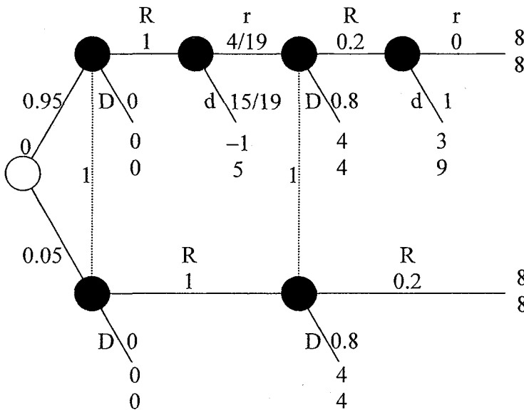
図 7-4. Myerson のモデル
