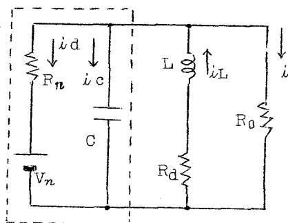
図 3 . 3 過渡状態の等価回路
