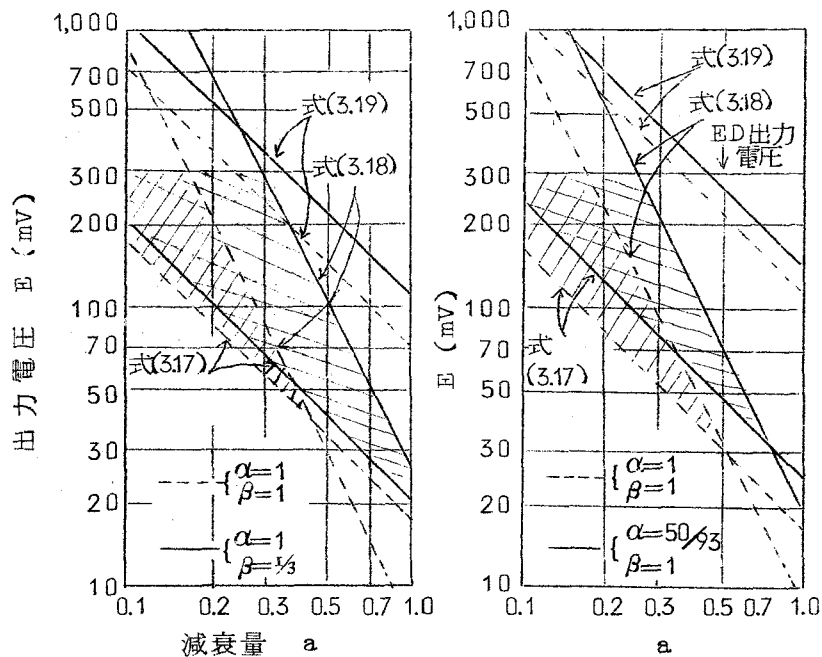
図 3.13 動作限界と R_T, R_L との関係
