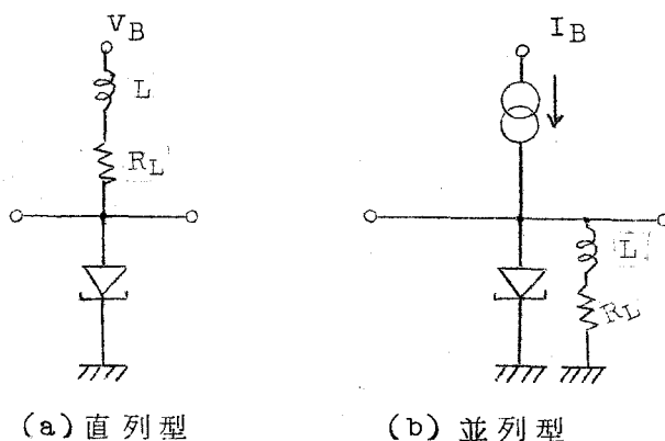
図 2.1 基本回路
