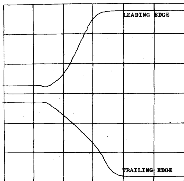
図 4 . 5 出力波形 (垂直軸：200mV/div. 水平軸：1ns/div.)
