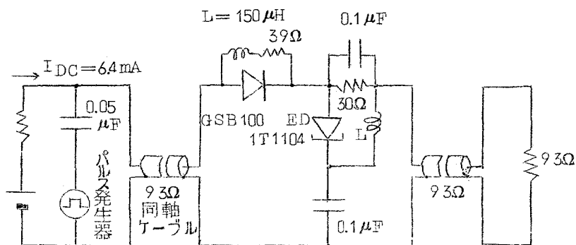
図3.5 測定回路
