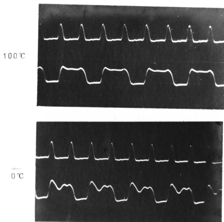
図 2.20 周囲温度による影響
