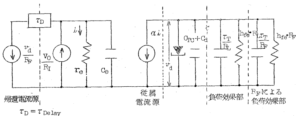
図 5.5 等価回路
