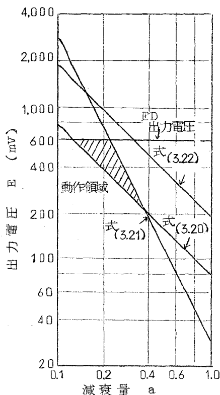
図3.16 ガリウム砒素( GaAs )エサキダイオードを用いた場合の動作限界
