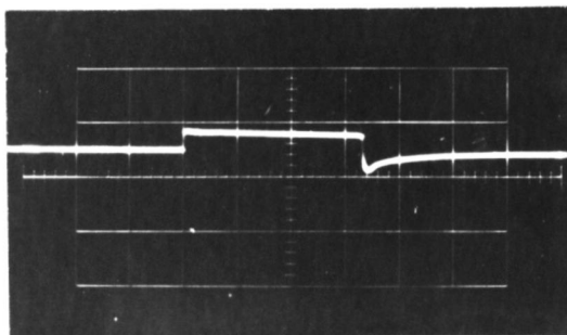
図 2.11 入力パルスでリセットされない場合の出力電圧波形
