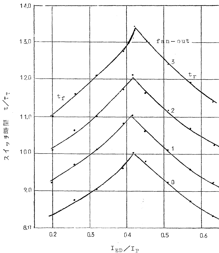
図 5.10 スイッチ時間と動作点
