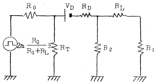
図 3.10 トリガ時の等価回路
