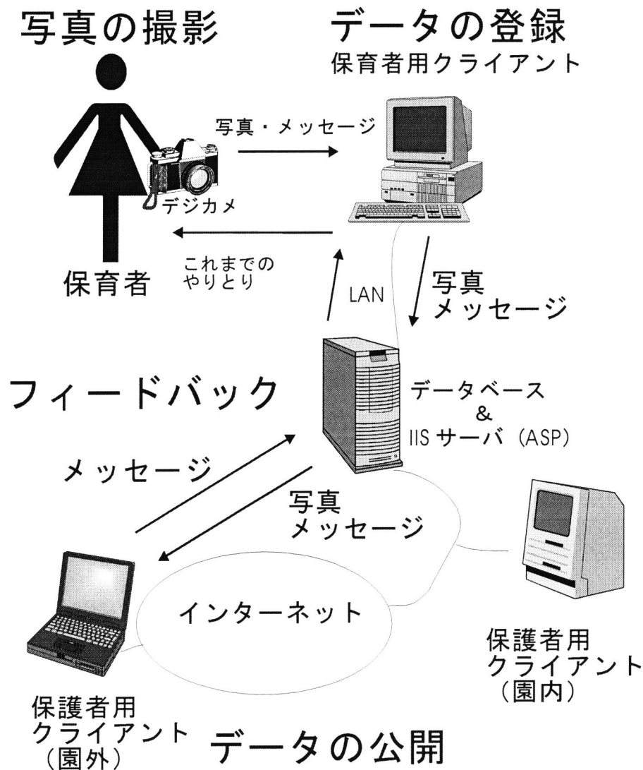
図2-1 システムの構成
