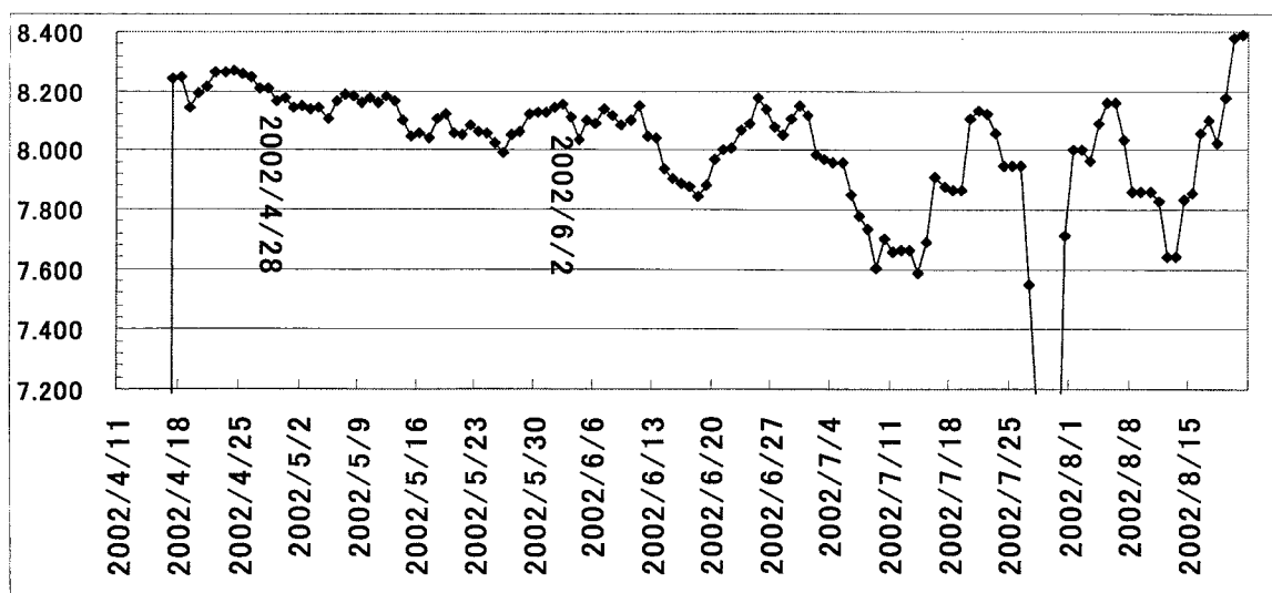
図4-6 1週間累積エントロピーの時系列変化(単位ビット)
