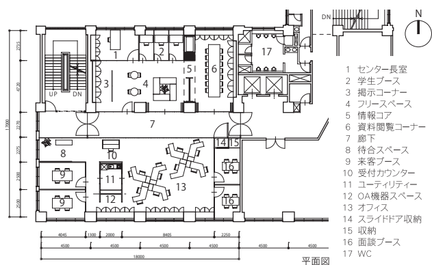
平面図
