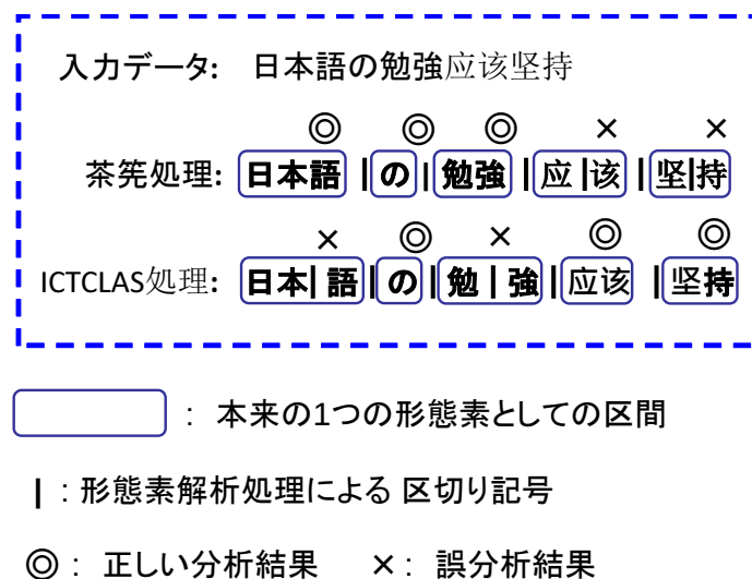
図 4.1: 両言語が混在する文の形態素解析結果の例
