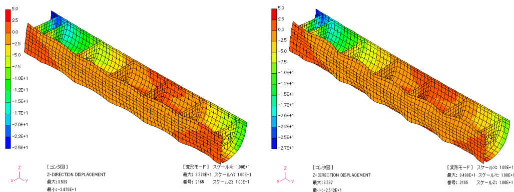
(a) 微小変形解析 (最大変位=3.5 mm) (b) 大変形解析 (最大変位=3.5 mm) 図 5.7 溶接局部変形による捩れ変形 (Case-A2).
