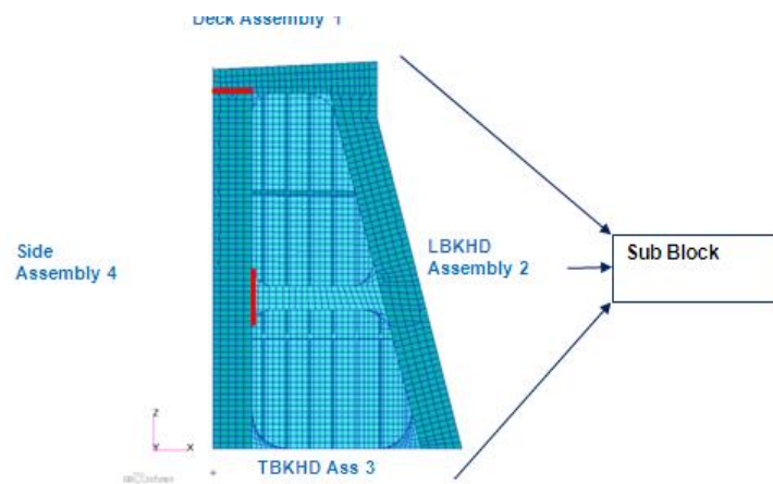
図4.5.3 4つの中組立部材
