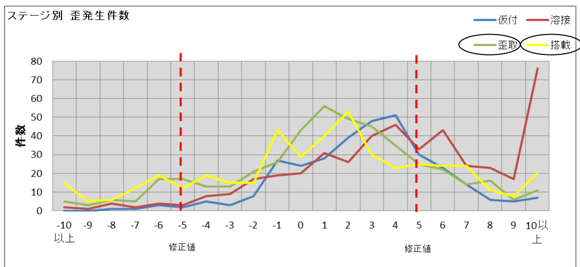
図 6.19 実船での各ステージでの歪み発生傾向
