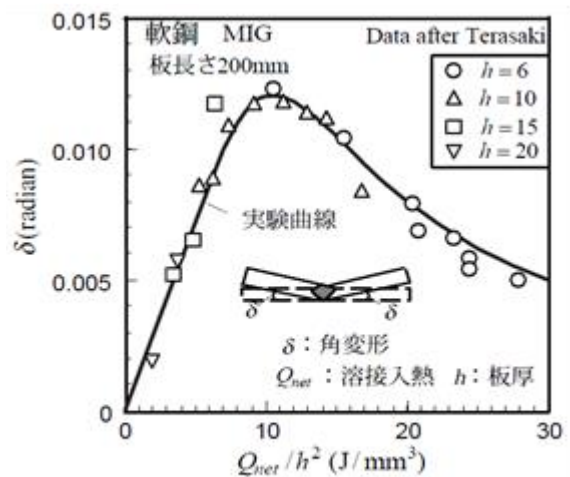
図 3.5: 縦収縮に及ぼす溶接入熱の影響
