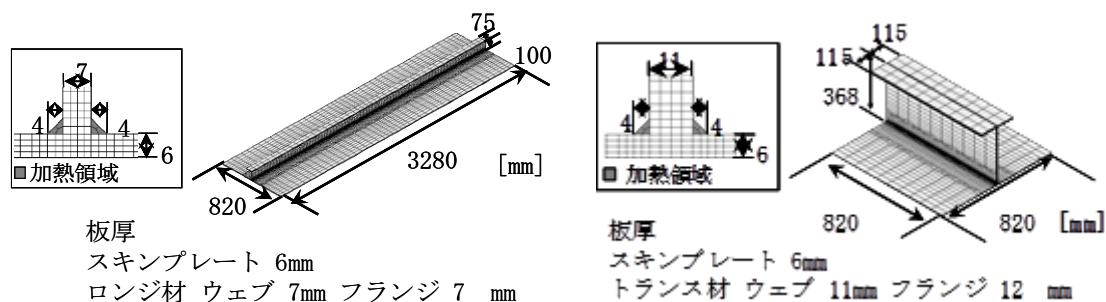
図 3.6 熱弾塑性解析用防撓材付きモデル
