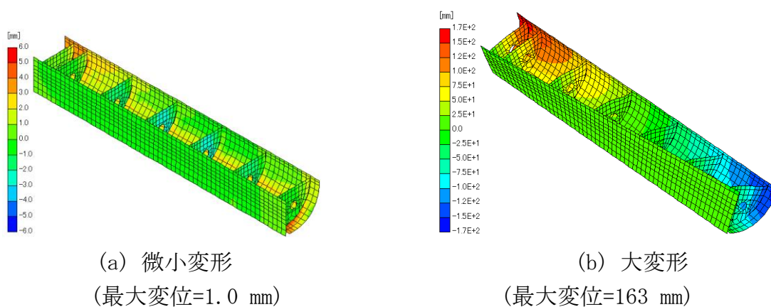
図 5.10 ギャップ矯正により生じた捩れ変形 (Case-C2)
