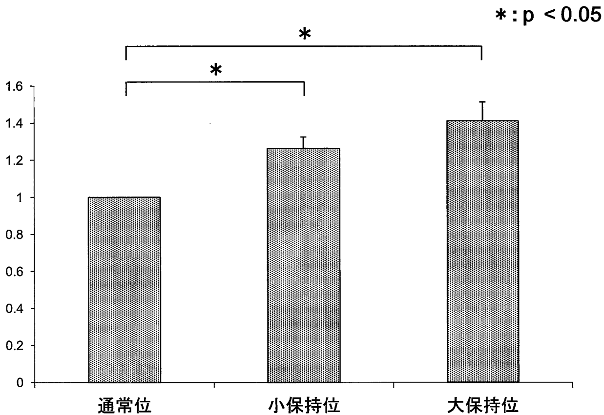
図12 測定タスク間における筋活動時間の比較 (バー:標準誤差)
