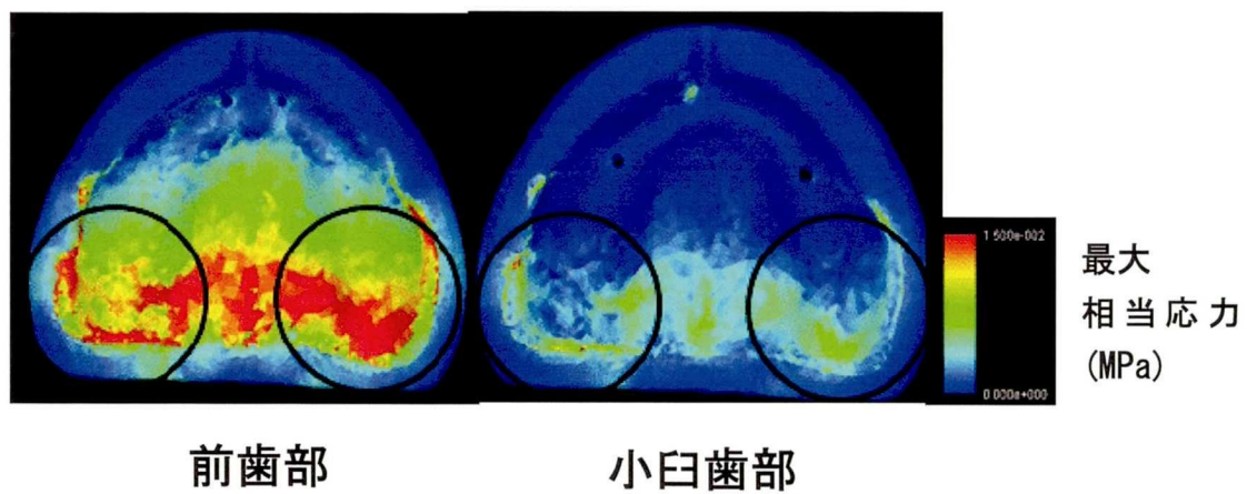
図 14 粘膜の相当応力分布図（前歯部と小臼歯部）
