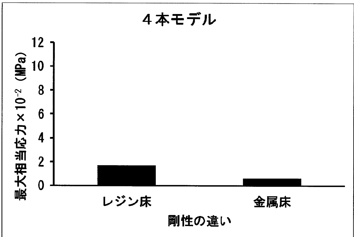
図 28 粘膜の最大相当応力（レジン床と金属床）
