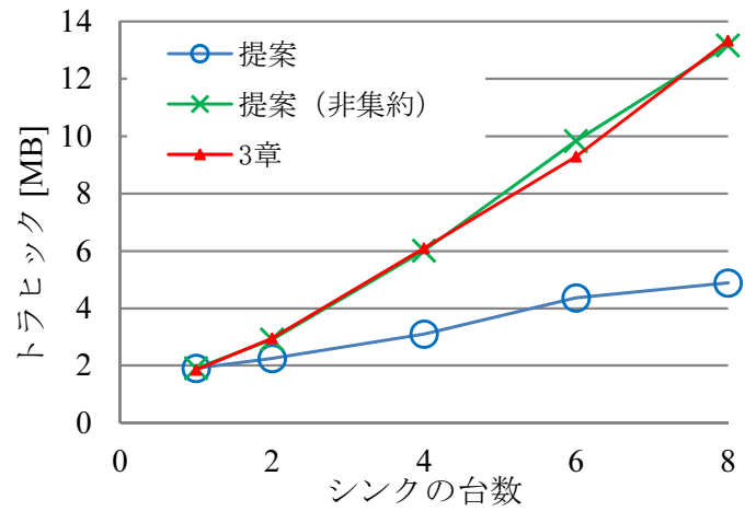
図 4.8: シンクの台数の影響：トラフィック
