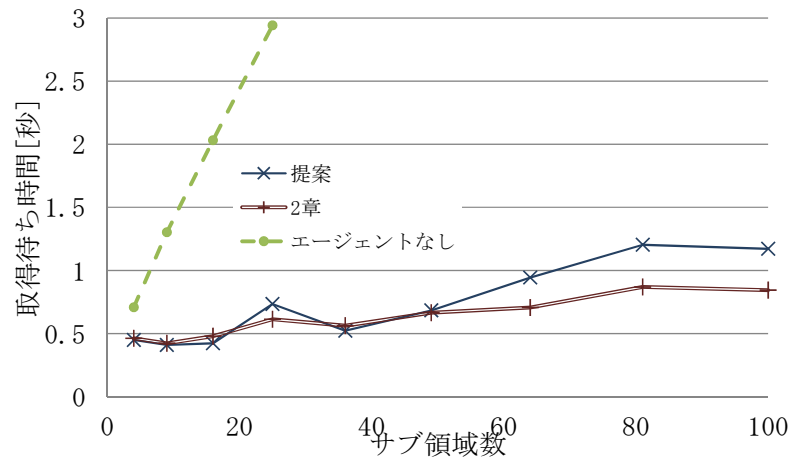
図 3.11: サブ領域数の影響：取得待ち時間
