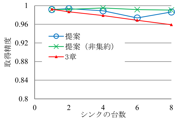
図 4.9: シンクの台数の影響：取得精度
