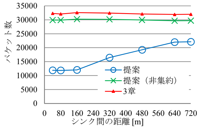
図 4.15: シンク間の距離の影響：パケット数
