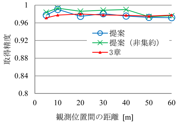
図 4.13: 観測位置間の距離の影響：取得精度
