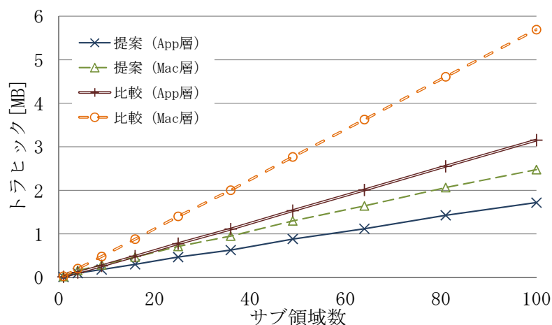
図 2.13: サブ領域数の影響：トラフィック
