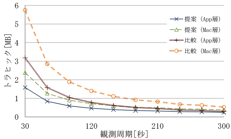
図 2.9: 観測周期の影響：トラフィック
