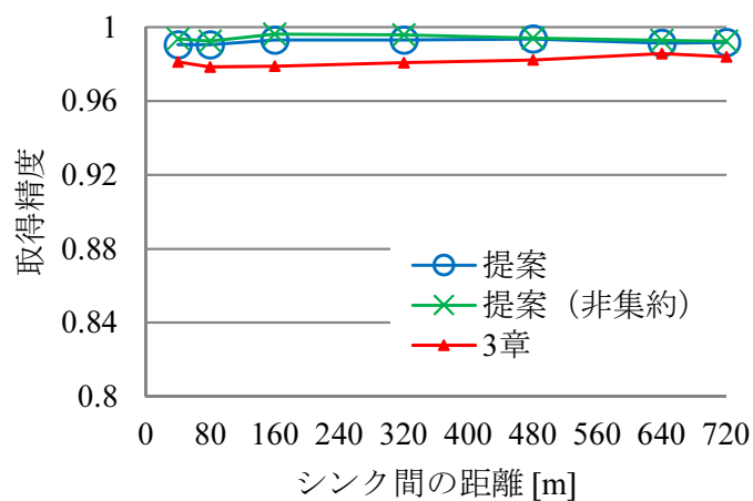
図 4.17: シンク間の距離の影響：取得精度
