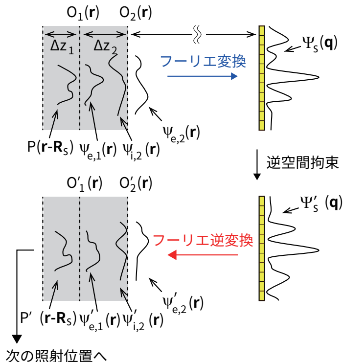
図 6.3 マルチスライスタイコグラフィの位相回復アルゴリズム (3PIE) の模式図. ePIE にマルチスライス法の概念を取り入れることで厚い試料の再構成が可能なアルゴリズムへ拡張した.
