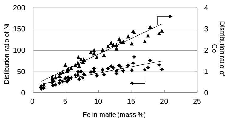
Fig.4-9 マット中の Fe 濃度とマッ トー 転炉スラグ間の Ni、Co の分配比の散布図： ◆; Ni、 ▲; Co.
