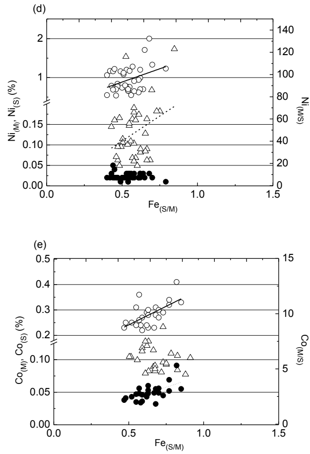
Fig. 2-3 2\text{MS} + \text{O}_2 = 2\text{MO} + \text{S}_2 の標準ギブスエネルギー変化が Fe のそれよりも大きい金属の \text{Fe}(\text{S/M}) と \text{M}(\text{M}) 、 \text{M}(\text{S}) および \text{M}(\text{M/S}) の散布図
