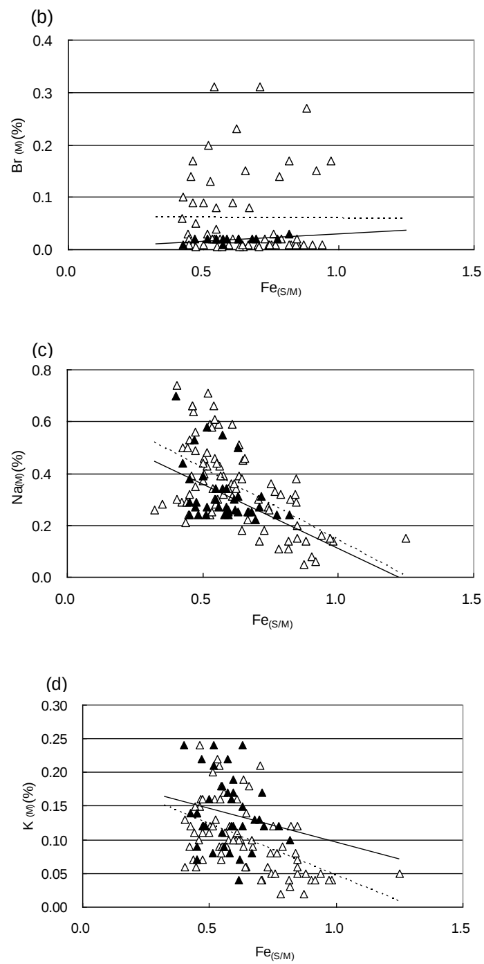
Fig. 2-6 Fe_{(S/M)} と、ハロゲンおよびアルカリ金属のマット中の濃度の散布図 (a) Cl、(b) Br、(c) Na、(d) K \cdots\triangle\cdots ；ダスト洗浄なし、 -\blacktriangle- ；ダスト洗浄実施
