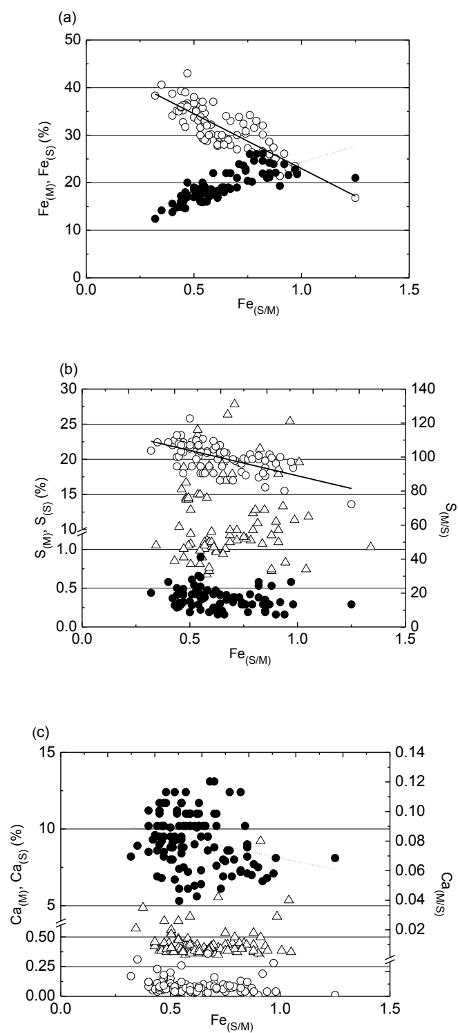
Fig. 2-5 2\text{MS} + \text{O}_2 = 2\text{MO} + \text{S}_2 の標準ギブスエネルギー変化が Fe のそれと同程度か または小さい金属の \text{Fe}_{(S/M)} と M_{(M)} 、 M_{(S)} および M_{(M/S)} の散布図
