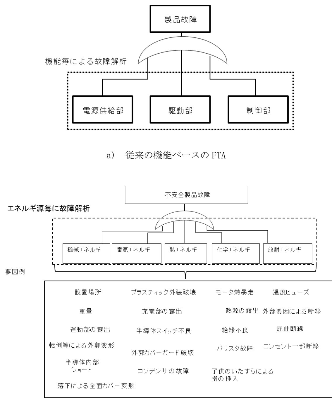
図 2-8 従来の FTA と提案する FTA の相違
