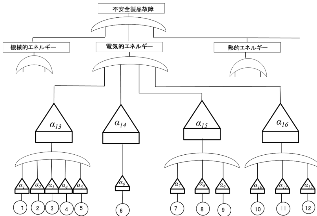
図 2-12 扇風機の手ザードベース FTA
