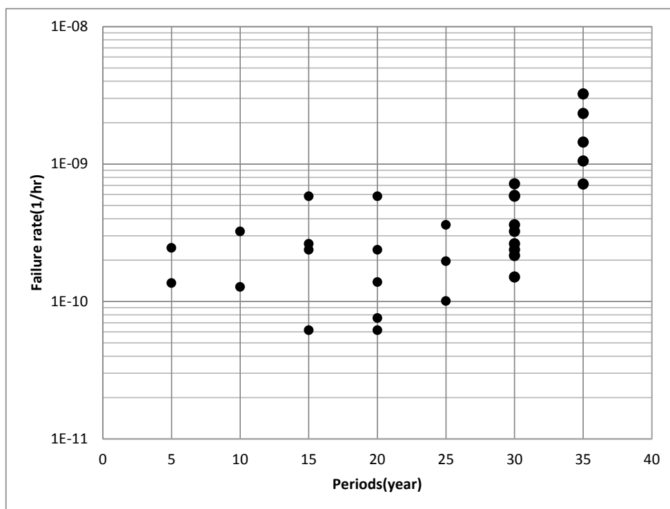
図 3-4 事故報告例から計算された扇風機の故障率
