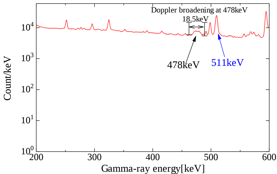
(478keV 付近拡大図) 図 2-25 AmBe 及びホウ酸を設置した場合の HPGe 検出器で測定した PHS
