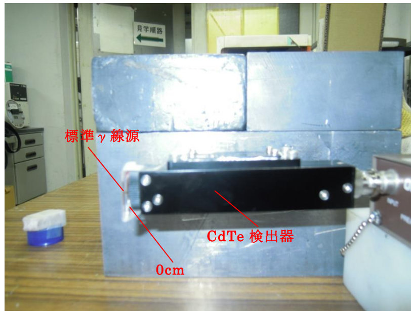
図 2-15 FWHM 測定時の標準 \gamma 線源と CdTe 検出器の距離
