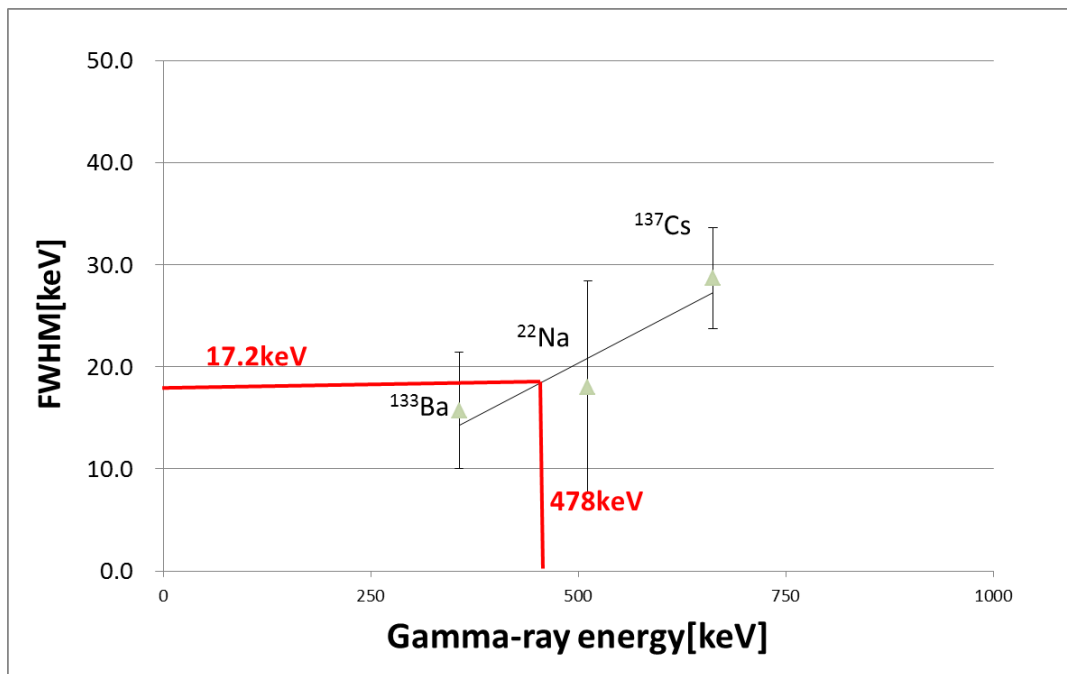
図 4-10 CdTe(2 素子)検出器の FWHM
