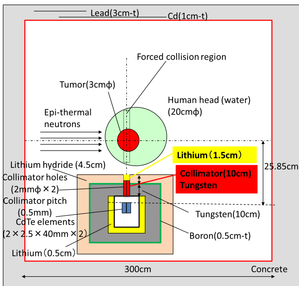
図 3-6 3 番の計算モデル
