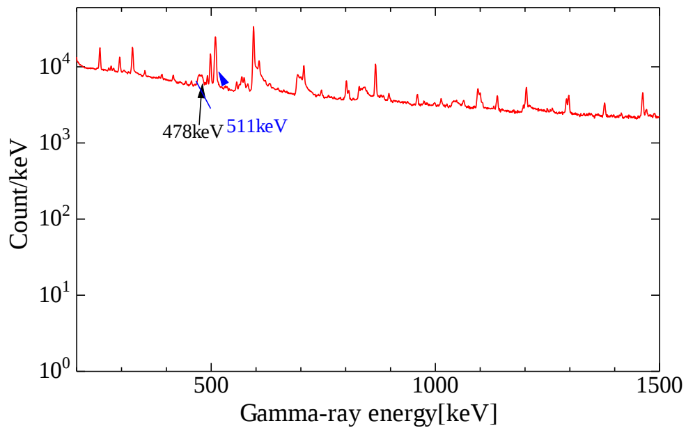
図 2-24 AmBe 及びホウ酸を設置した場合の HPGe 検出器で測定した PHS ( ^{10}\text{B} (n, \alpha ) ^7\text{Li} 反応から放出される 478keV と 511keV \gamma 線が見られる。)
