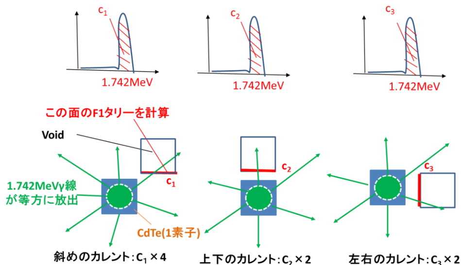
図 3-28 等方で放出する 1.742MeV \gamma 線のカレントを求める計算モデル
