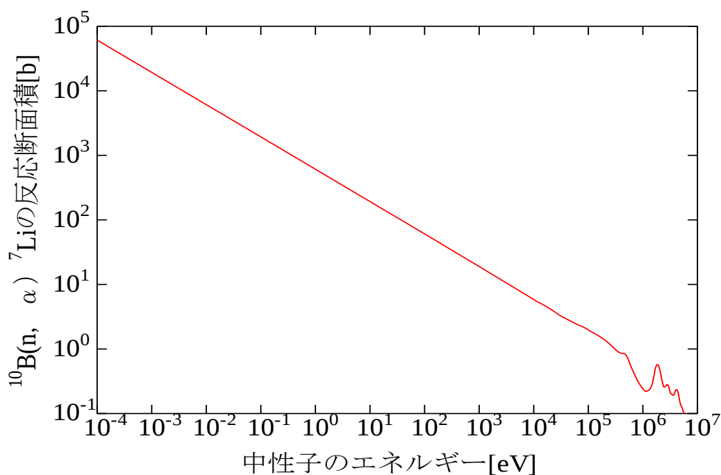
図 1-4 ^{10}\text{B}(\text{n},\alpha)^7\text{Li} の反応断面積
