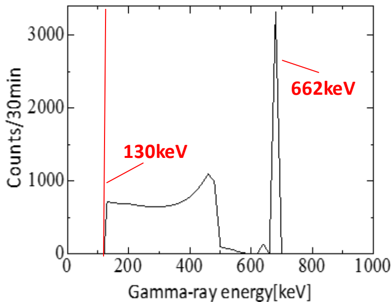
(a)計算で求めた ^{137}\text{Cs} 線源の PHS
