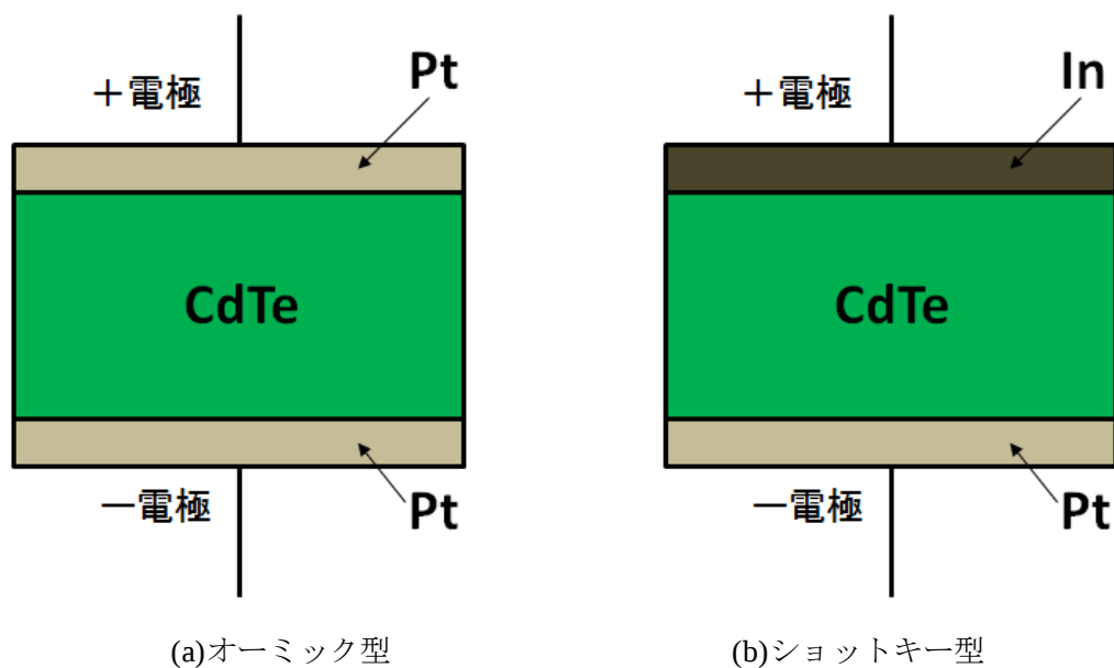
図 2-3 CdTe 素子の種類
