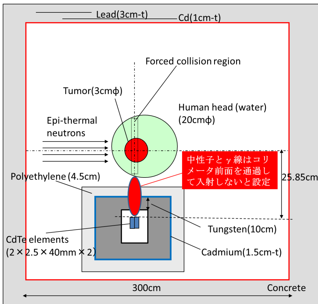
図 3-5 2 番の計算モデル
