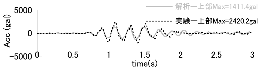
(d) 3.0 倍入力
