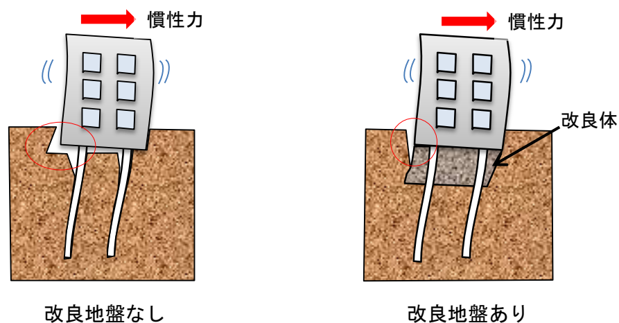
図 1.1.3 杭と改良地盤の周囲地盤の強非線形現象
