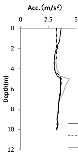
(b) 最大加速度の深さ分布
