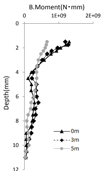
図 4.2.25 杭の最大曲げモーメント分布 (告示神戸位相 0.2 倍・短辺加振)
