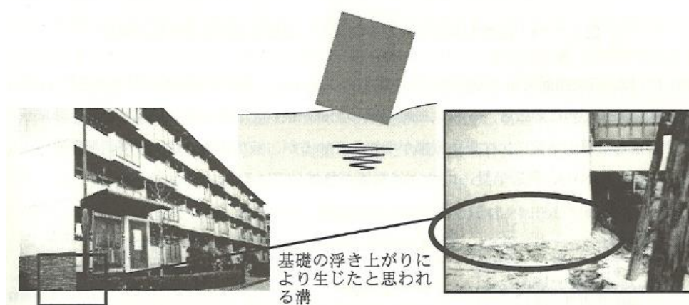
図 1.1.2 直接基礎で支持された共同住宅の基礎浮き上がり 6)
