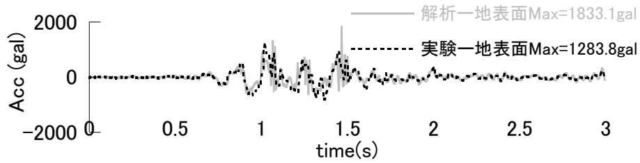
(c) 1.7 倍入力
