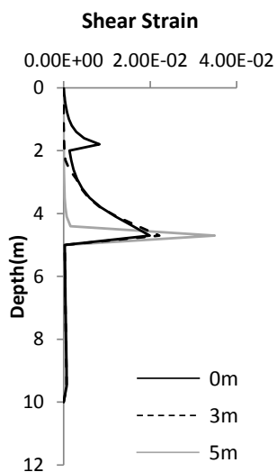
(a) 最大ひずみの深さ分布
