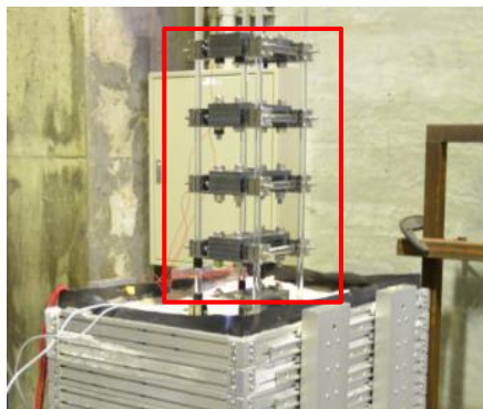
(a) 4 層建物
