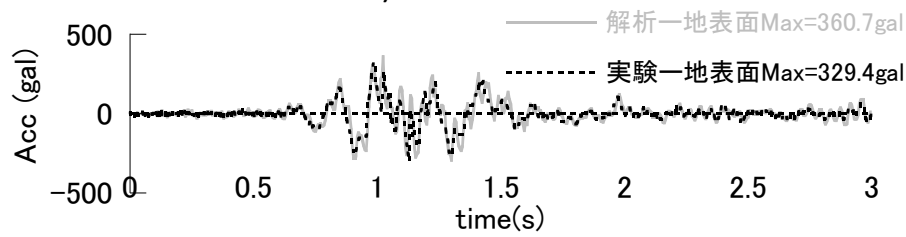
(a) 0.2 倍入力
