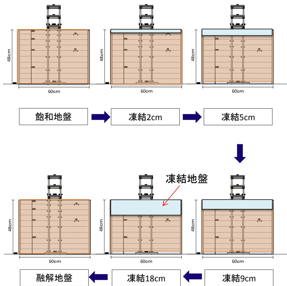
図 3.3.8 実験の流れ
