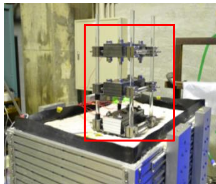
(b) 2 層建物
