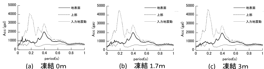
図 4.3.12 地表面、建物上部および入力地震動の加速度応答スペクトル (告示神戸位相 1.0 倍・2 階建物)
