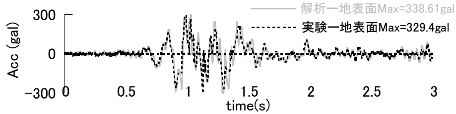
(a) 0.2 倍入力
