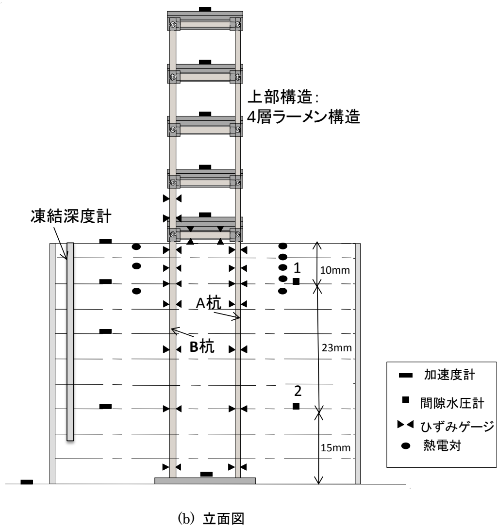
図 3.3.4 実験モデル
