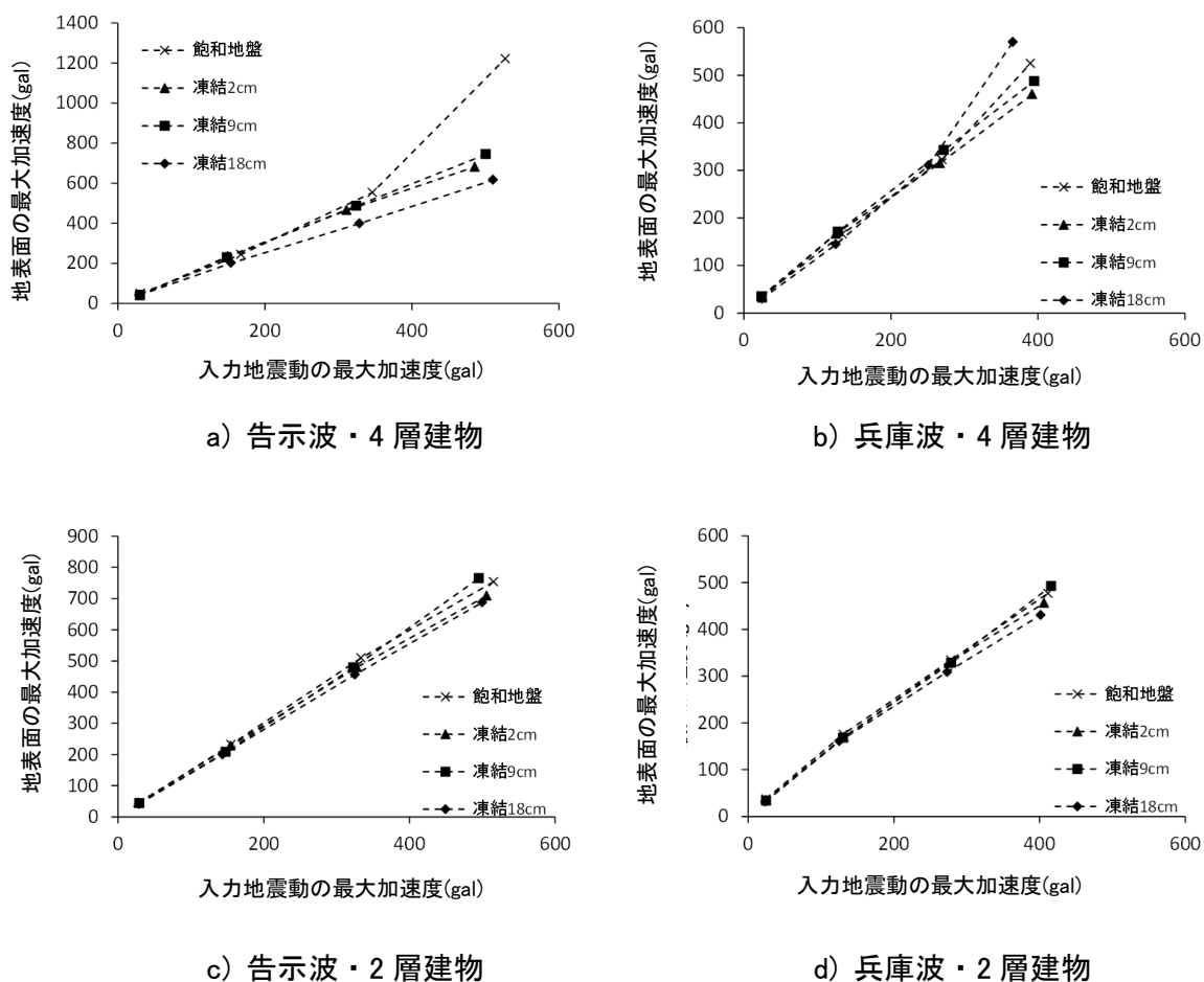
図 3.3.20 地表面の最大加速度の比較
