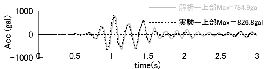
(b) 1.0 倍入力
