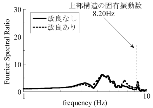
(f) 兵庫県南部地震波3.0倍加震
