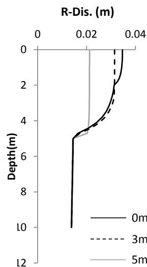
(c) 最大変位の深さ分布
