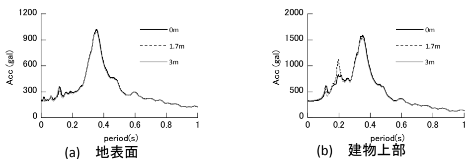
図 4.3.7 凍結深さによる地表面と建物上部の加速度応答スペクトルの比較 (告示乱数位相 0.2 倍・2 階建物)
