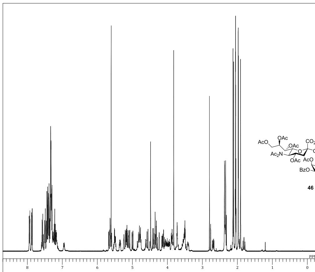
1 H NMR
