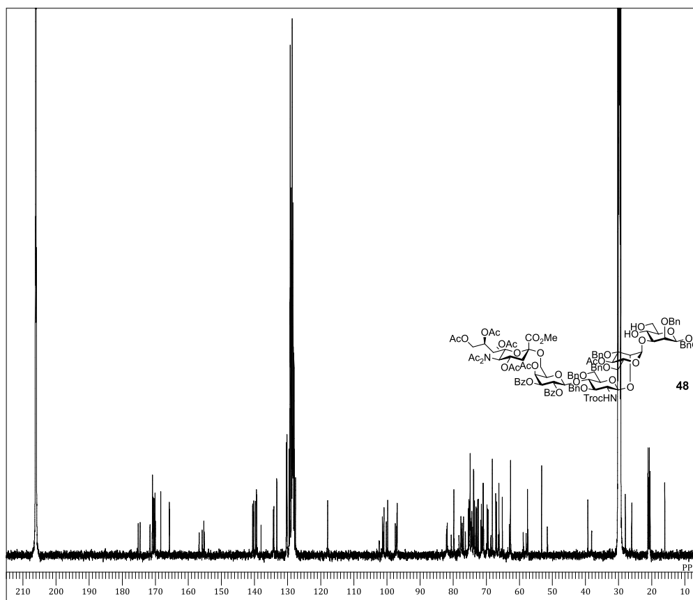
13 C NMR
