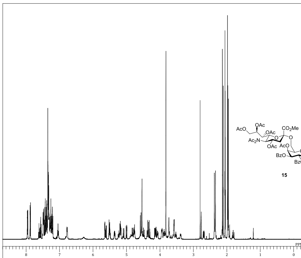
1 H NMR
