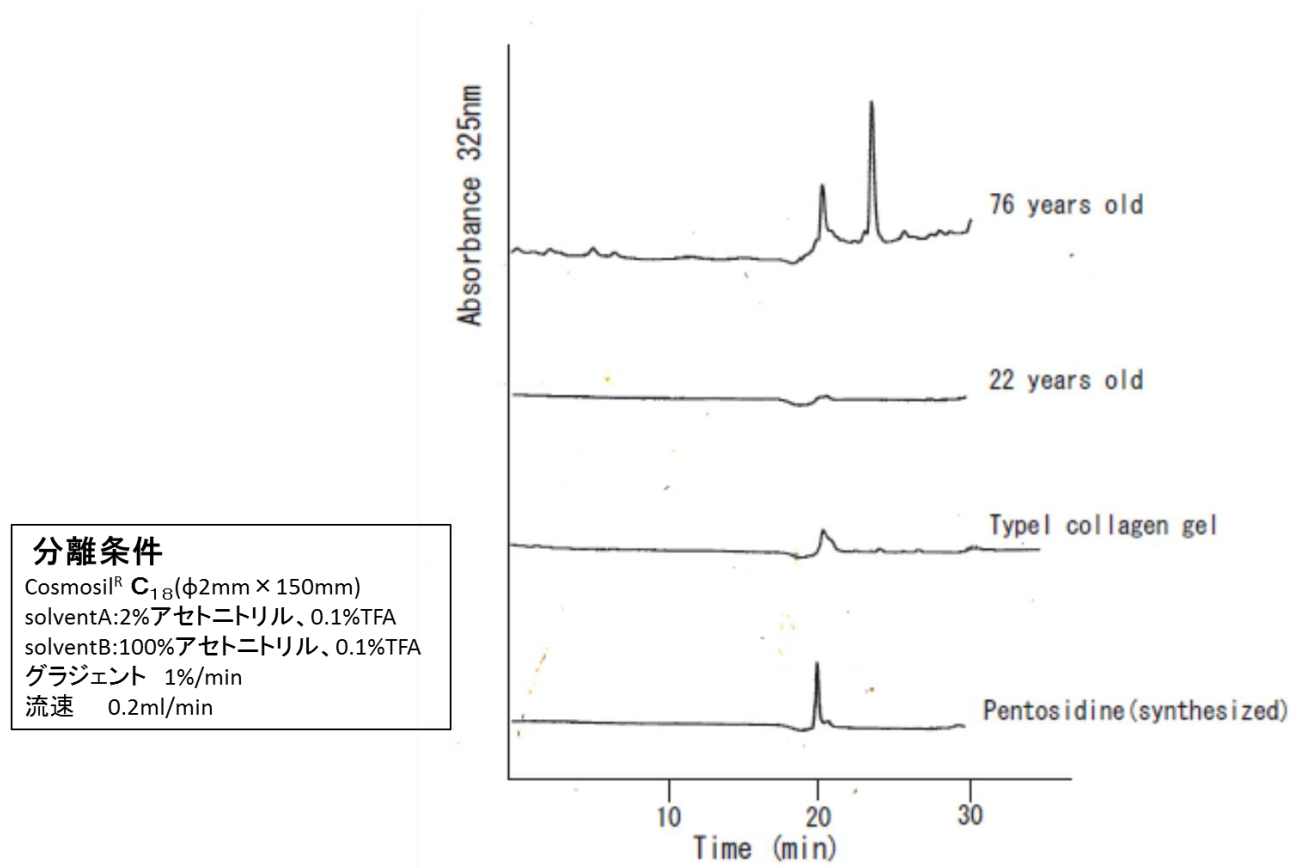
図 1 8 象牙質酸加水分解物の逆相カラムによるクロマトグラム
