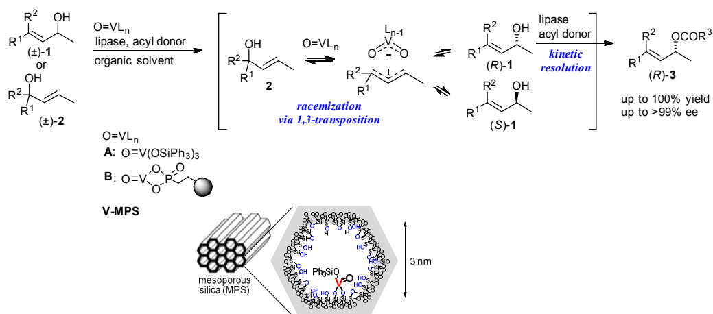
Scheme 1. リパーゼとオキソバナジウムを併用する動的光学分割(DKR)法。
