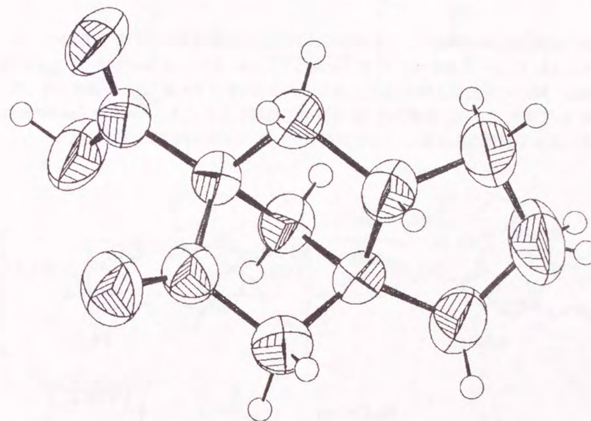
Figure 5.2 69 のORTEP図
