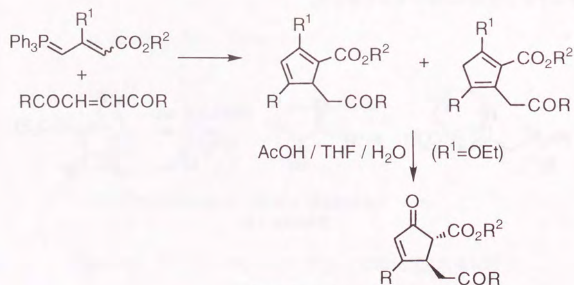
Scheme 1.4
