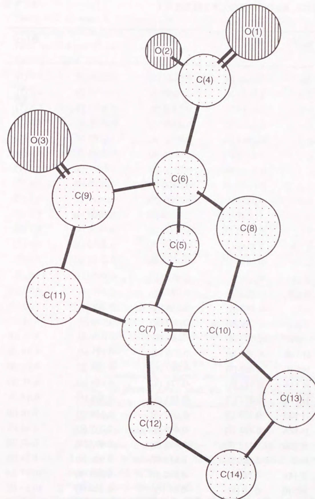
Figure 5.10 69 の結晶構造
