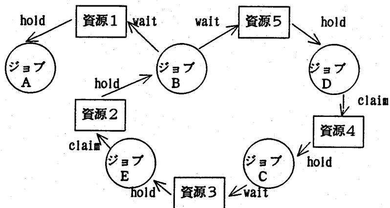
図 5.4 Hold-WaitとHold-Claimの混合グラフ
