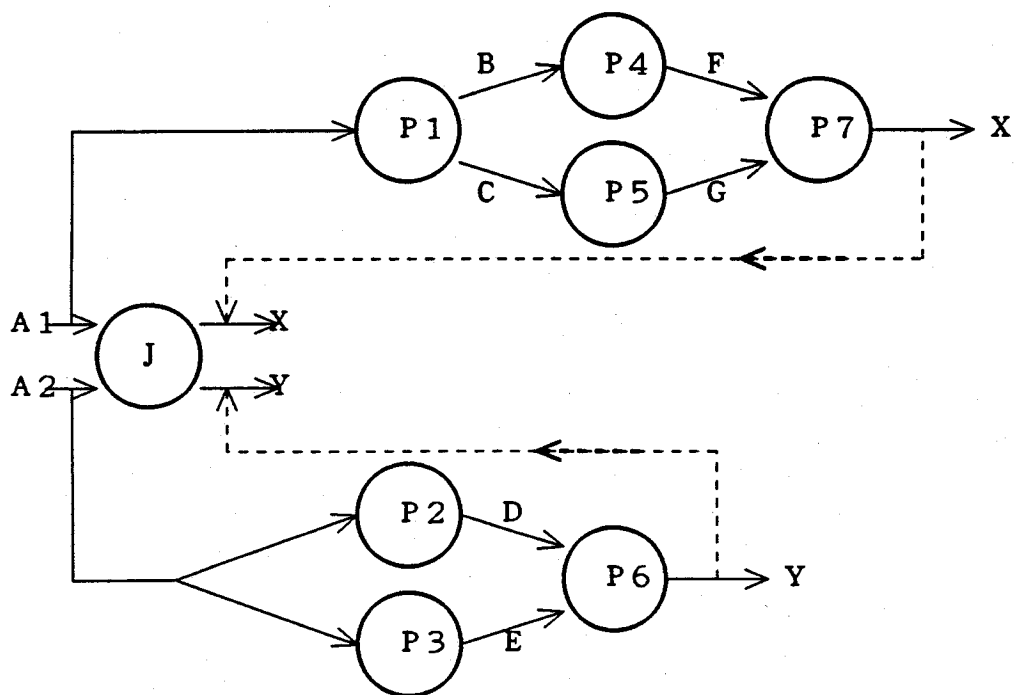
図3.1 プロセス列合成の例
