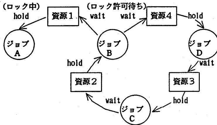
図 5.1 Hold-Wait グラフ
