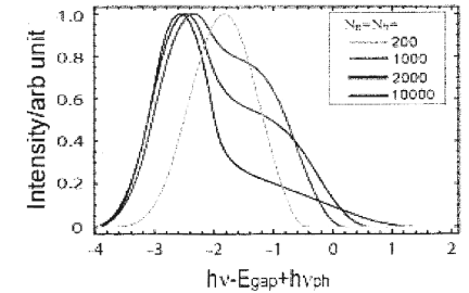
図 2. 発光スペクトルの液滴サイズ依存性
