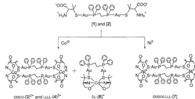
図 2 金(I)二核錯体配位子と Co III および Ni II イオンとの反応
