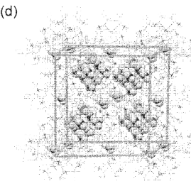
図 1 (a) Au 4 M III 2 六核錯体の合成、 (b) [3](ClO 4 ) 2 におけるカチオン六量体、 (c) アニオン 10 量体、および (d) カチオン-アニオン分離集積構造
