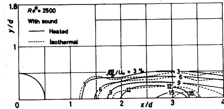
図6-8 周期的等変動速度 \sqrt{u_z'}/U_\infty 線図 ( Re^* = 2500 )
