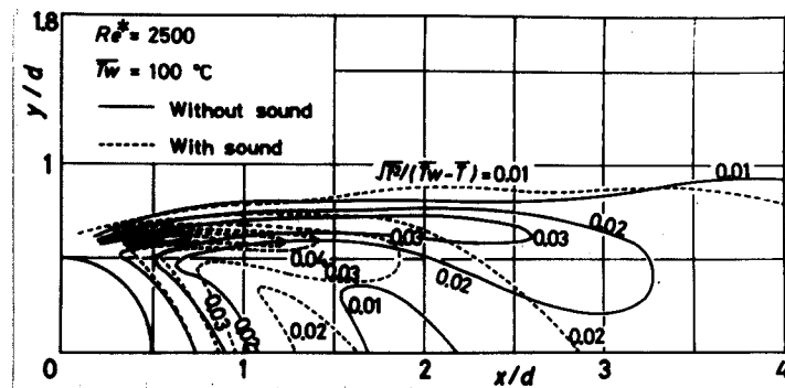
(b) 等変動温度 \sqrt{\bar{T}(T_w - T)} / (\bar{T}_w - \bar{T}) 線図
