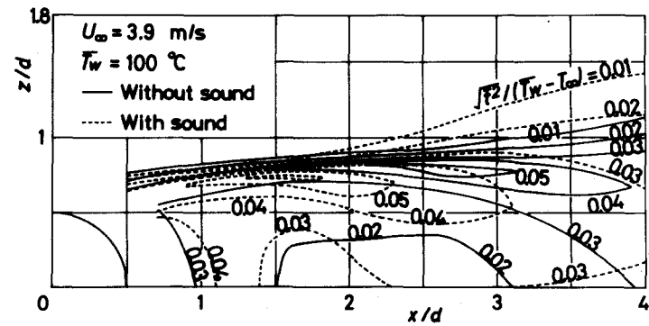
(b) 等変動温度 \sqrt{\theta^2} / (\bar{T}_w - T_{\infty}) 線図
