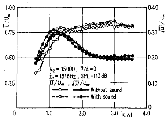
図3-10 円柱後流軸上のx方向 平均速度 \bar{U} ならびに変動 速度分布 ( Re = 15000 , f_a = 1918 Hz, SPL = 110 dB)
