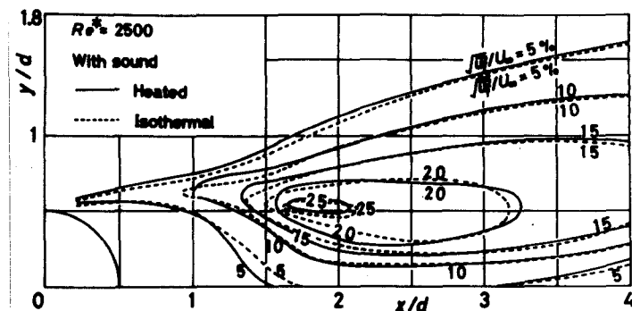
図6-7 周期的等変動速度 \sqrt{u'}/U_\infty 線図 ( Re^* = 2500 )
