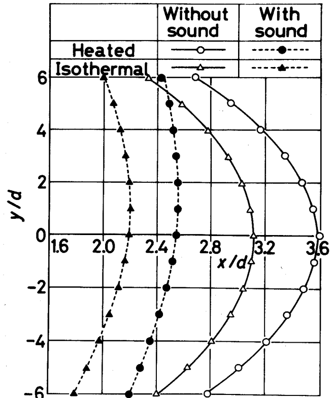
図5-12 最大乱れ位置 (x/d)_m におけるうず系形状 ( U_{\infty} = 3.9 \text{ m/s} )
