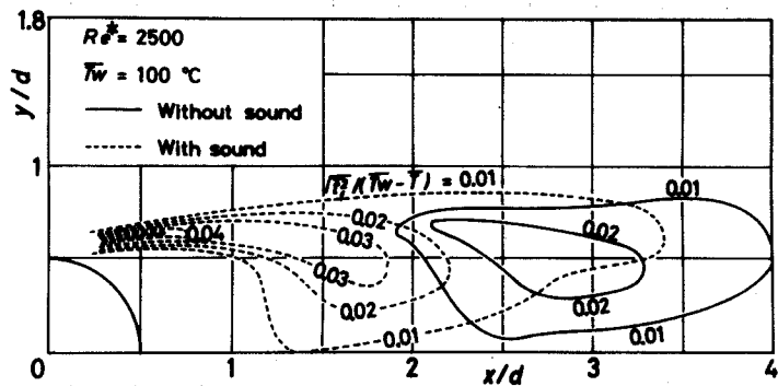
(c) 周期的等変動温度 \sqrt{\bar{T}(T_w - T)} / (\bar{T}_w - \bar{T}) 線図
