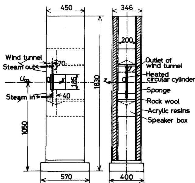
図5-1 実験装置
