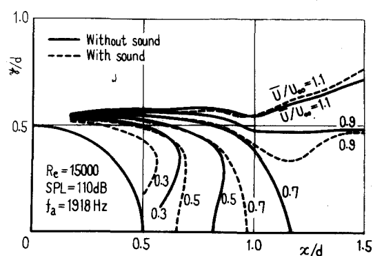
図3-11 等平均速度 \bar{U}/U_\infty 線図 ( Re = 15000 , f_a = 1918 Hz, SPL = 110 dB)
