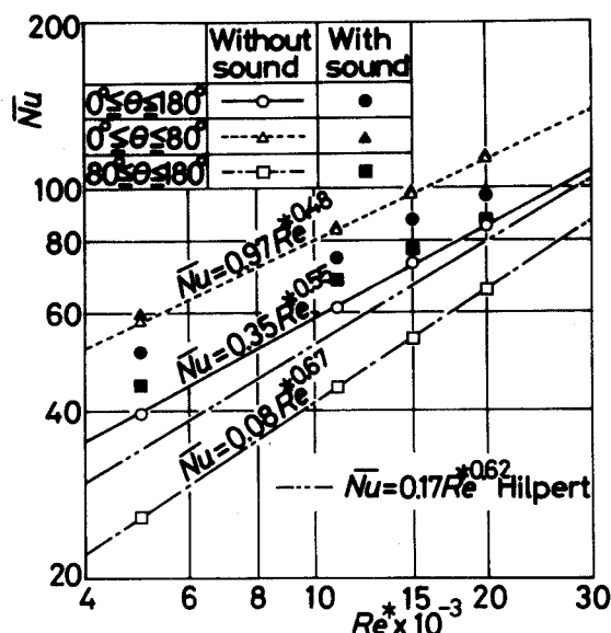
図5-7 平均熱伝達率
