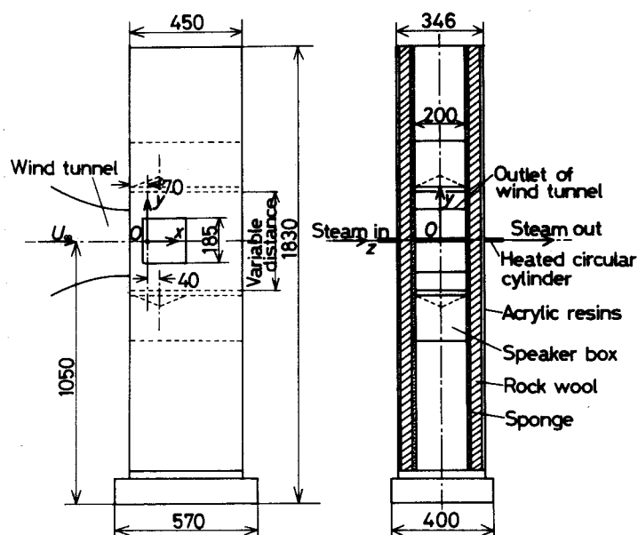
図6-1 実験装置
