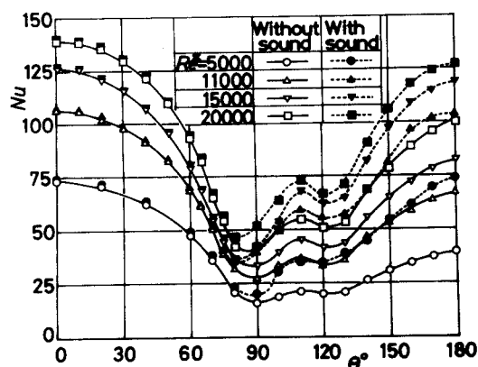
図5-6 局所熱伝達率分布
