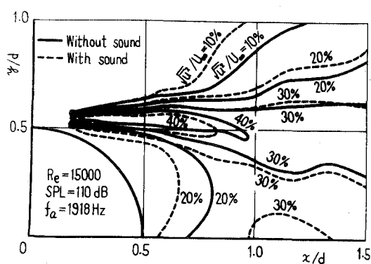
図3-12 等変動速度 \sqrt{\bar{u}^2}/U_\infty 線図 ( Re = 15000 , f_a = 1918 Hz, SPL = 110 dB)
