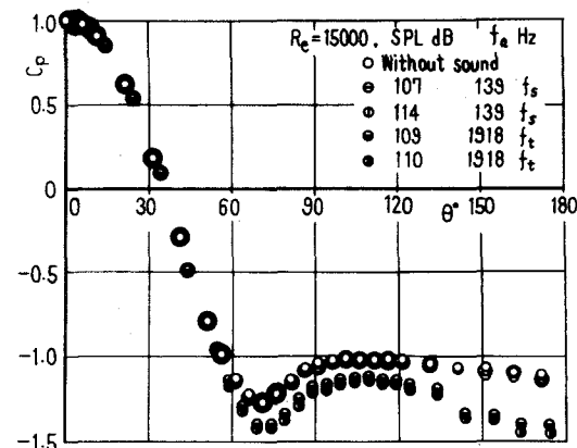
図3-8 円柱まわりの圧力分布 ( Re = 15000 )
