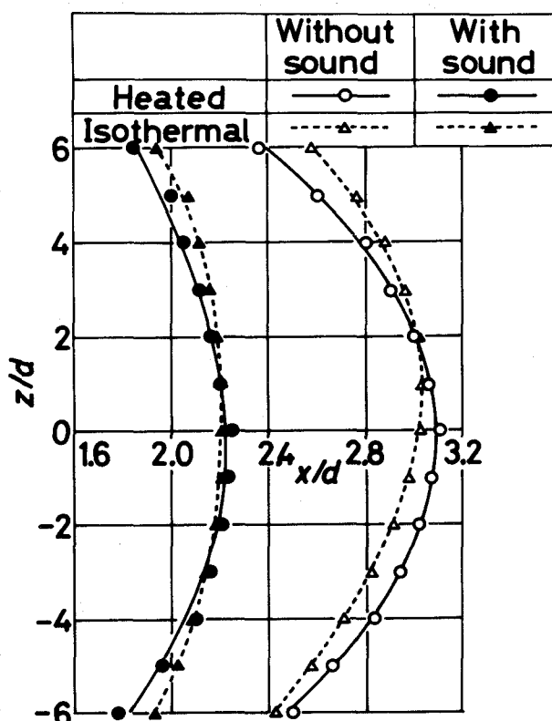
図6-11 最大乱れ位置 ( x/d ) m におけるうず系形状 ( Re^* = 2500 )
