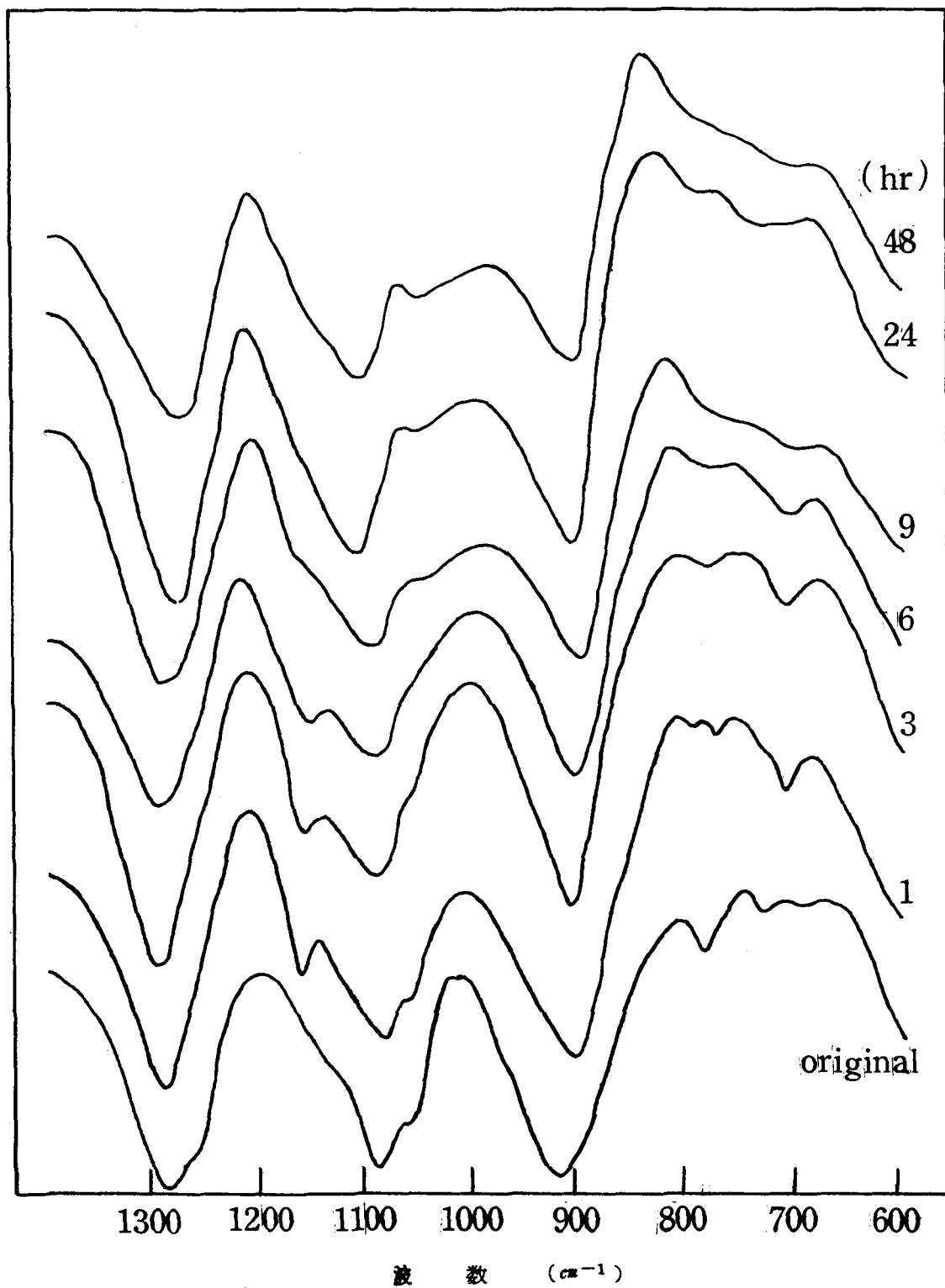
図4.6 \text{LiPO}_3\text{I} の摩砕によるIRSの変化
