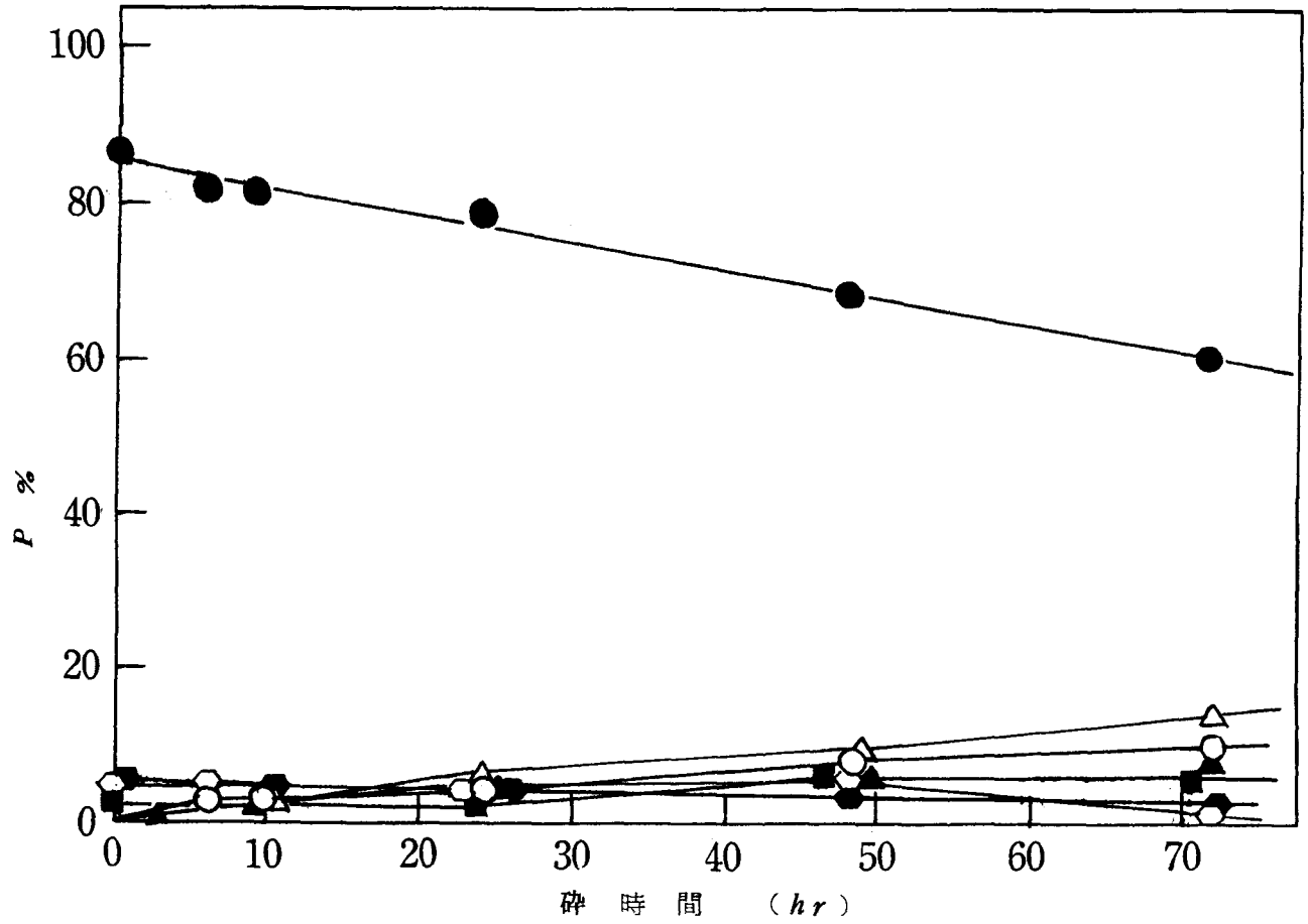
図 39 Na_2O_3G の摩砕による分子種の変化
