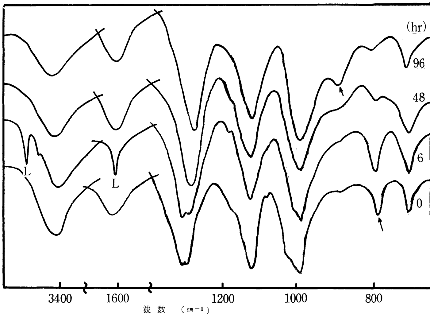
図24 \text{Na}_4\text{P}_4\text{O}_{12} の摩砕による IRS の変化
