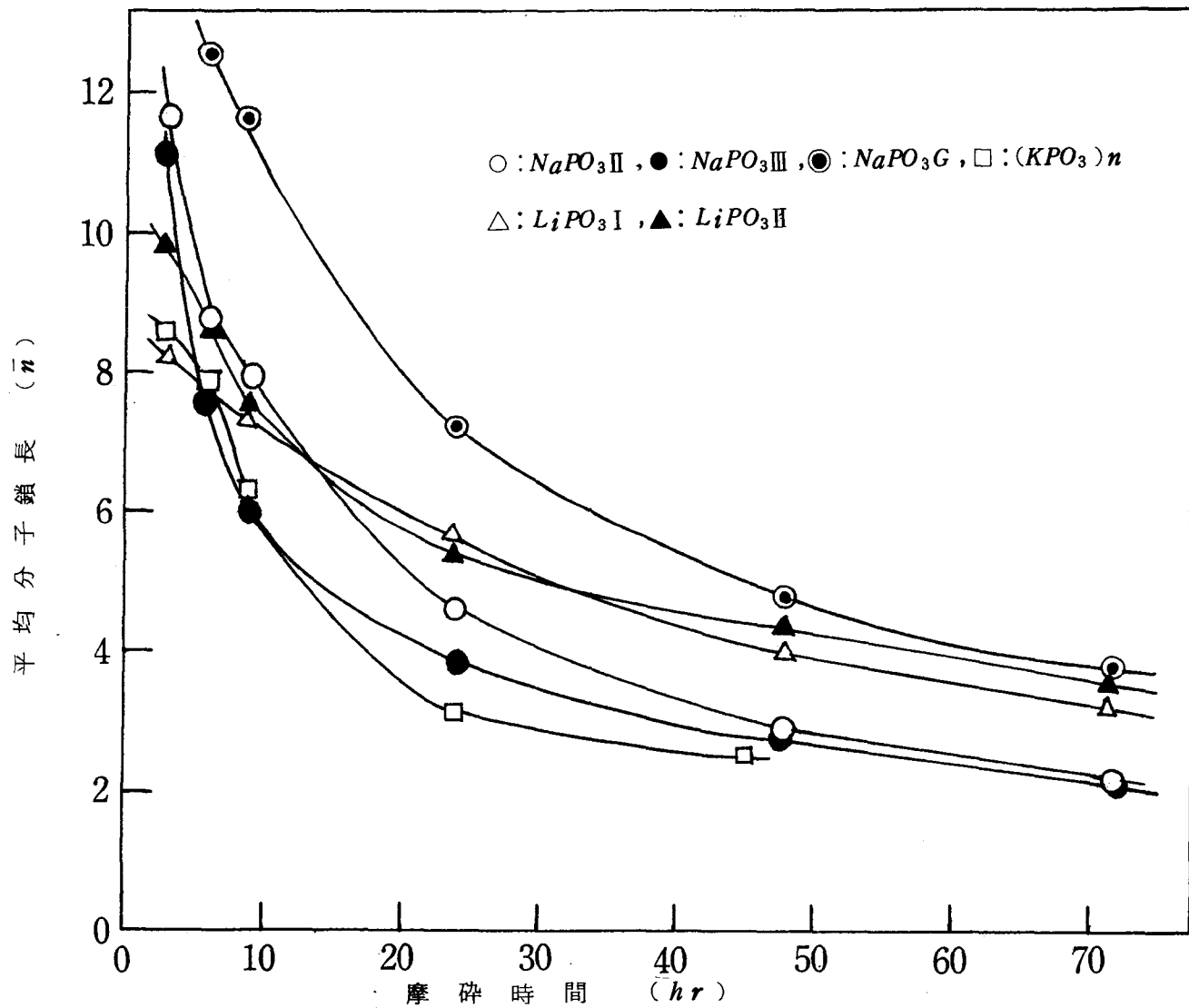
図50 長鎖状ポリリン酸塩の摩砕による可溶性成分の平均分子鎖長( \bar{n} )の変化
