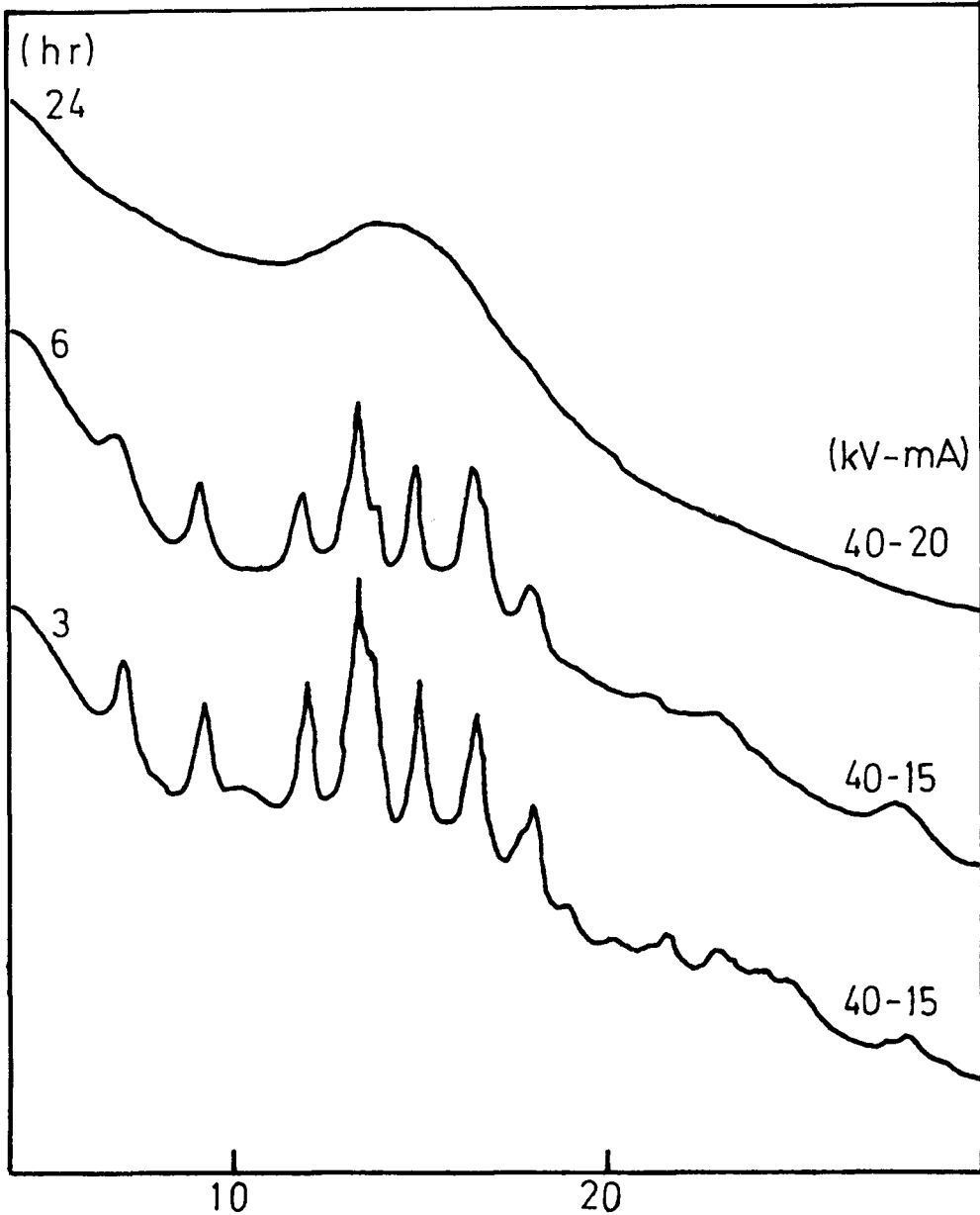
図6 X線回折図の変化 ③ 湿度10%
