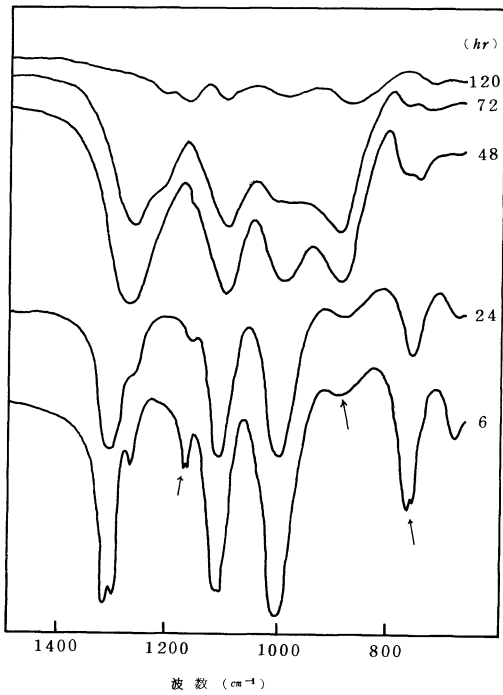
図9 I R S の変化 ②湿度30%
