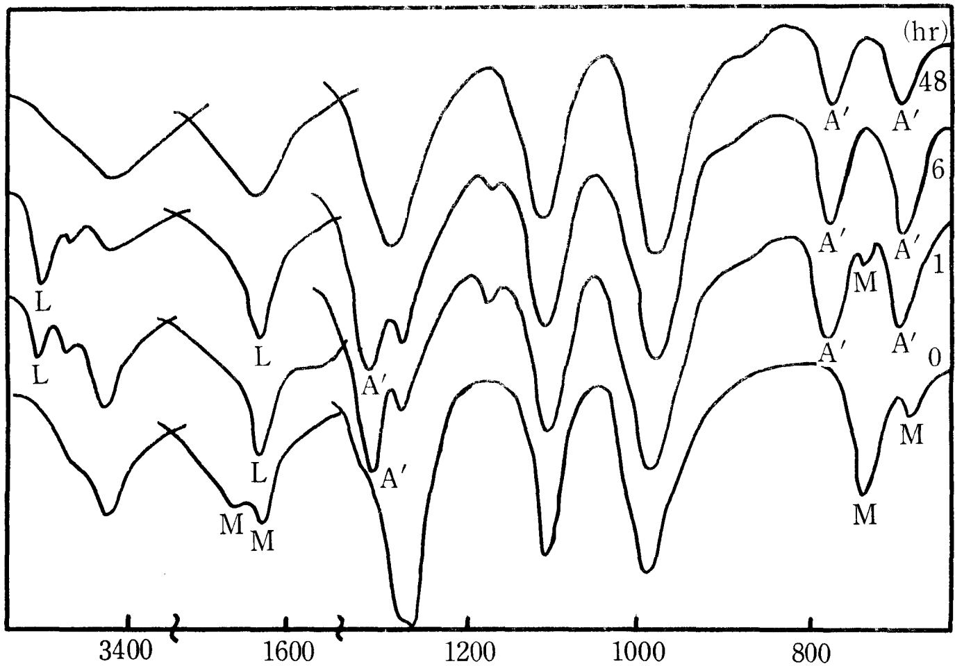
波 数 ( \text{cm}^{-1} ) 図 29 \text{Na}_4\text{P}_4\text{O}_{12} \cdot 4\text{H}_2\text{O} (M-form) の摩砕による IRS の変化 右側の数字は摩砕時間を示す。L: loose water
