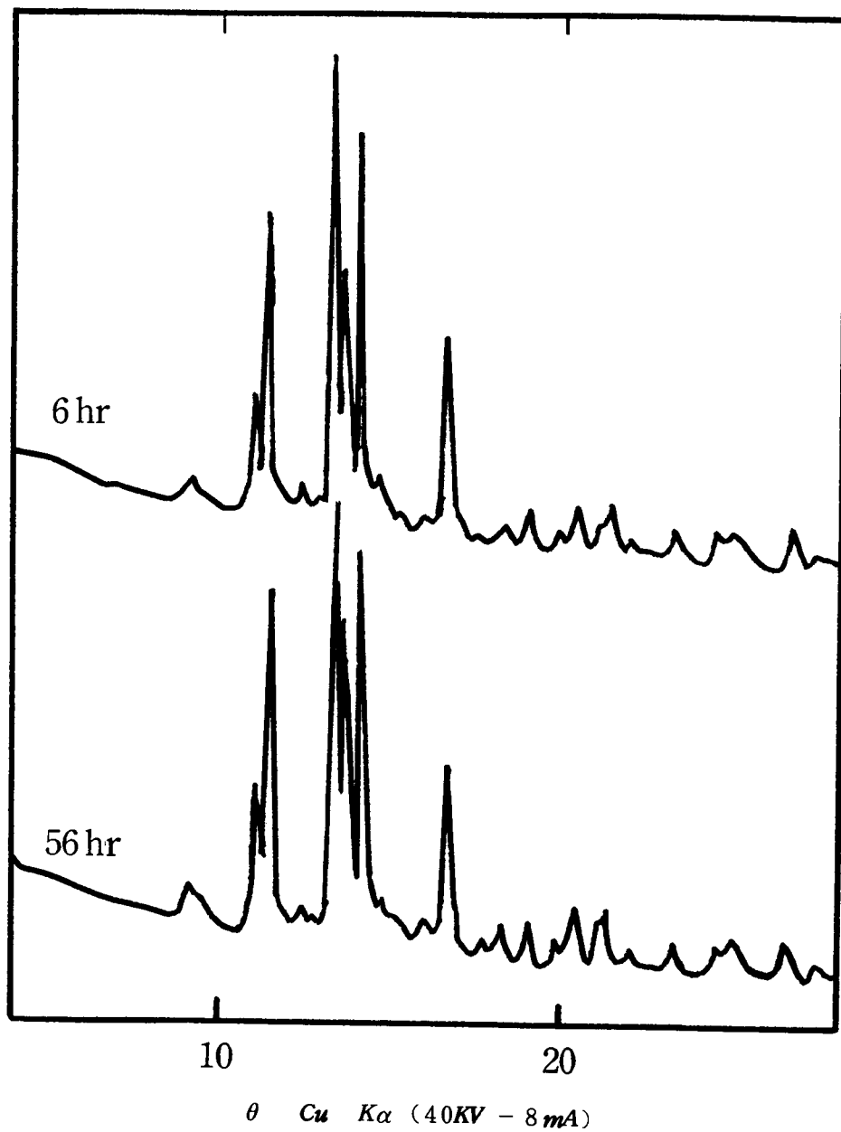
図 5 1 低湿度下で摩砕した \text{NaH}_2\text{PO}_4 の X 線回折図
