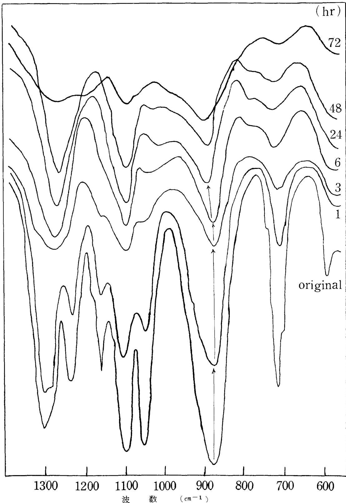
図 35 \text{NaPO}_3 III の摩砕による IRS の変化
