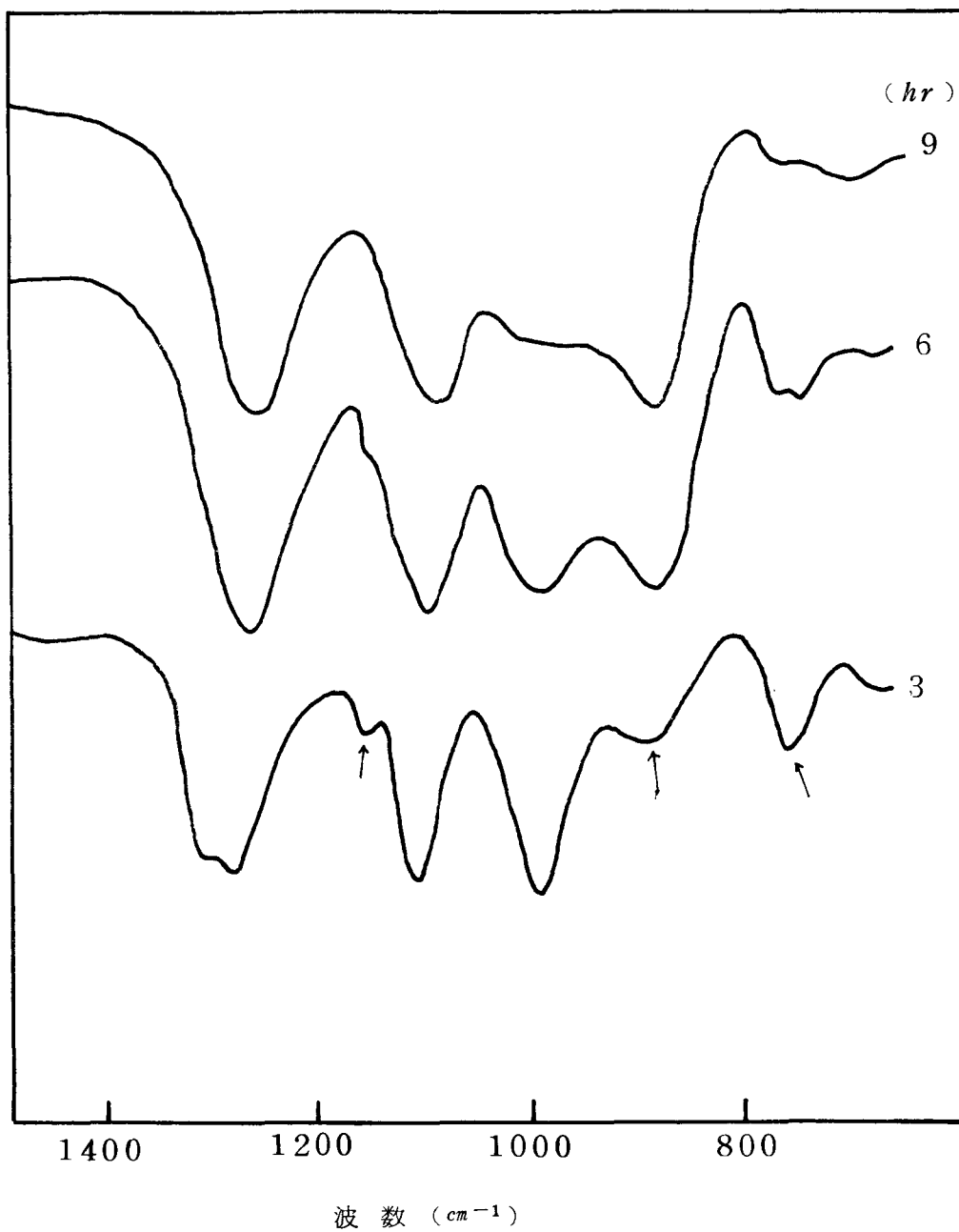
図11 I R S の変化 ④湿度5%以下
