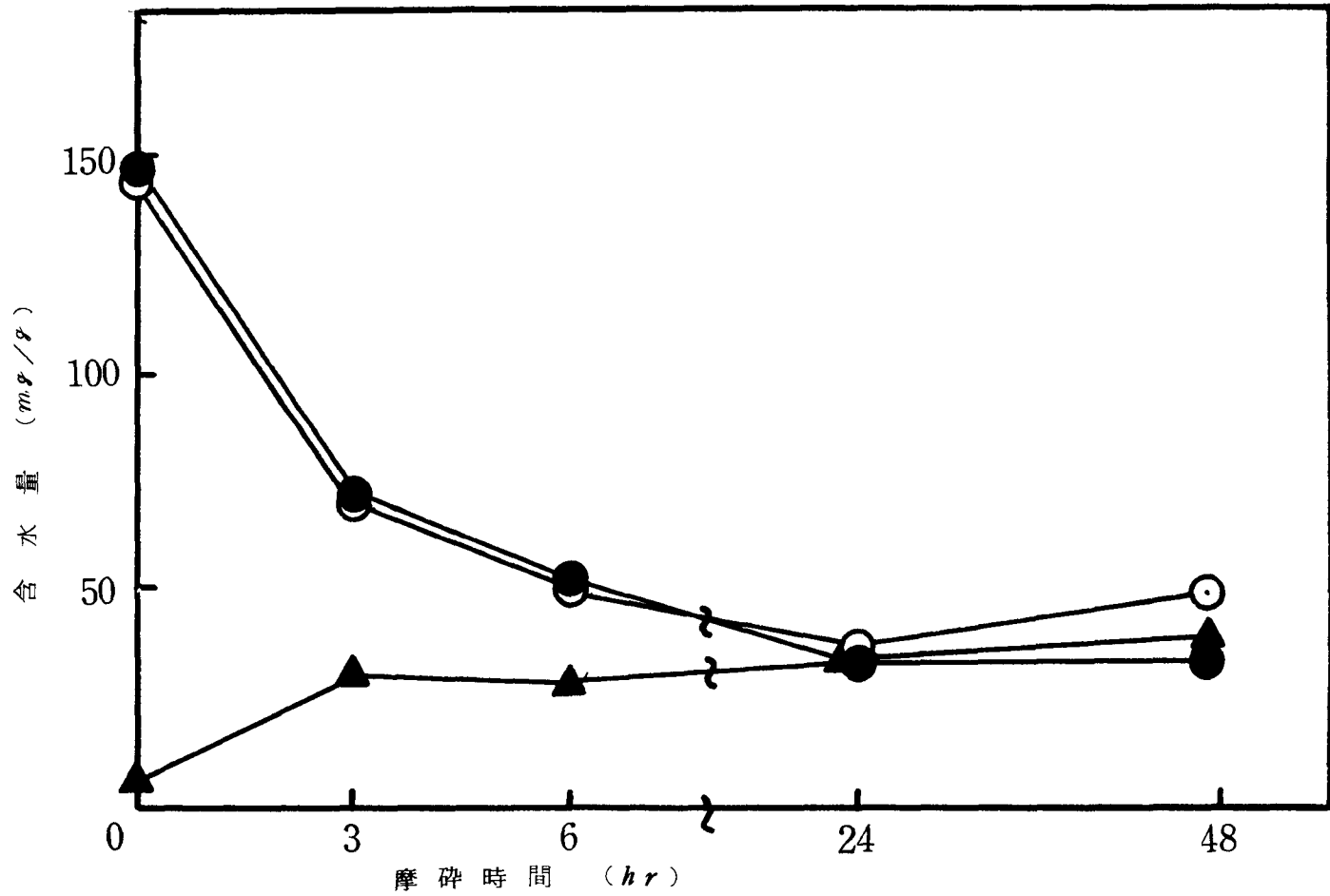
図30 磨碎による含水量の変化
