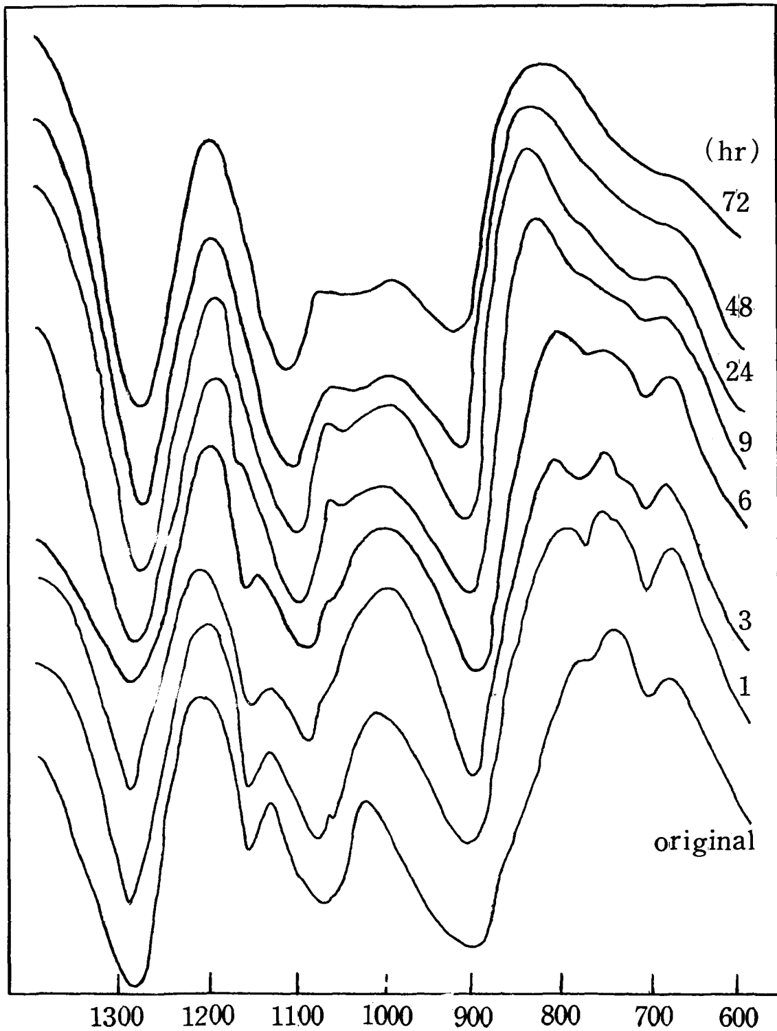
図 47 \text{LiPO}_3 \text{ II} の摩砕による IRS の変化
