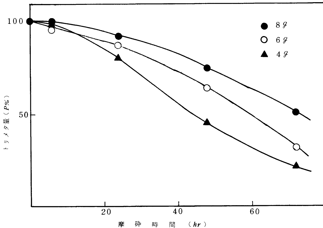
図3 摩碎効果におよぼす試料量の影響
