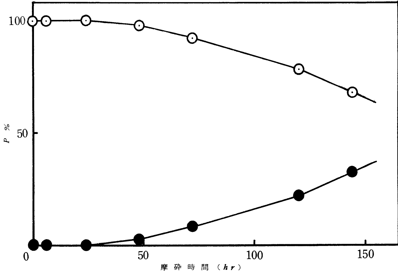
図25 Na_4P_4O_{12} の摩碎によるテトラメタリン酸塩の減少と鎖状リン酸塩の増大
