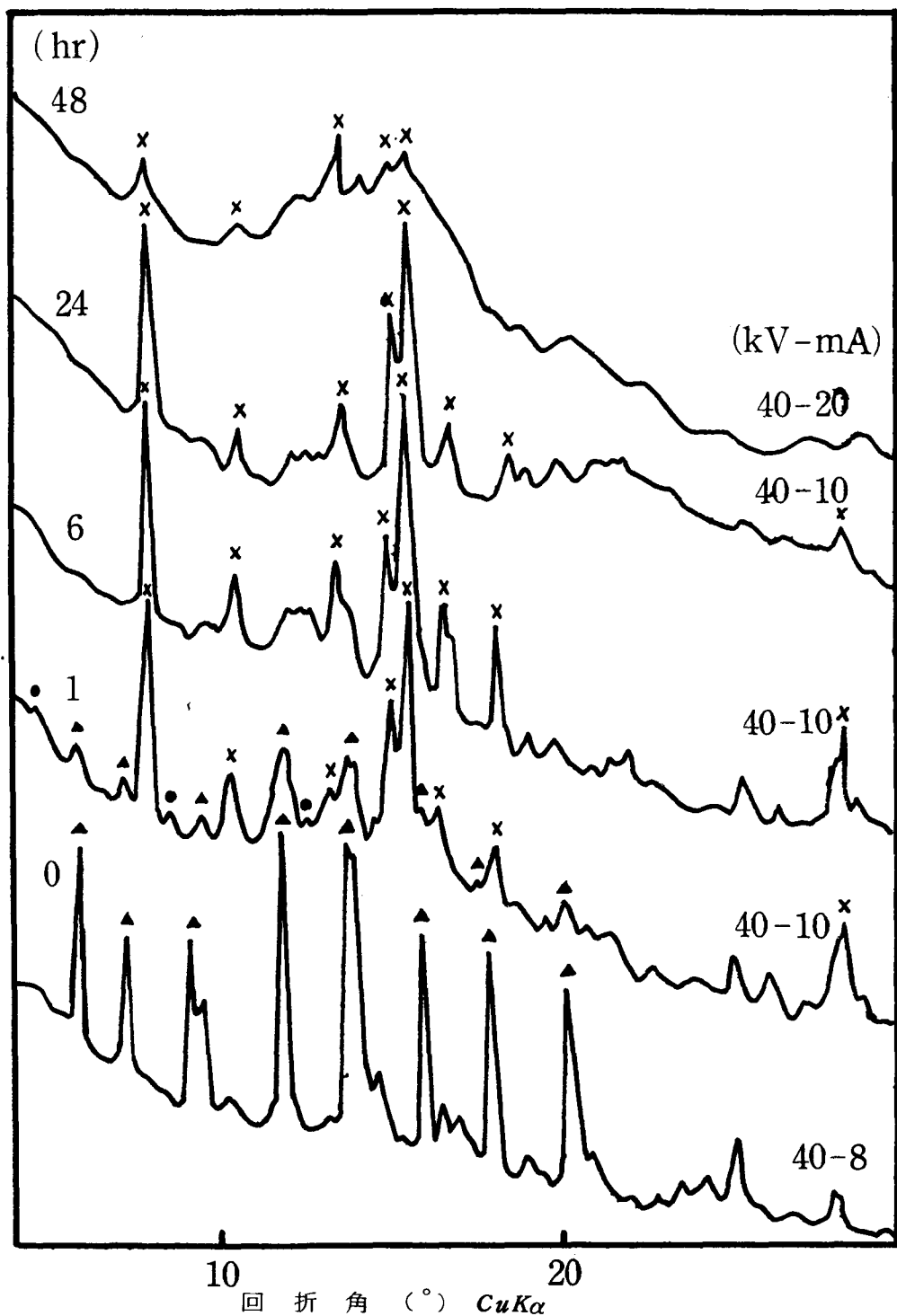
図28 \text{Na}_4\text{P}_4\text{O}_{12} \cdot 4\text{H}_2\text{O} (M-form) の摩砕による X線回折図の変化 \Delta : M-form, \bullet : T-form, \times : A の主要回折線を示す。
