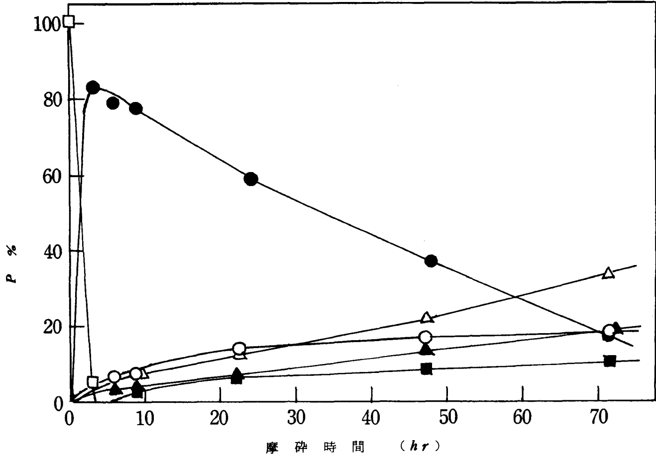
図 38 NaPO_3 III の摩碎による分子種の変化
