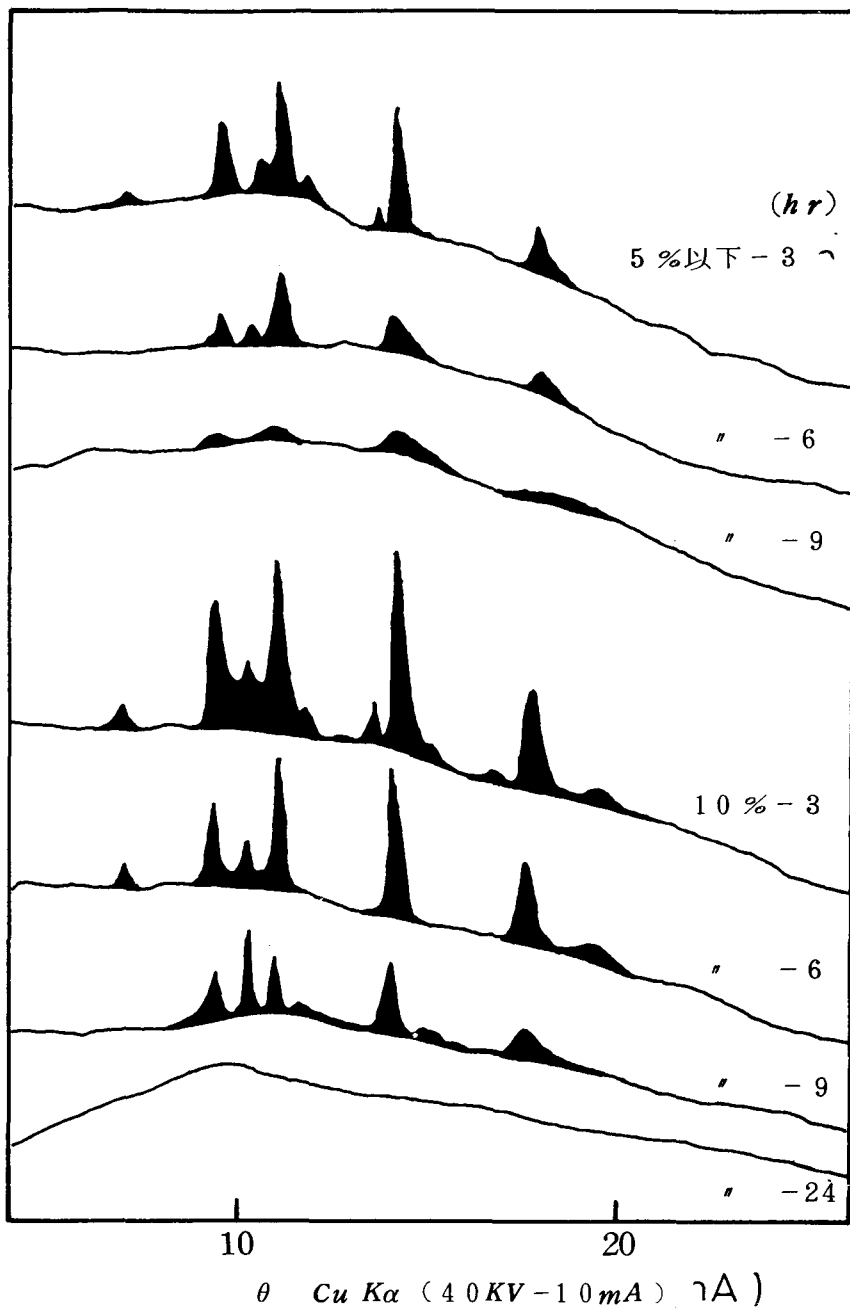
図56 摩砕した Li_2H_2P_2O_7 の X線回折図
