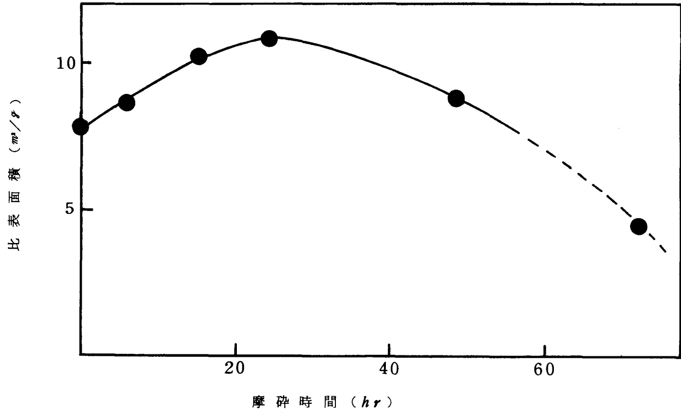
図 22 摩砕による比表面積の変化
