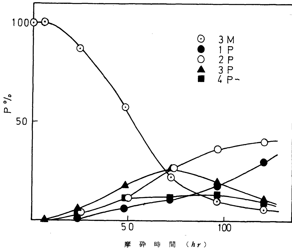
図14 分子種の変化 ②湿度30%
