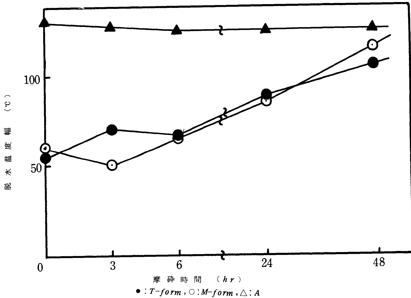
図 31 摩砕による脱水温度幅の変化
