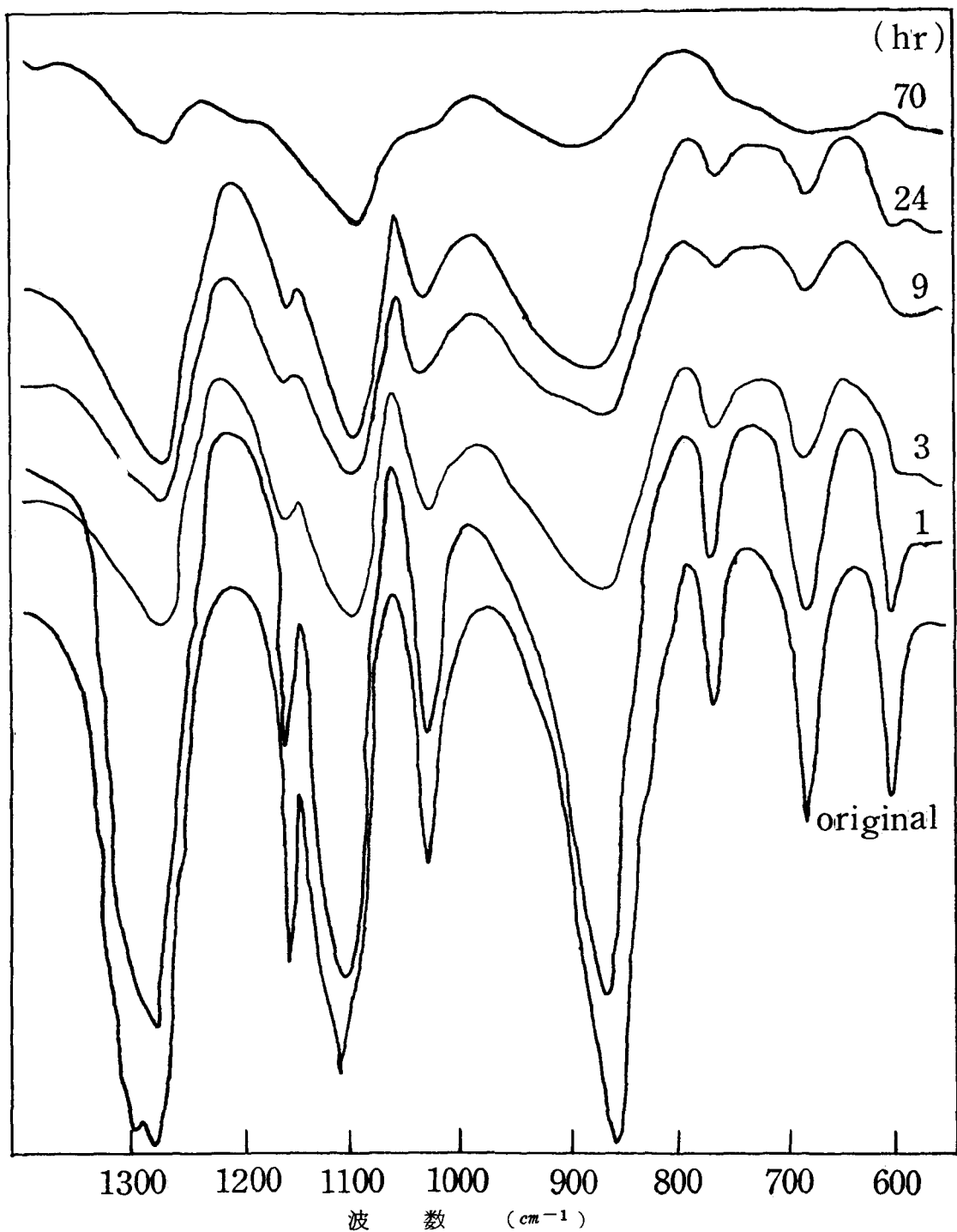
図 42 (KPO_3) n の摩砕による IRS の変化
