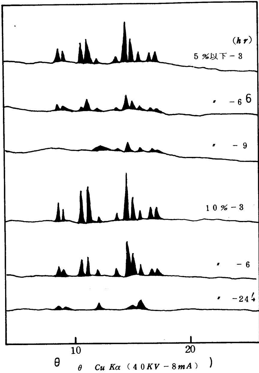
図 57 摩砕した K_2H_2P_2O_7 の X 線回折図
