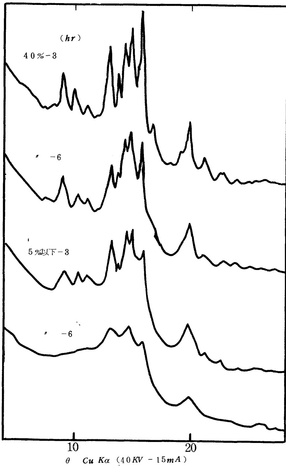
図53 種々の条件下における Na_3H_2P_3O_{10} の摩砕変化
