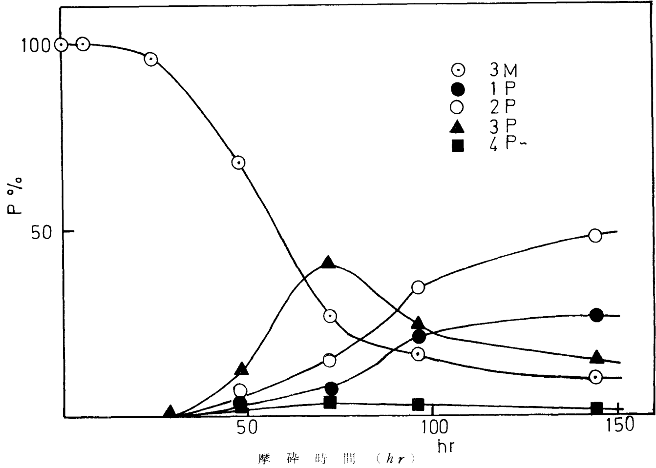
図13 分子種の変化 ①湿度60%
