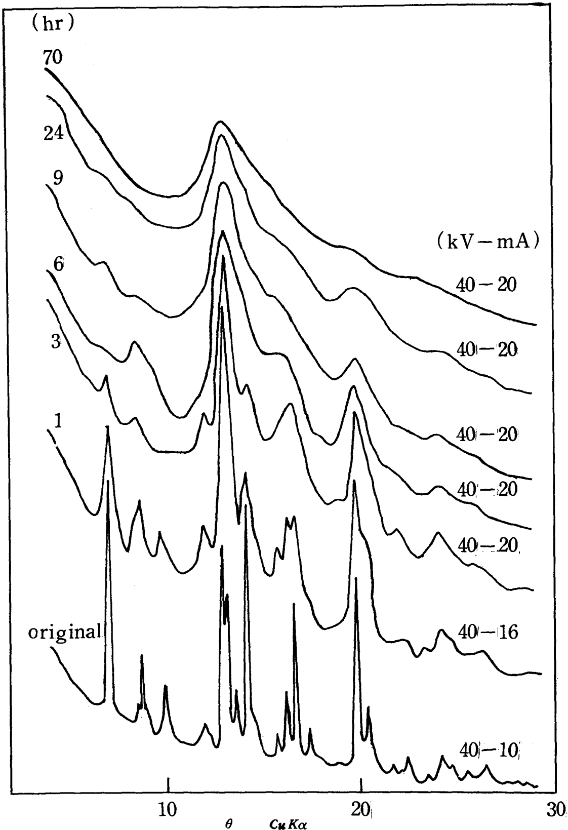
図 40 (KPO_3)_n の摩砕による X 線回折図の変化
