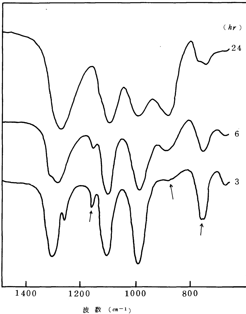
図10 I R S の変化 ③湿度10%
