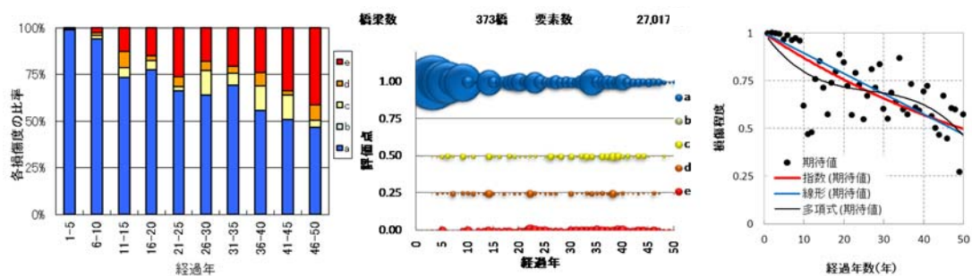
図-4.3.1 (4) 散布データと期待値の回帰式（鋼鈑桁主桁防食機能の劣化（C 塗装系））
