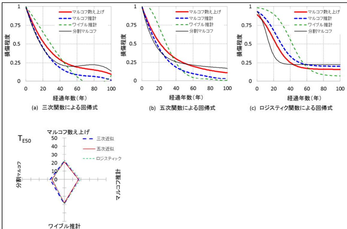
図-4.3.6(9) 損傷程度の評価の期待値の劣化曲線 (コンクリートのひびわれ (下部工・橋脚))
