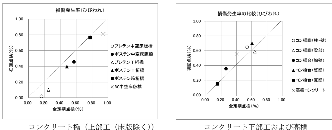
図-3.5.11 初回点検と2回目以降の定期点検の損傷発生率の比較（コンクリートのひびわれ）
