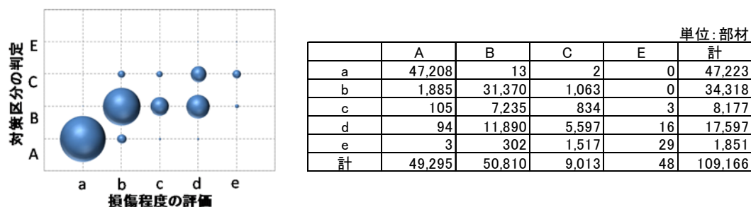
図-3.5.14 「損傷程度の評価」と「対策区分の判定」の比較（鋼橋主桁（鈹桁・腐食））
