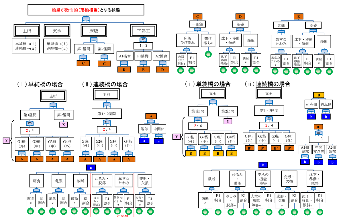
図-4.4.26 FT 図 (RC 床版を有する 4 主鉄桁橋)
