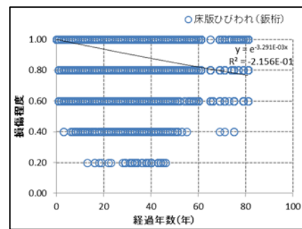
(b) 鋼桁
