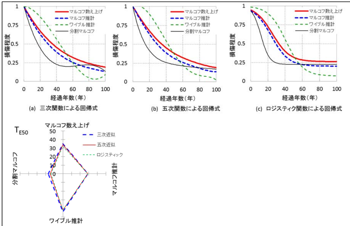
図-4.3.6(8) 損傷程度の評価の期待値の劣化曲線 (コンクリートのひびわれ (下部工・橋台))
