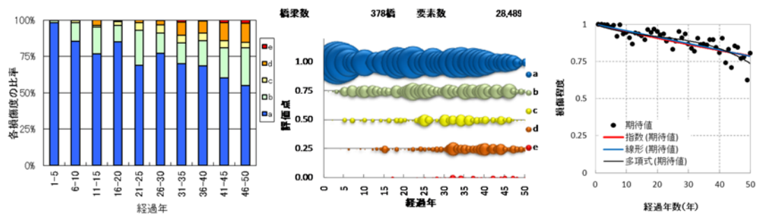
図-4.3.1 (2) 散布データと期待値の回帰式（鋼鈑桁主桁腐食（C 塗装系））
