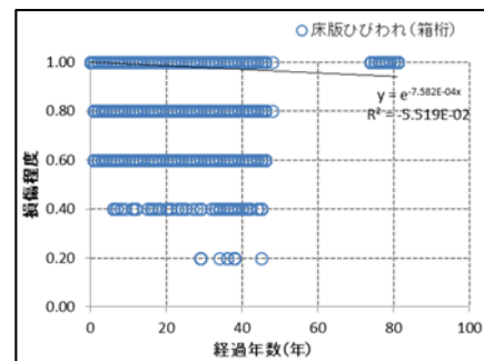
(f) 箱桁
