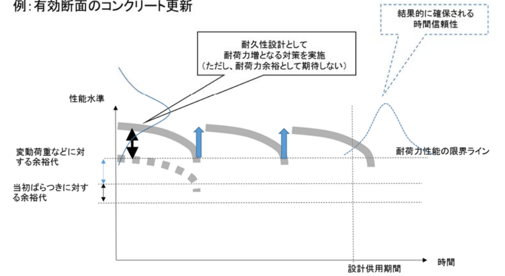
図-4.5.2 劣化の特徴から考えられる設計における耐久性確保戦略（パターン B）
