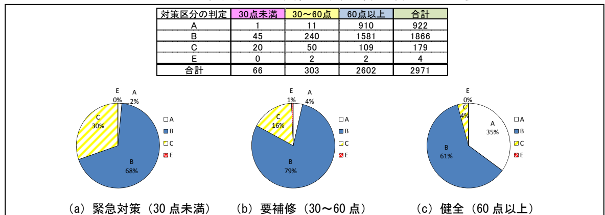
図-5.3.5 走行安全性の指標と対策区分の判定との比較
