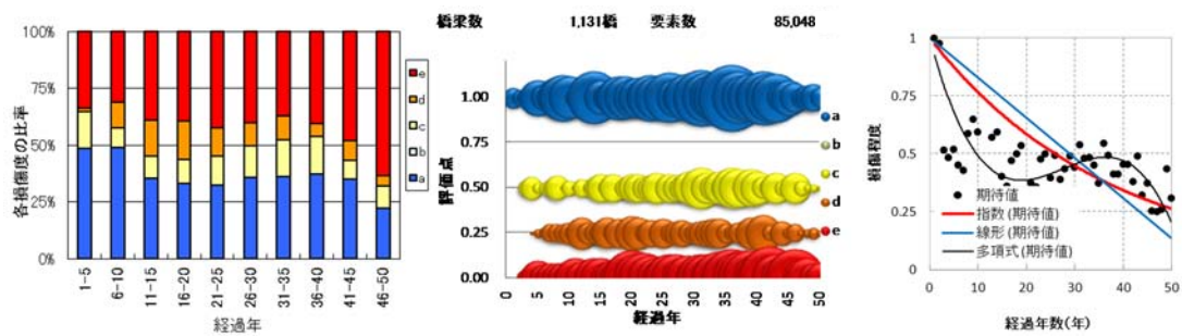
図-4.3.1 (3) 散布データと期待値の回帰式（鋼鈑桁主桁防食機能の劣化（A,B 塗装系））
