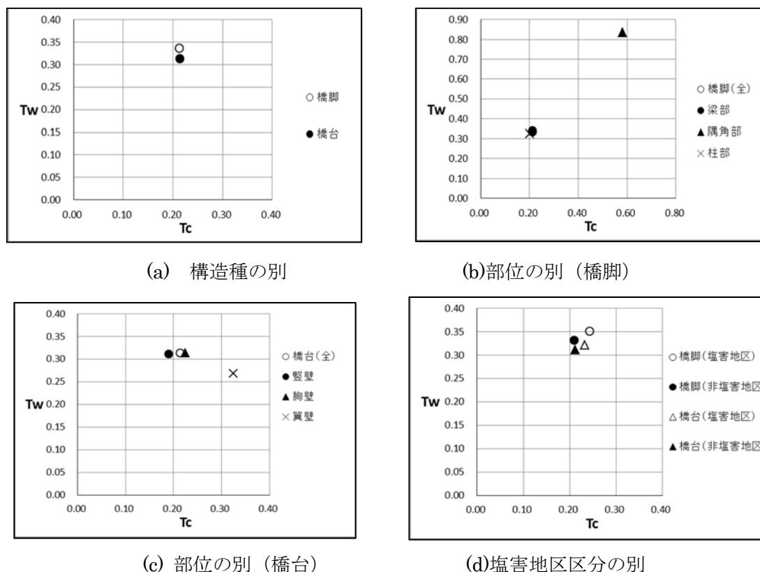
図-4.4.9 遷移確率行列からの劣化傾向 (コンクリート下部工のひびわれ)
