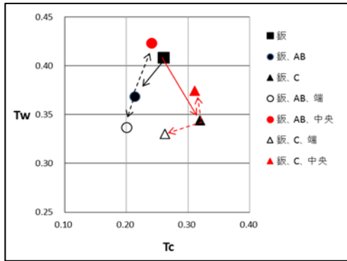
(a) 鋼主桁の腐食（鋼桁）
