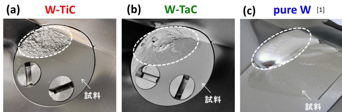
図 7.3 溶融実験後の試料の表面凝固層 (a) W-TiC 試料、(b) W-TaC 試料、(c) pure W ([1]から抜粋)
