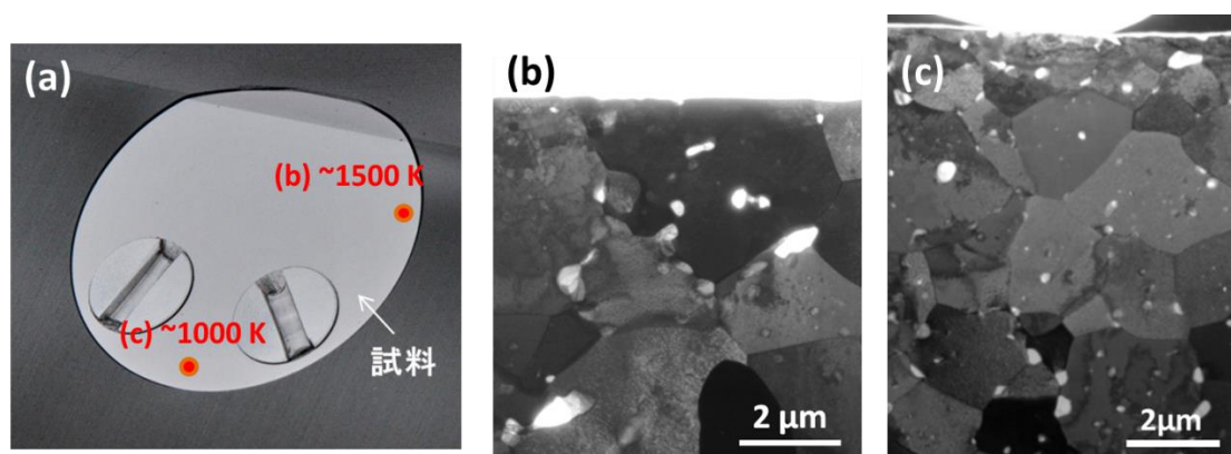
図 7.8 損耗実験後の W-TiC 試料の(a) 表面状態、 表面近傍の微細構造 (b) \sim 1500 K および(c) \sim 1000 K
