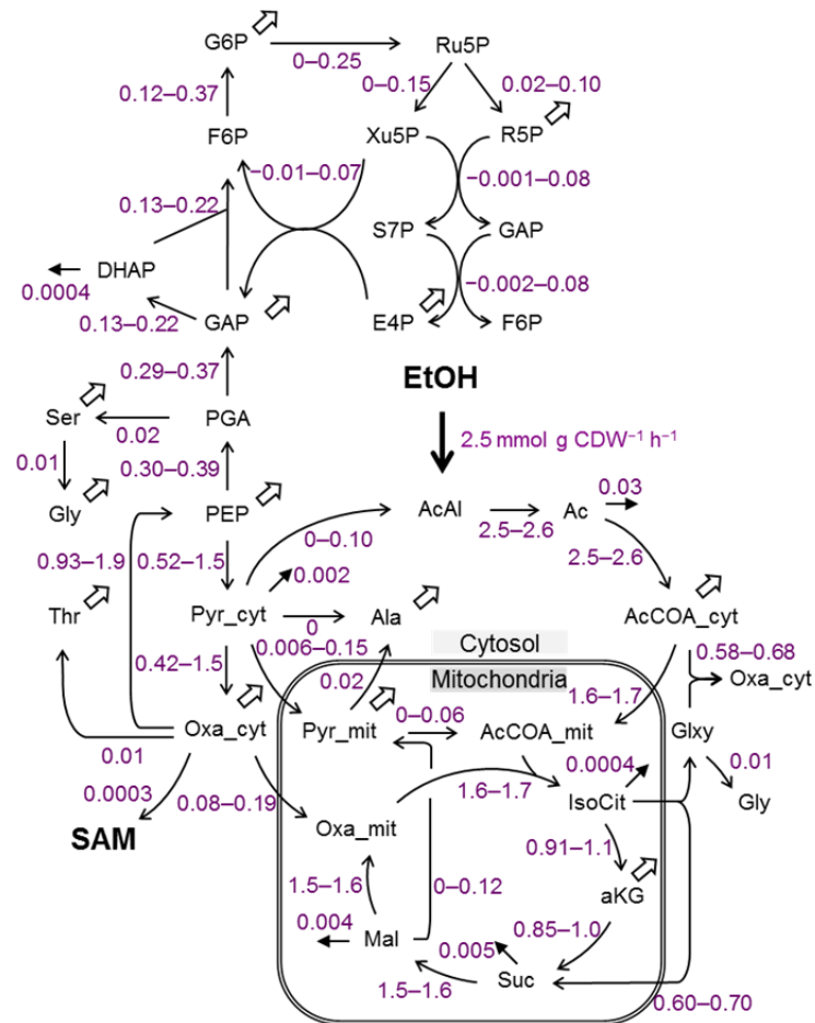
Fig. 3-2 清酒酵母協会 6 号の代謝フラックス分布 (希釈率 0.06 h -1 ) (続き)
