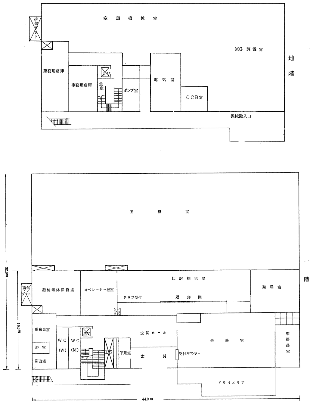
図2. 大型計算機センター建物平面図
