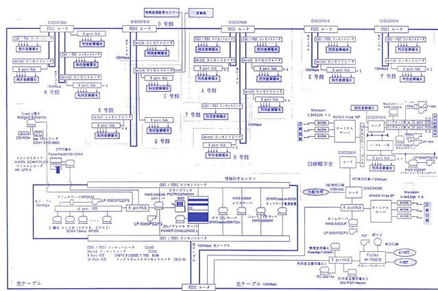
大阪電気通信大学のネットワークシステム構成図
