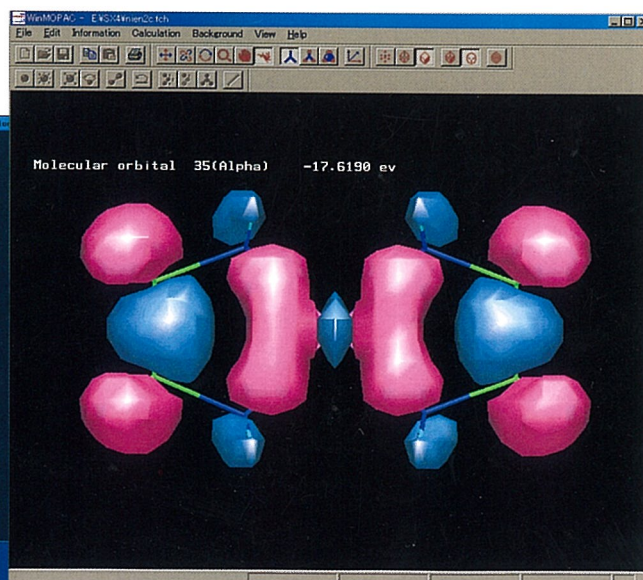
Win MOPAC ® による分子軌道の等値曲面
