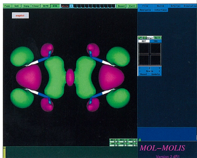
Mol Molis ® による [Ni(en)2]2+ の 35 番 MO の等値曲面
